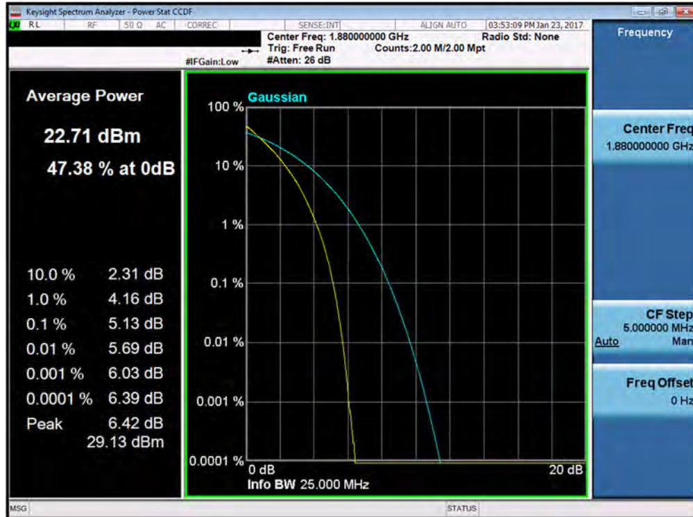
Plot 7-153. PAR Plot (Band 2 – 20.0MHz QPSK – RB Size 100)
