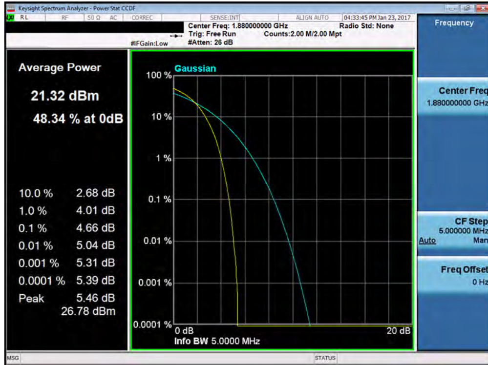
Plot 7-147. PAR Plot (Band 2 – 5.0MHz QPSK – RB Size 25)
