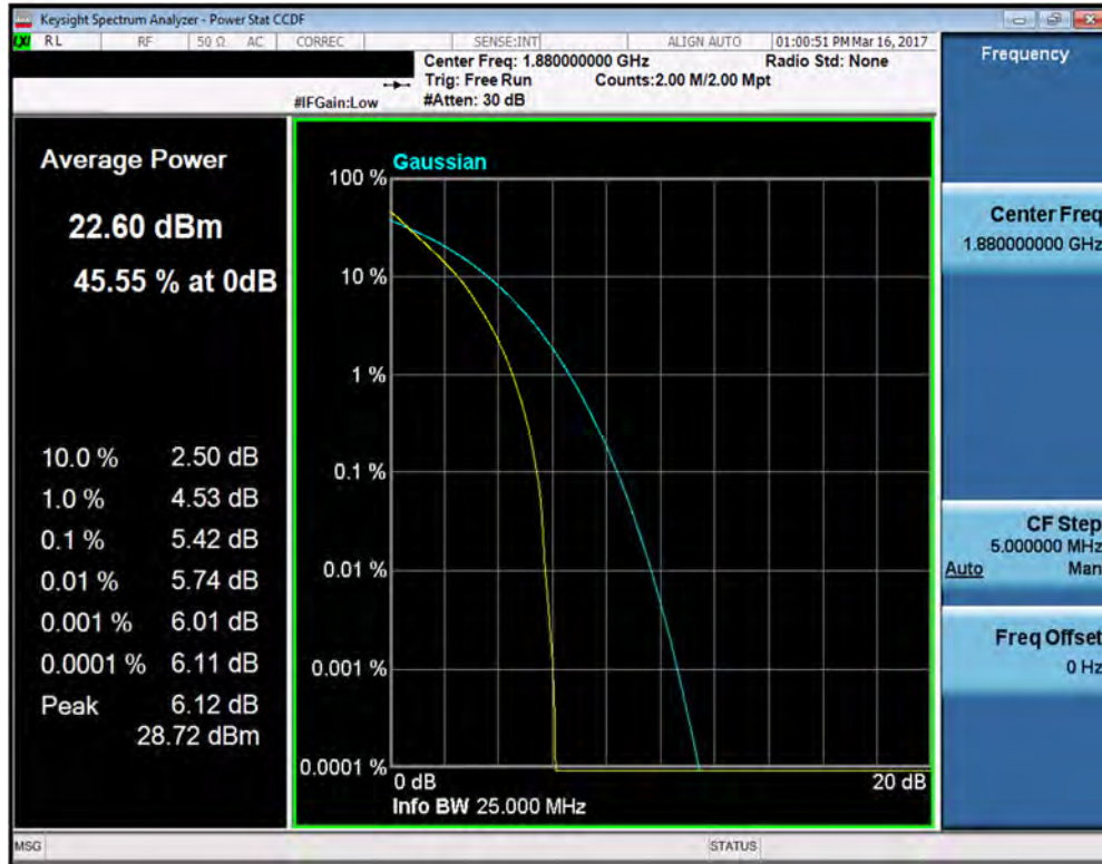
Plot 7-151. PAR Plot (Band 2 – 15.0MHz QPSK – RB Size 75)
