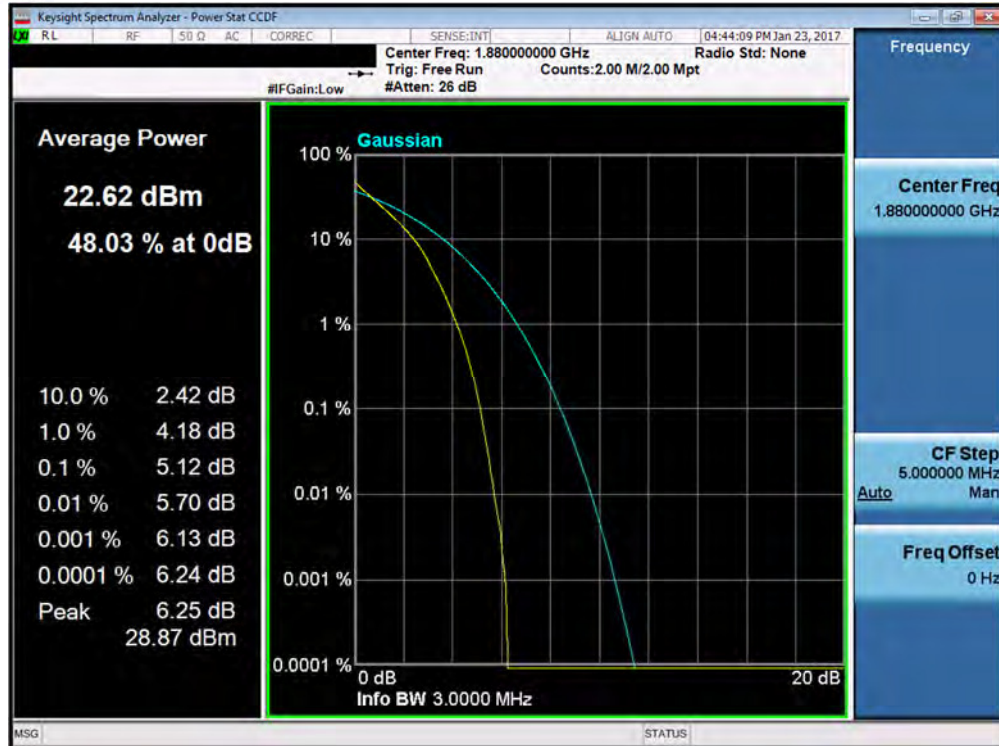
Plot 7-145. PAR Plot (Band 2 – 3.0MHz QPSK – RB Size 15)
