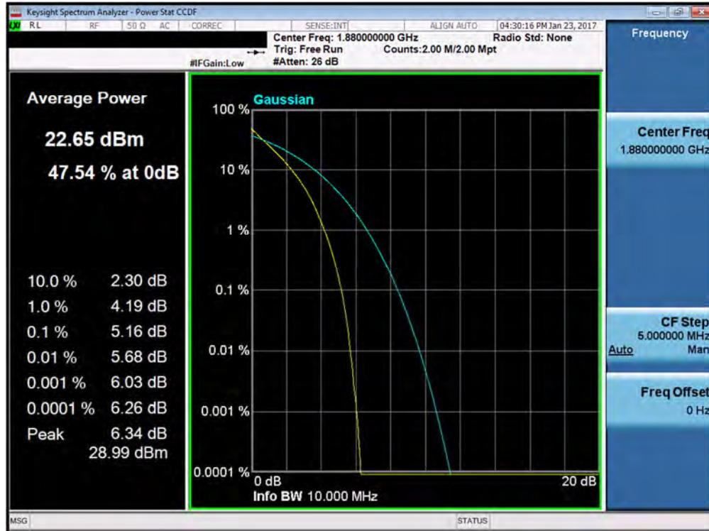
Plot 7-149. PAR Plot (Band 2 – 10.0MHz QPSK – RB Size 50)
