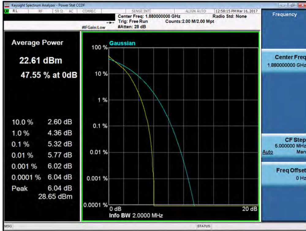
Plot 7-143. PAR Plot (Band 2 – 1.4MHz QPSK – RB Size 6)
