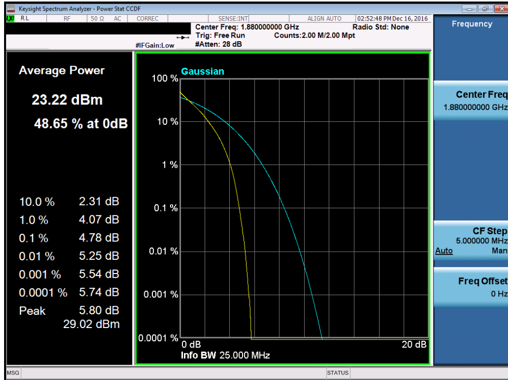
Plot 7-148. PAR Plot (Band 2 – 20.0MHz QPSK – RB Size 100)
