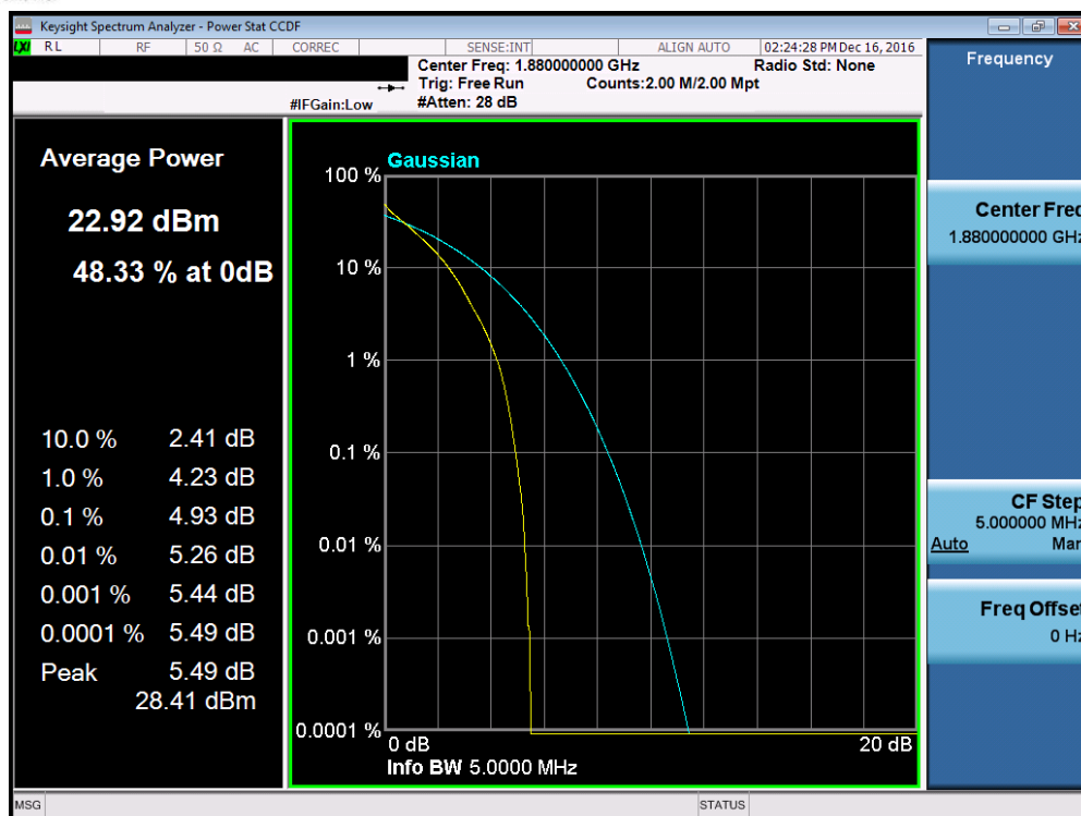
Plot 7-142. PAR Plot (Band 2 – 5.0MHz QPSK – RB Size 25)
