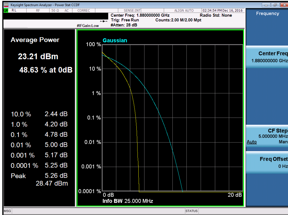
Plot 7-146. PAR Plot (Band 2 – 15.0MHz QPSK – RB Size 75)
