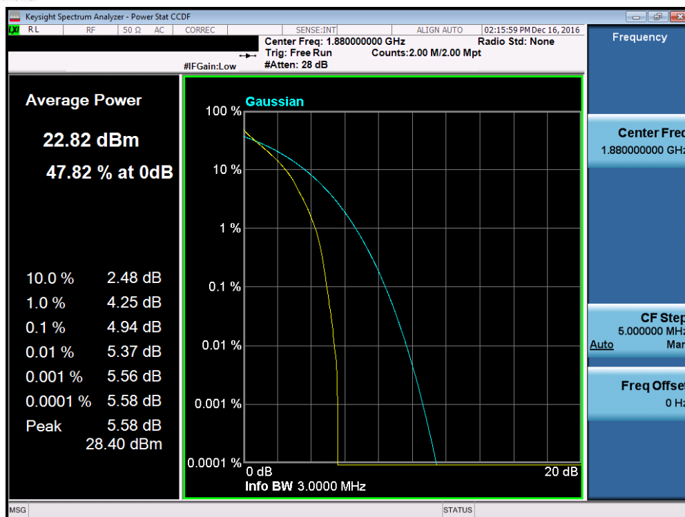
Plot 7-140. PAR Plot (Band 2 – 3.0MHz QPSK – RB Size 15)
