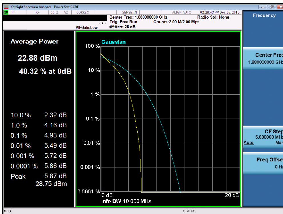
Plot 7-144. PAR Plot (Band 2 – 10.0MHz QPSK – RB Size 50)
