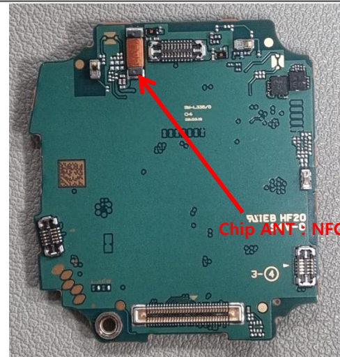
PBA Top
