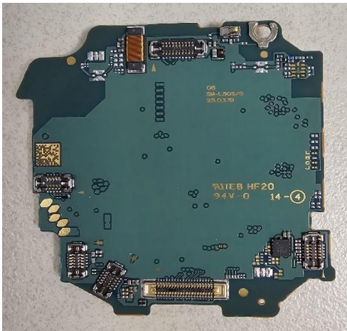
PBA Top
