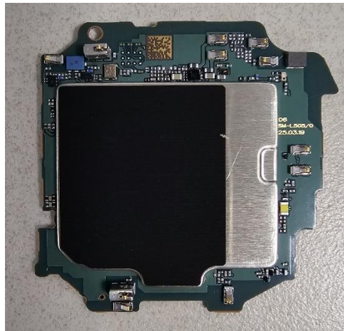
PBA Bottom
