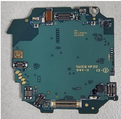
PBA Top
