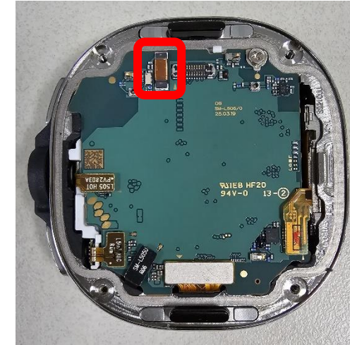
NFC ANT
