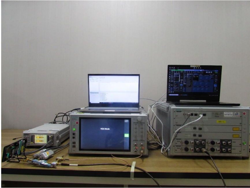
Test setup photo-3(NR NSA)
