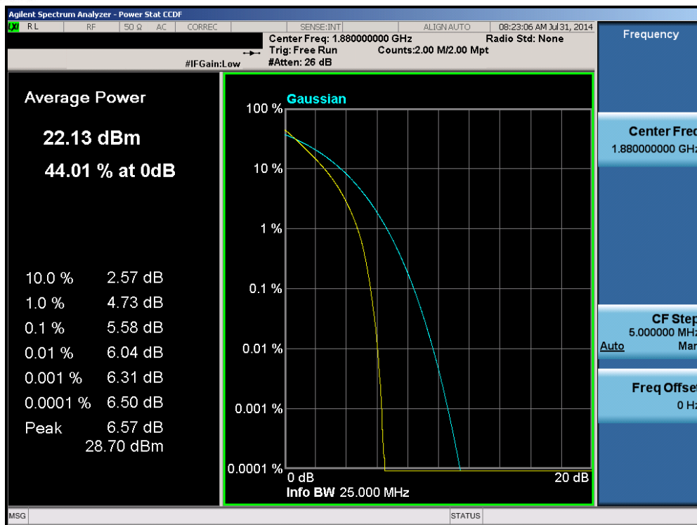
Plot 6-123. PAR Plot (Band 2 – 20.0MHz QPSK – RB Size 100)
