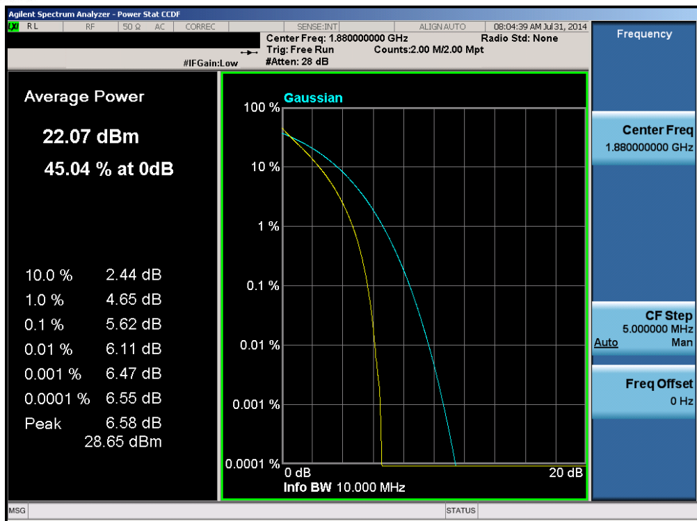
Plot 6-119. PAR Plot (Band 2 – 10.0MHz QPSK – RB Size 50)
