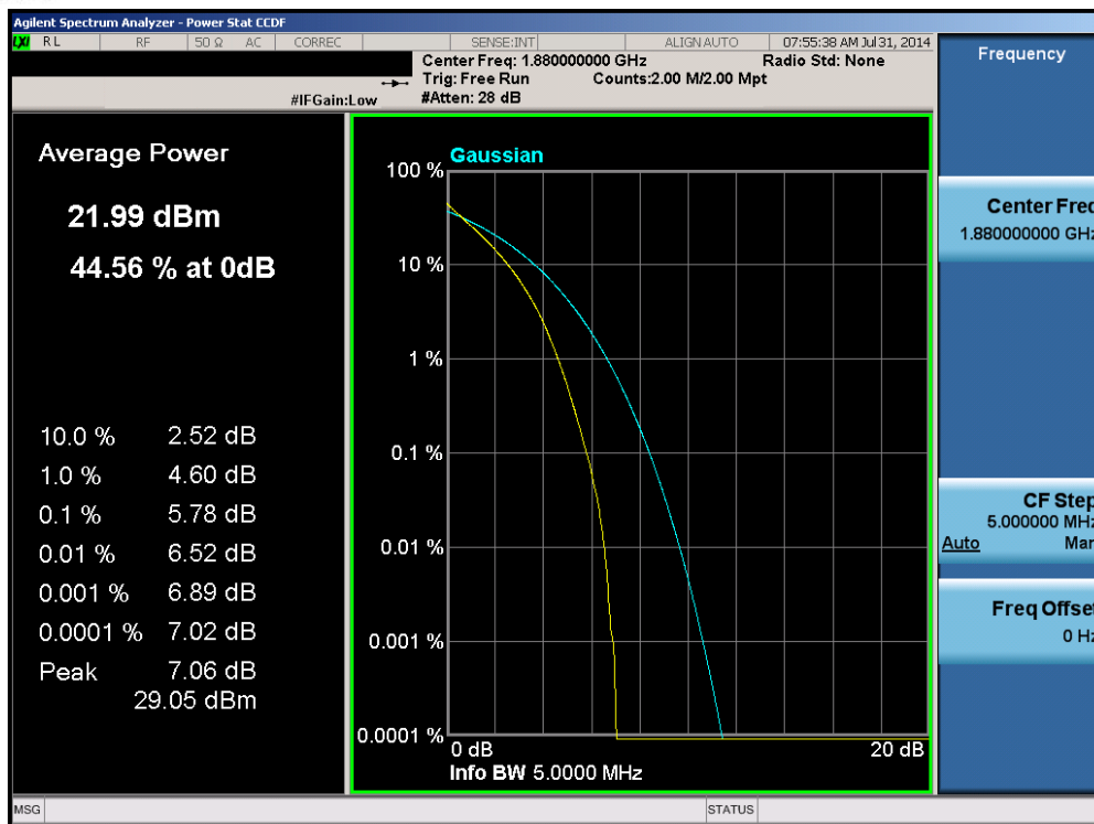
Plot 6-117. PAR Plot (Band 2 – 5.0MHz QPSK – RB Size 25)
