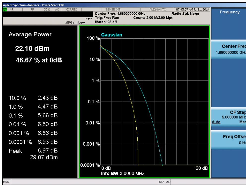
Plot 6-115. PAR Plot (Band 2 – 3.0MHz QPSK – RB Size 15)
