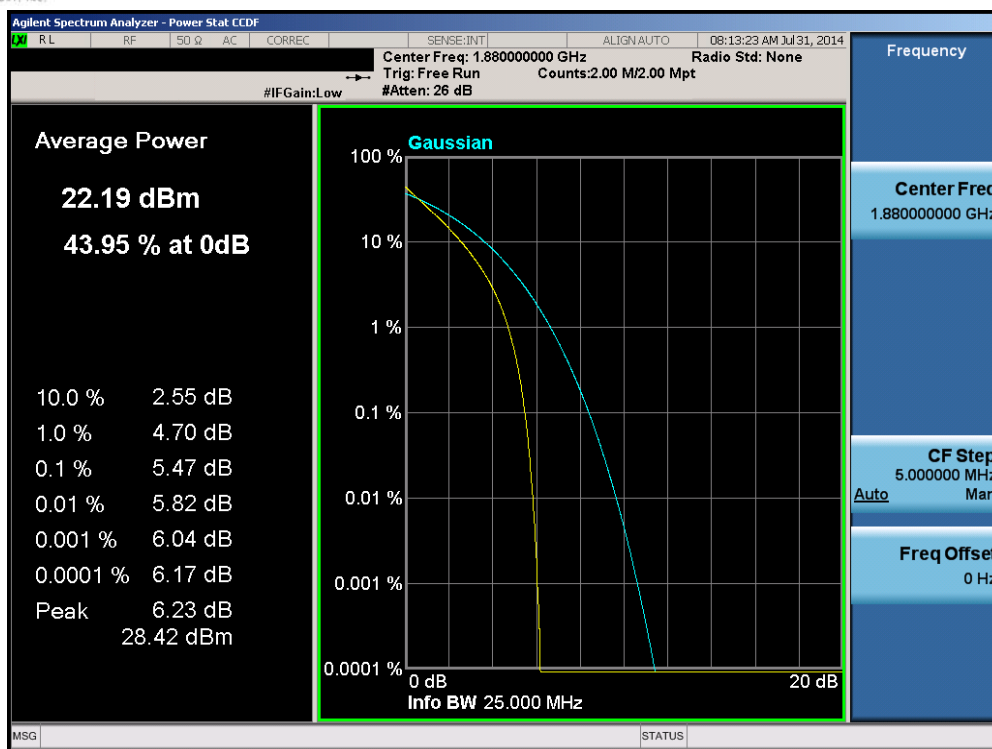
Plot 6-121. PAR Plot (Band 2 – 15.0MHz QPSK – RB Size 75)
