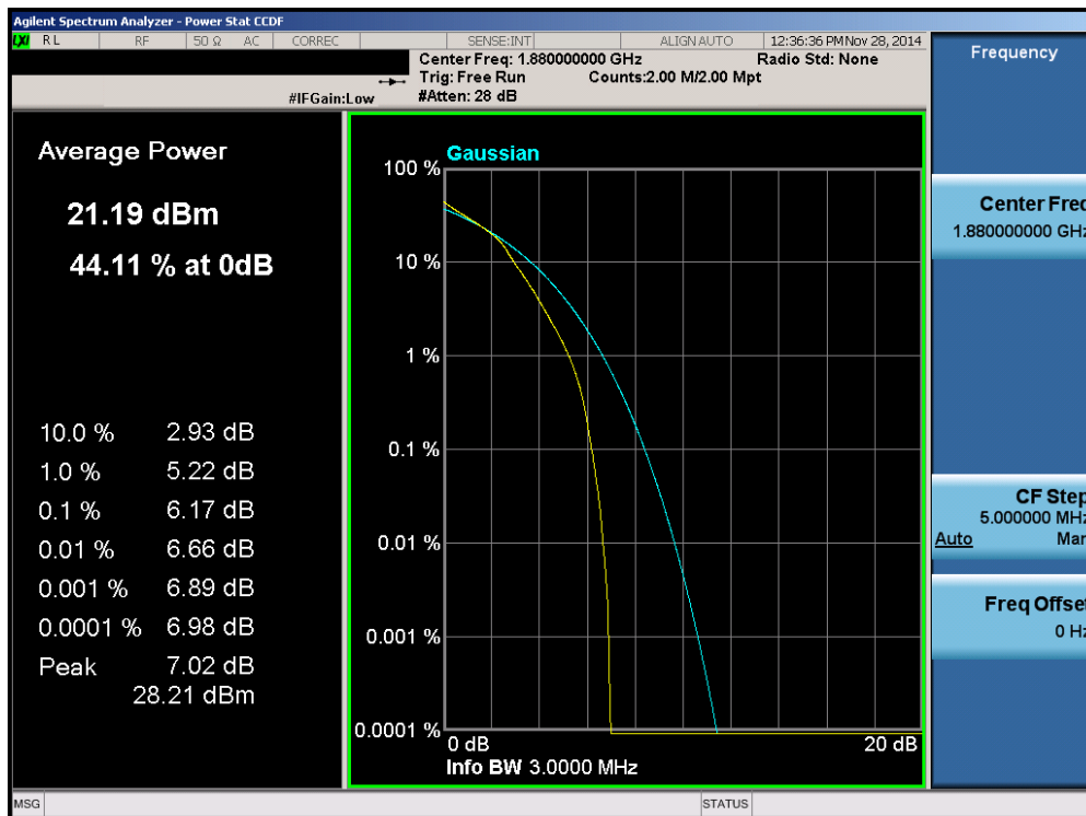
Plot 6-144. PAR Plot (Band 2 - 3.0MHz 16-QAM - RB Size 15)
