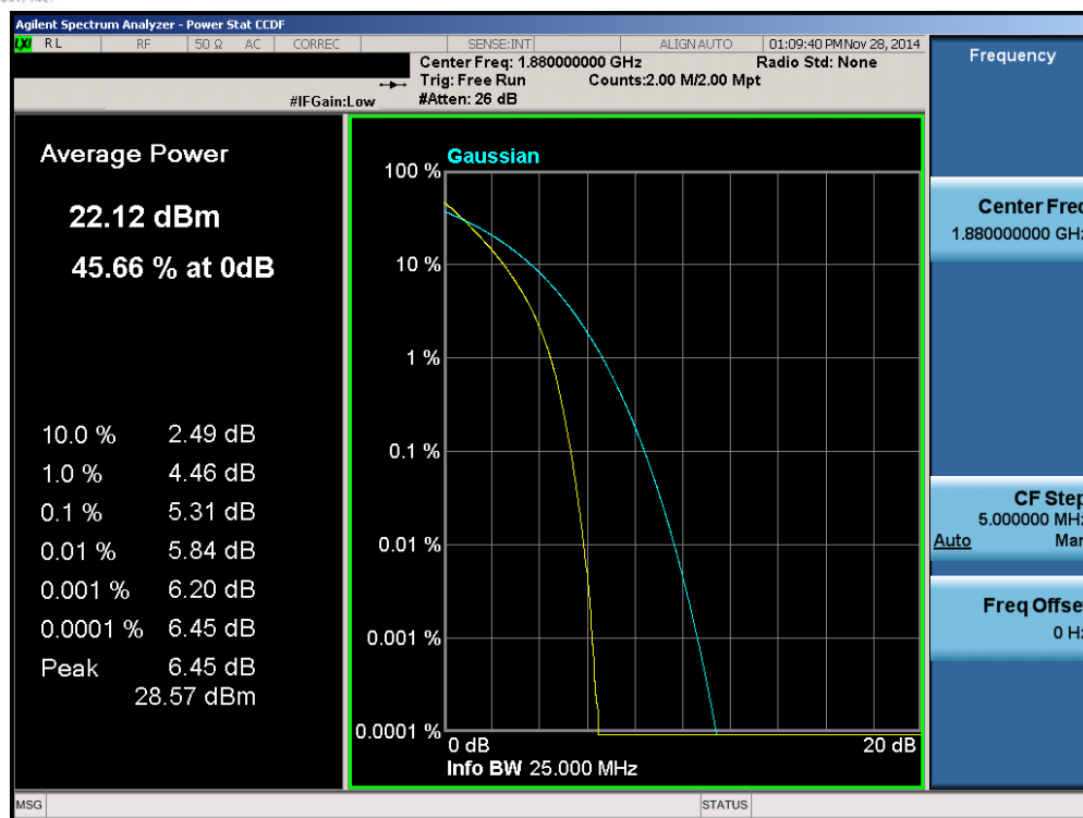
Plot 6-151. PAR Plot (Band 2 – 20.0MHz QPSK – RB Size 100)
