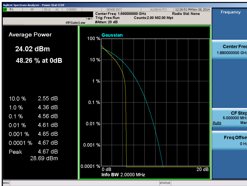
Plot 6-141. PAR Plot (Band 2 – 1.4MHz QPSK – RB Size 6)
