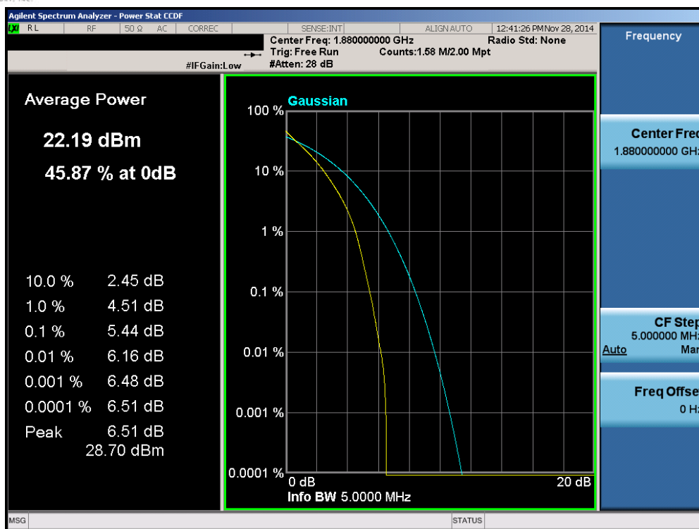
Plot 6-145. PAR Plot (Band 2 – 5.0MHz QPSK – RB Size 25)
