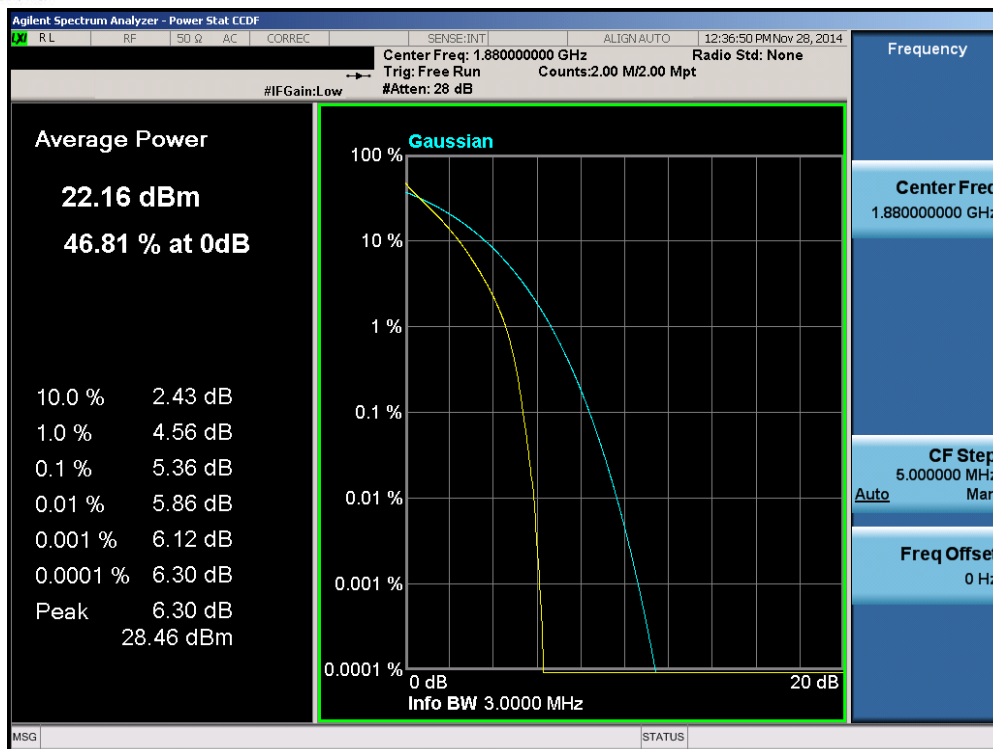
Plot 6-143. PAR Plot (Band 2 - 3.0MHz QPSK - RB Size 15)
