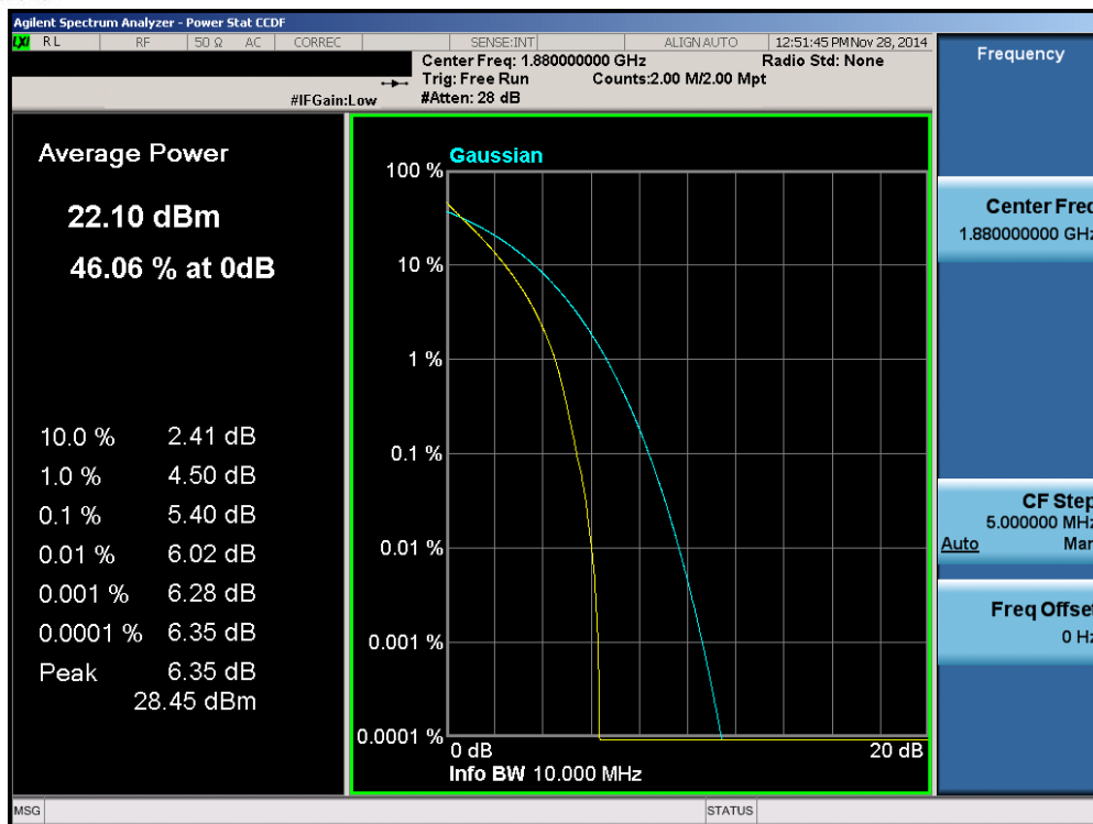
Plot 6-147. PAR Plot (Band 2 – 10.0MHz QPSK – RB Size 50)
