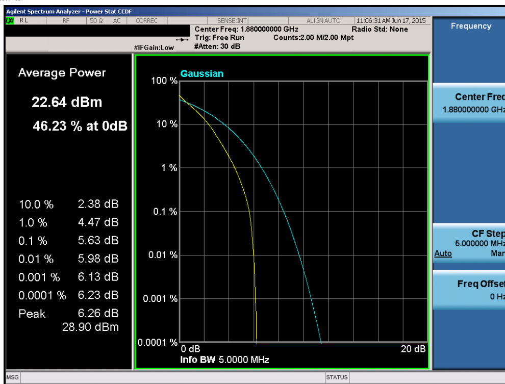
Plot 6-170. PAR Plot (Band 2 – 5.0MHz QPSK – RB Size 25)
