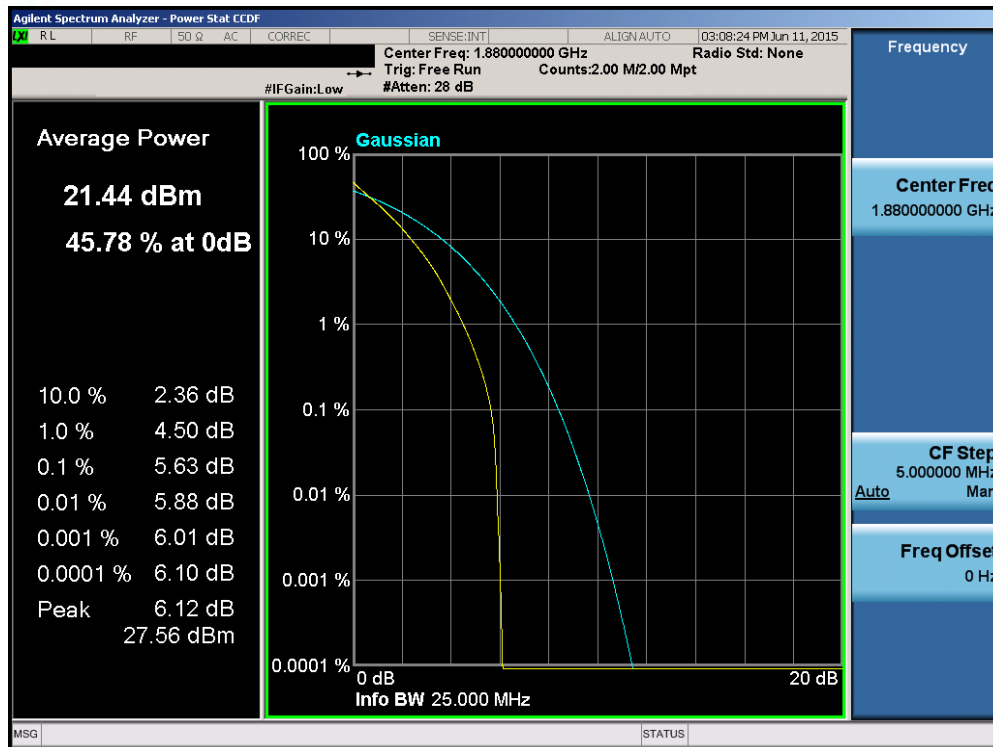
Plot 6-167. PAR Plot (Band 2 – 20.0MHz QPSK – RB Size 100)
