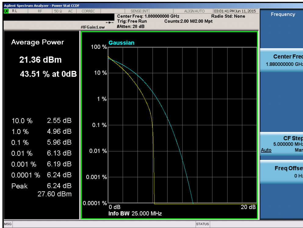
Plot 6-165. PAR Plot (Band 2 – 15.0MHz QPSK – RB Size 75)
