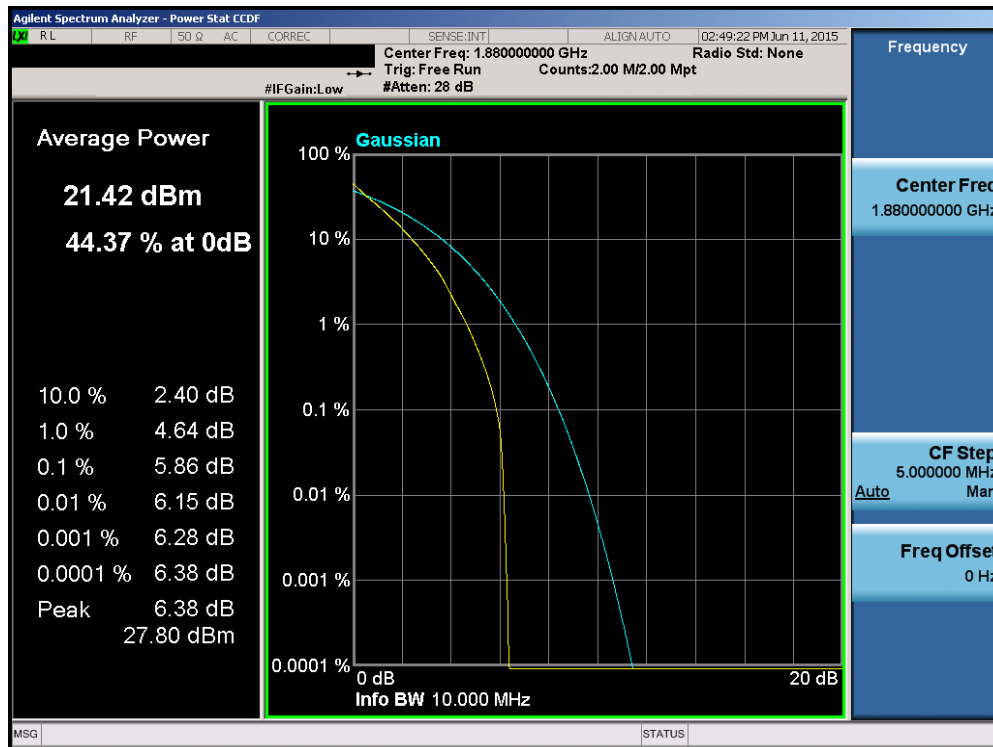
Plot 6-163. PAR Plot (Band 2 – 10.0MHz QPSK – RB Size 50)
