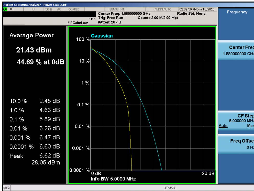
Plot 6-161. PAR Plot (Band 2 – 5.0MHz QPSK – RB Size 25)
