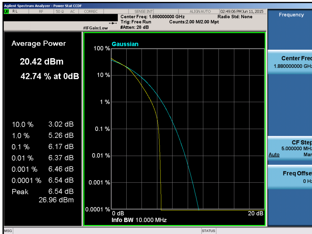
Plot 6-164. PAR Plot (Band 2 – 10.0MHz 16-QAM – RB Size 50)
