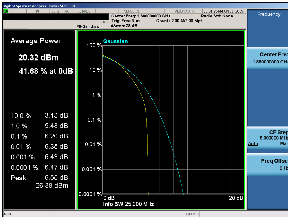
Plot 6-166. PAR Plot (Band 2 – 15.0MHz 16-QAM – RB Size 75)
