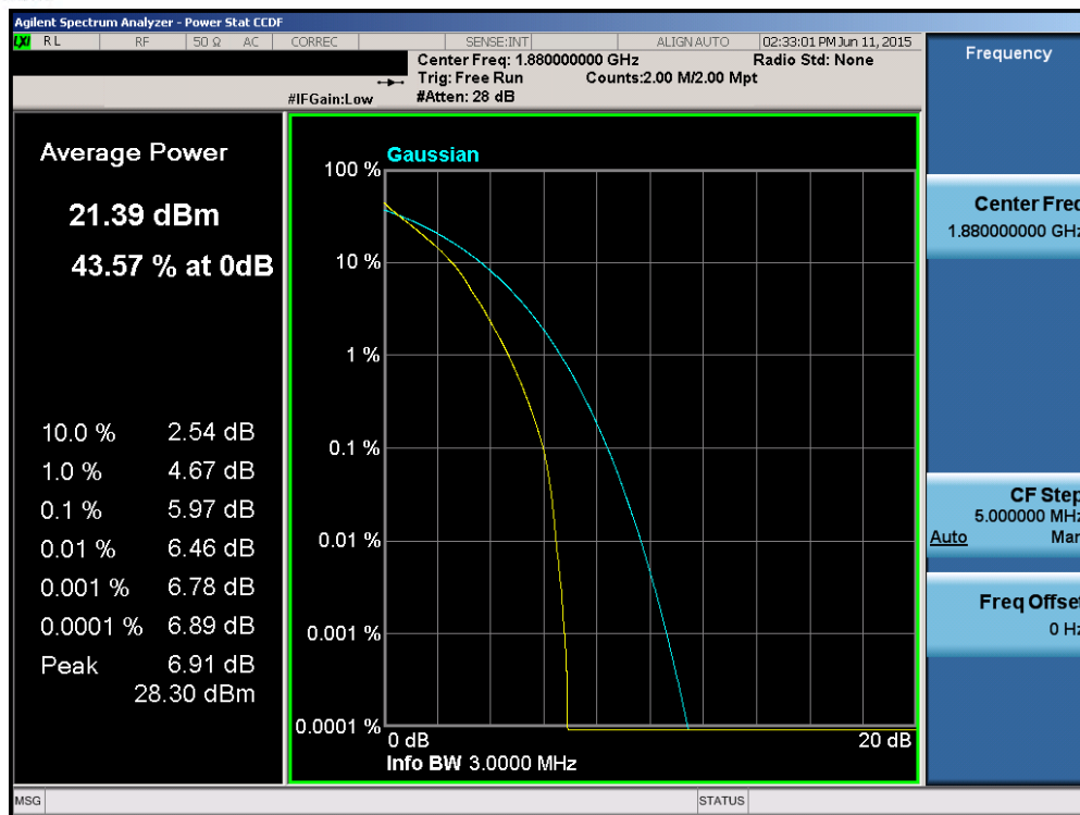
Plot 6-159. PAR Plot (Band 2 – 3.0MHz QPSK – RB Size 15)
