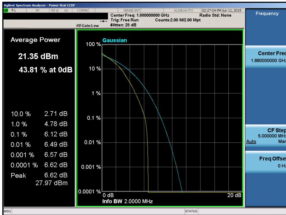
Plot 6-157. PAR Plot (Band 2 – 1.4MHz QPSK – RB Size 6)
