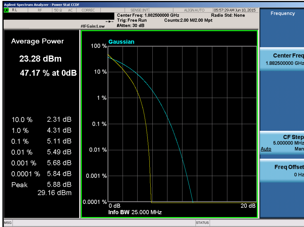
Plot 6-191. PAR Plot (Band 25 – 20.0MHz QPSK – RB Size 100)
