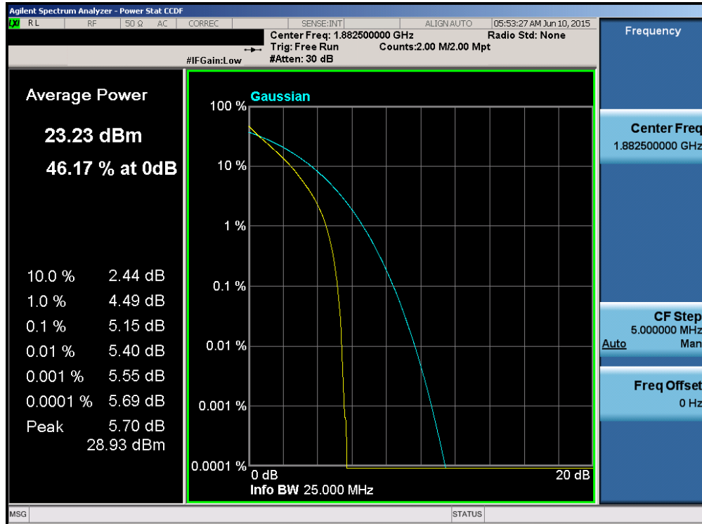
Plot 6-189. PAR Plot (Band 25 – 15.0MHz QPSK – RB Size 75)
