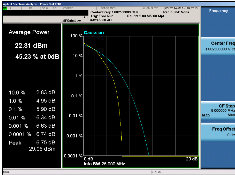
Plot 6-192. PAR Plot (Band 25 – 20.0MHz 16-QAM – RB Size 100)
