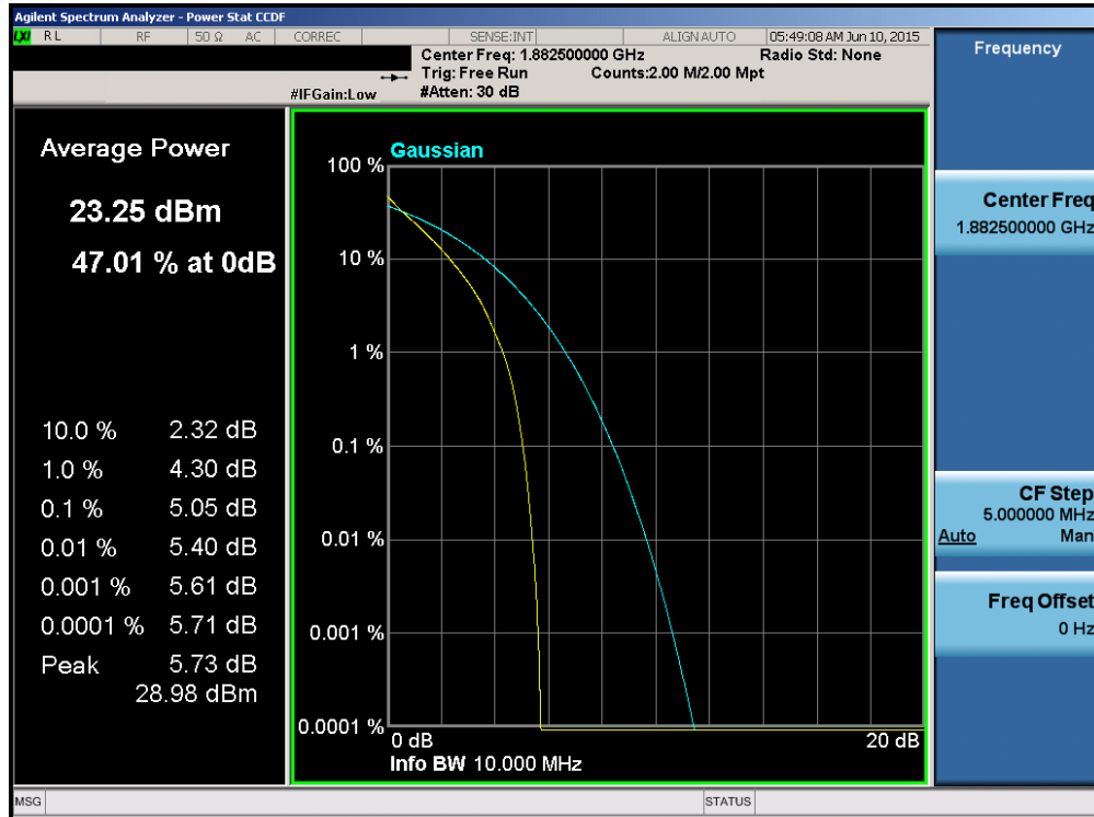
Plot 6-187. PAR Plot (Band 25 – 10.0MHz QPSK – RB Size 50)
