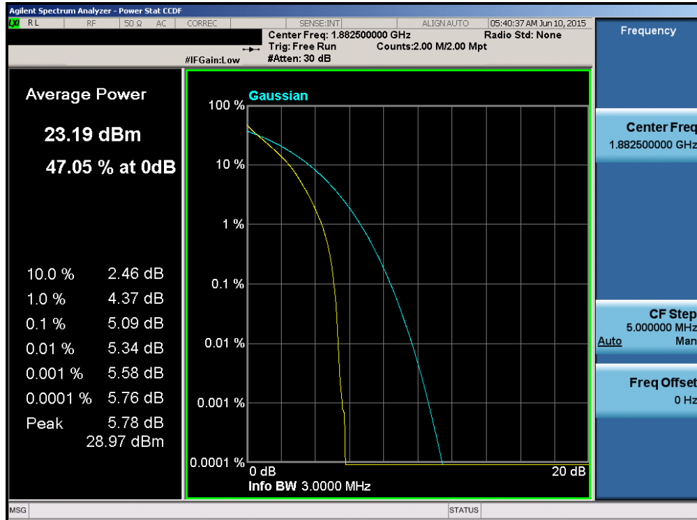
Plot 6-183. PAR Plot (Band 25 – 3.0MHz QPSK – RB Size 15)
