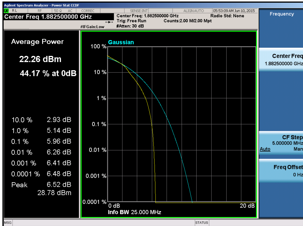
Plot 6-190. PAR Plot (Band 25 – 15.0MHz 16-QAM – RB Size 75)
