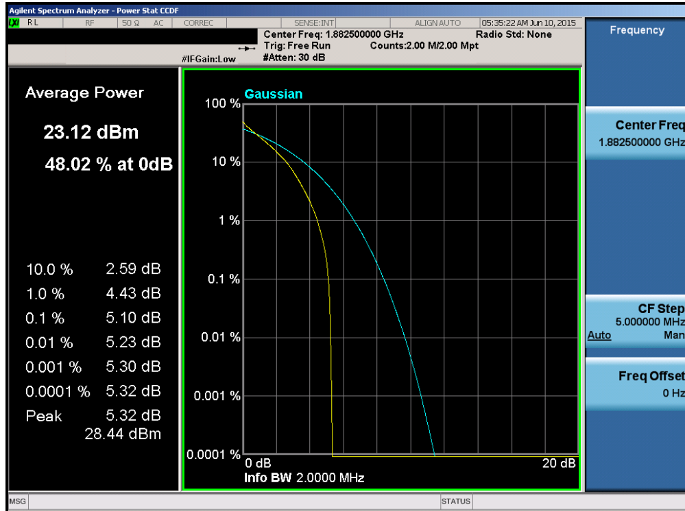
Plot 6-181. PAR Plot (Band 25 – 1.4MHz QPSK – RB Size 6)
