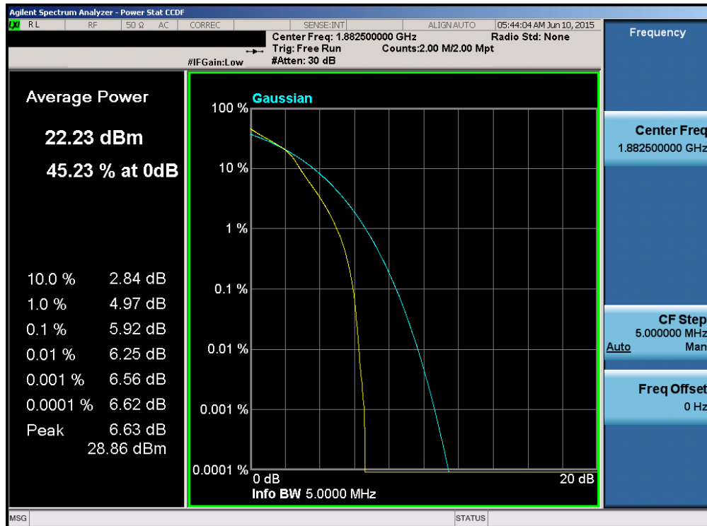
Plot 6-186. PAR Plot (Band 25 – 5.0MHz 16-QAM – RB Size 25)
