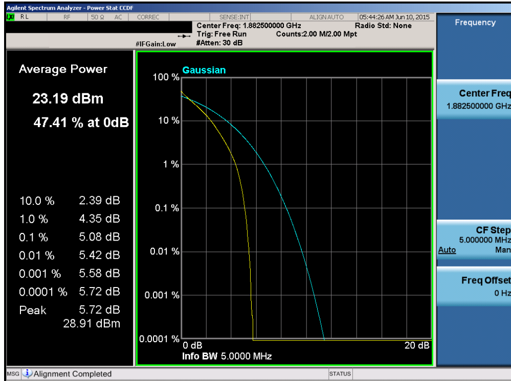
Plot 6-185. PAR Plot (Band 25 – 5.0MHz QPSK – RB Size 25)
