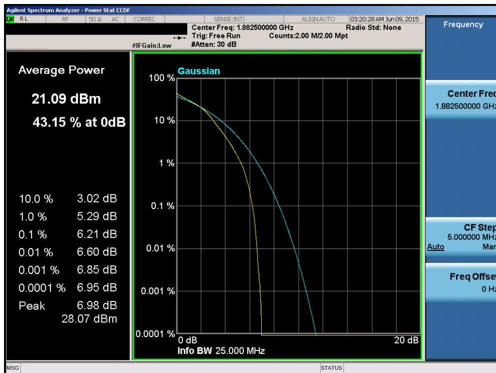
Plot 6-183. PAR Plot (Band 2/25 – 15.0MHz 16-QAM – RB Size 75)
