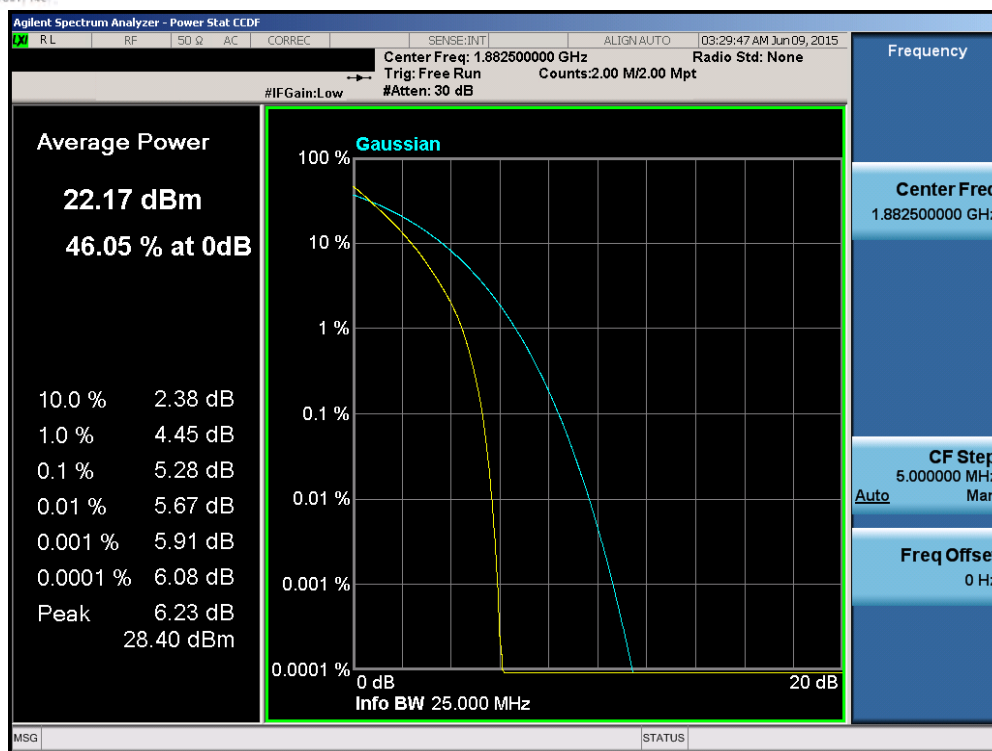
Plot 6-184. PAR Plot (Band 2/25 – 20.0MHz QPSK – RB Size 100)
