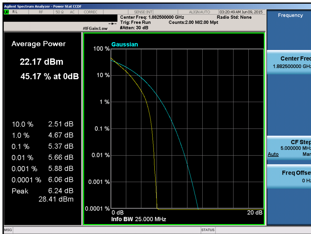
Plot 6-182. PAR Plot (Band 2/25 – 15.0MHz QPSK – RB Size 75)
