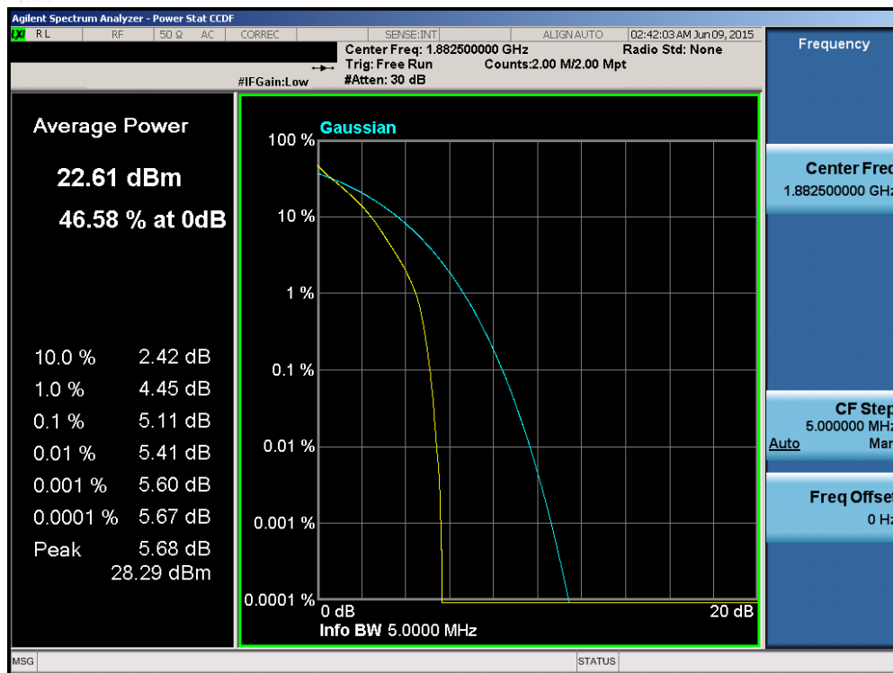
Plot 6-178. PAR Plot (Band 2/25 – 5.0MHz QPSK – RB Size 25)
