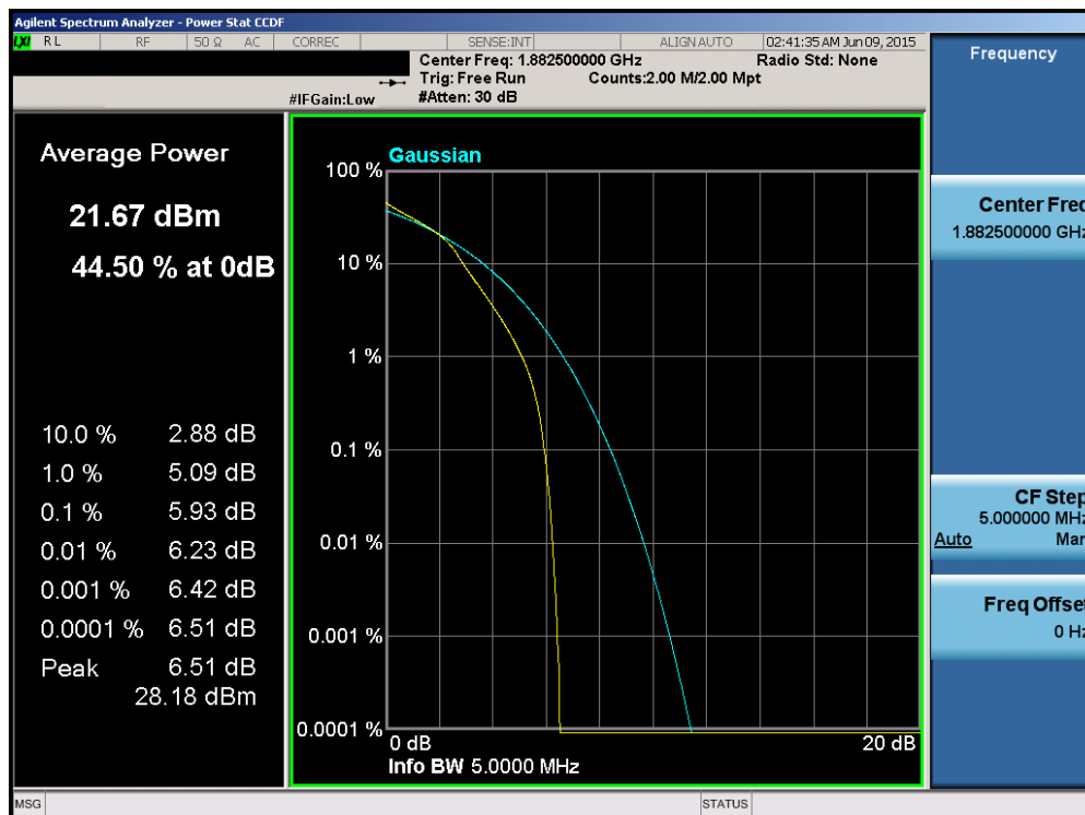
Plot 6-179. PAR Plot (Band 2/25 – 5.0MHz 16-QAM – RB Size 25)
