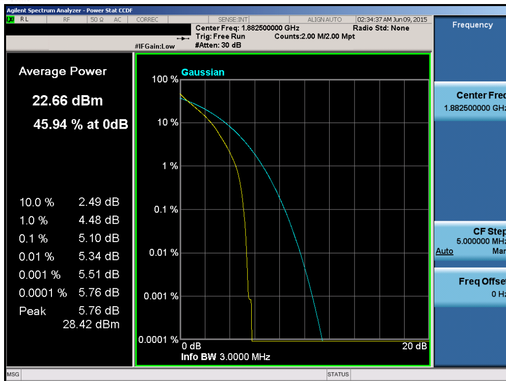
Plot 6-176. PAR Plot (Band 2/25 – 3.0MHz QPSK – RB Size 15)
