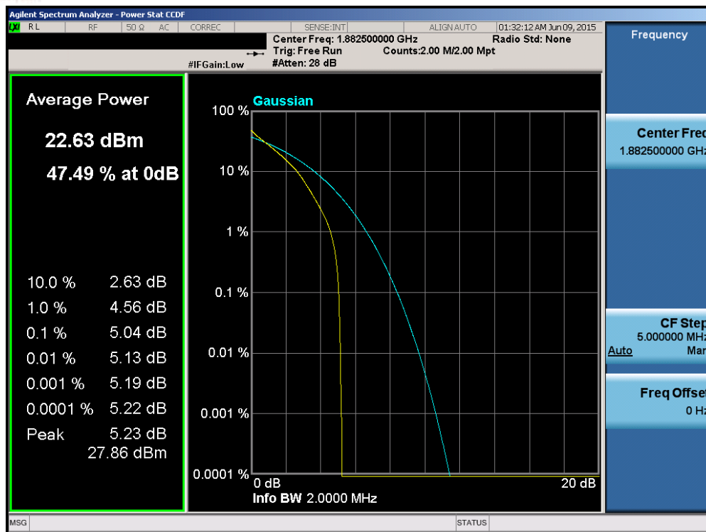
Plot 6-174. PAR Plot (Band 2/25 – 1.4MHz QPSK – RB Size 6)
