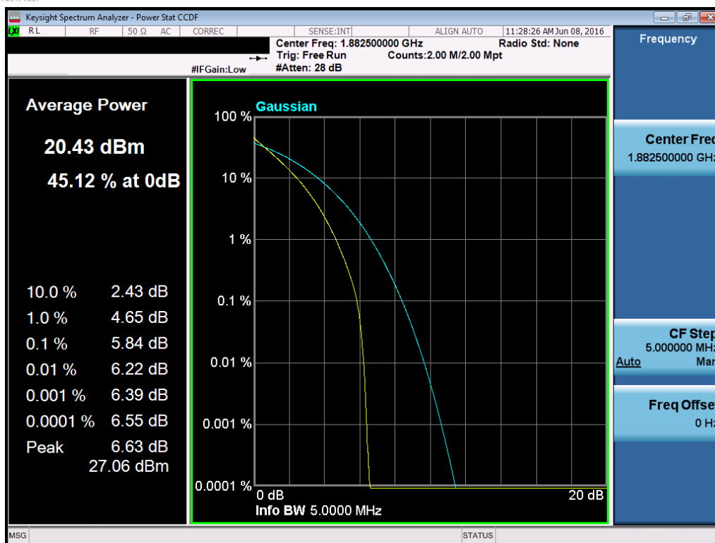
Plot 7-182. PAR Plot (Band 2/25 – 5.0MHz QPSK – RB Size 25)
