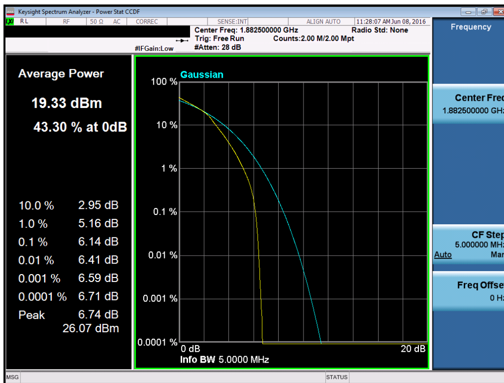
Plot 7-183. PAR Plot (Band 2/25 – 5.0MHz 16-QAM – RB Size 25)
