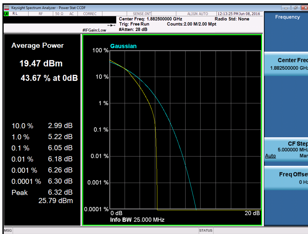
Plot 7-187. PAR Plot (Band 2/25 – 15.0MHz 16-QAM – RB Size 75)
