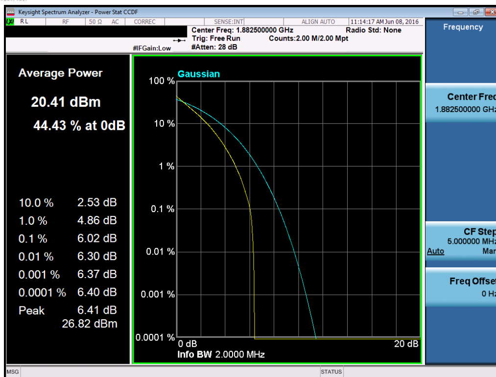
Plot 7-178. PAR Plot (Band 2/25 – 1.4MHz QPSK – RB Size 6)
