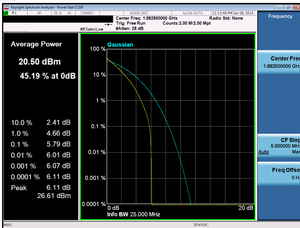
Plot 7-186. PAR Plot (Band 2/25 – 15.0MHz QPSK – RB Size 75)
