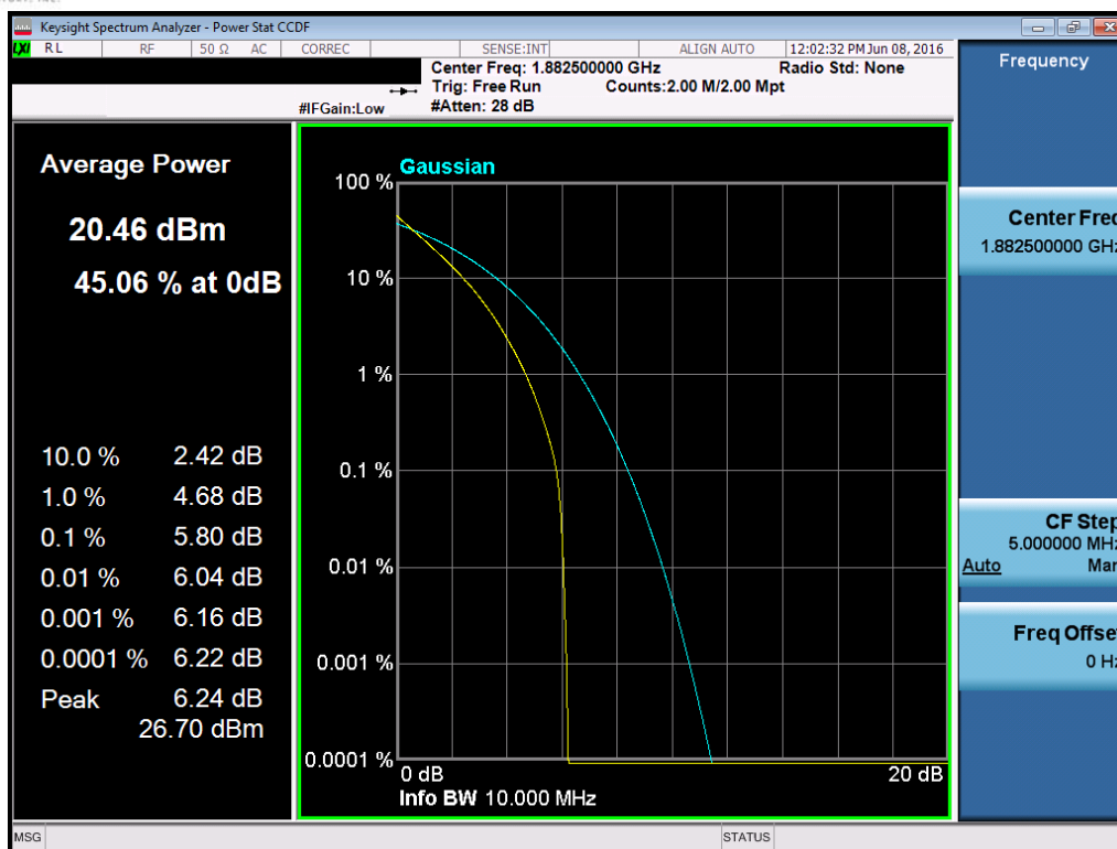
Plot 7-184. PAR Plot (Band 2/25 – 10.0MHz QPSK – RB Size 50)
