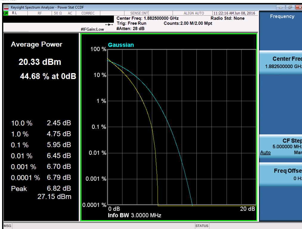
Plot 7-180. PAR Plot (Band 2/25 – 3.0MHz QPSK – RB Size 15)
