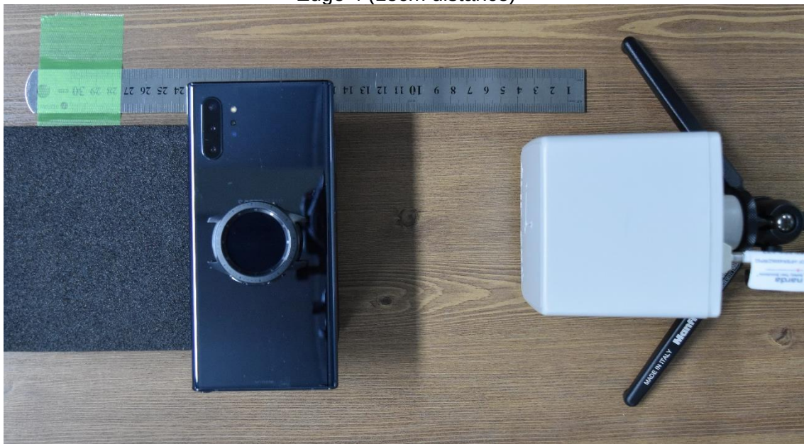
Edge 4 (15cm distance)
