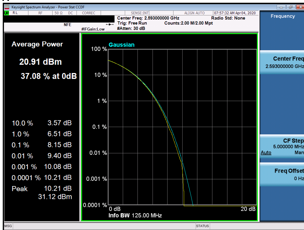
Plot 7-51. PAR Plot (Band n41 - 100.0MHz DFT-s-OFDM-BPSK - Full RB Configuration)
