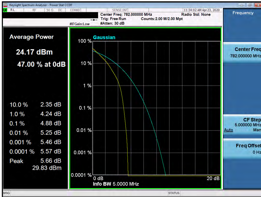
Plot 7-521. PAR Plot (Band 13 - 5.0MHz QPSK - Full RB Configuration)
