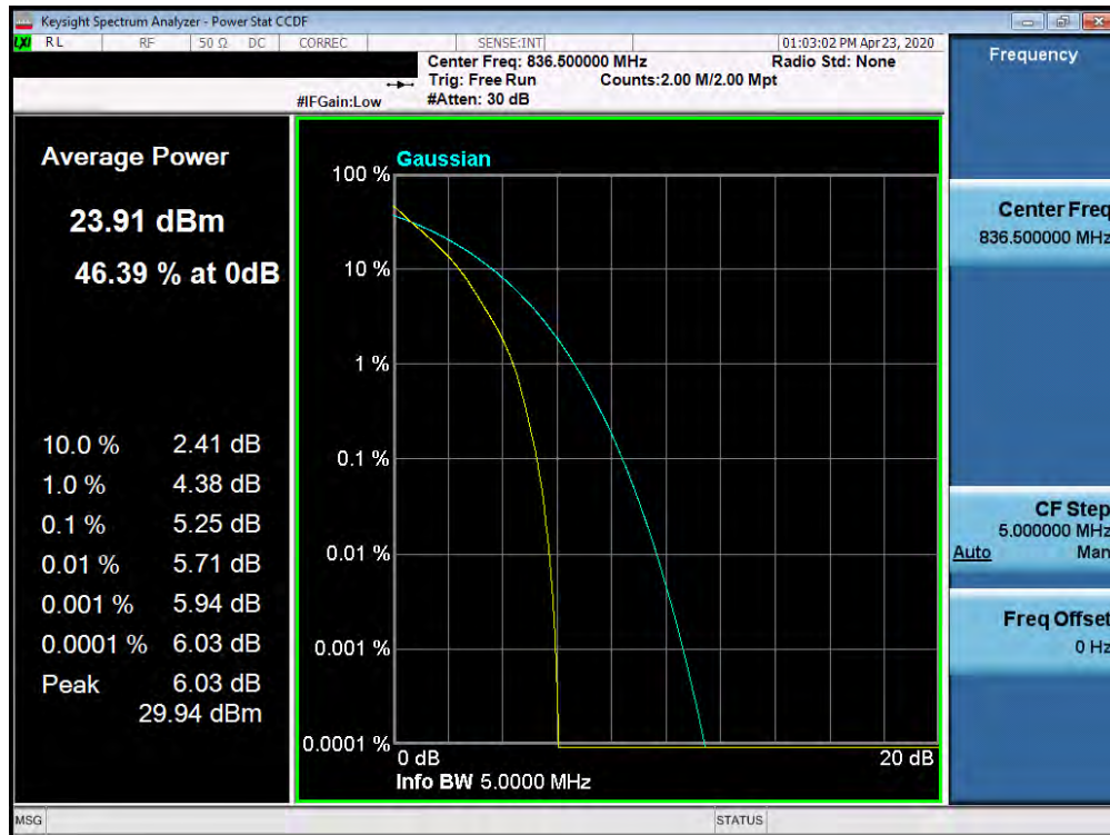
Plot 7-537. PAR Plot (Band 5 - 5.0MHz QPSK - Full RB Configuration)
