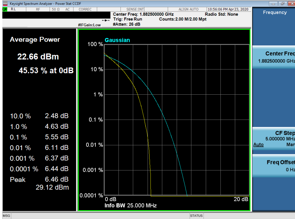
Plot 7-561. PAR Plot (Band 25/2 - 15.0MHz QPSK - Full RB Configuration)
