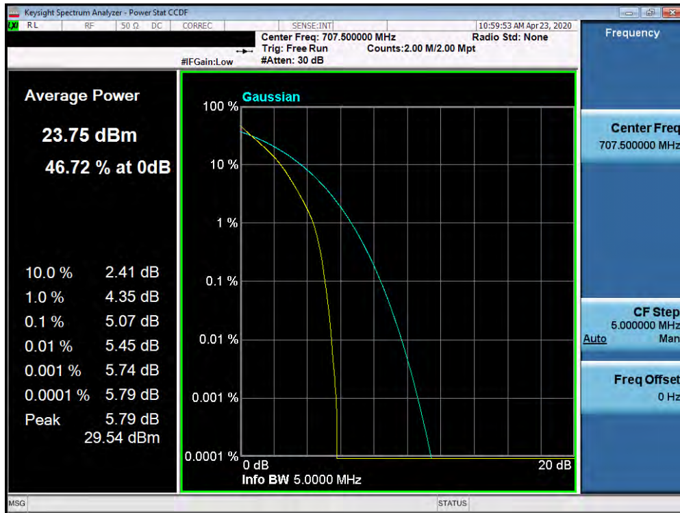
Plot 7-513. PAR Plot (Band 12 - 5.0MHz QPSK - Full RB Configuration)
