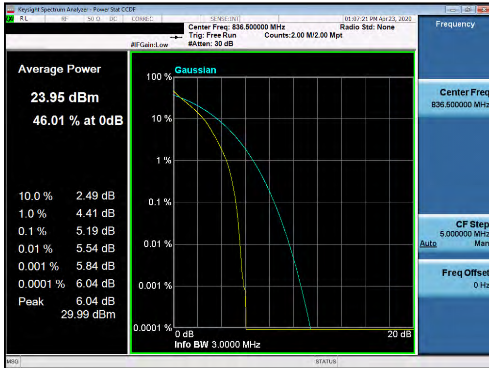
Plot 7-533. PAR Plot (Band 5 - 3.0MHz QPSK - Full RB Configuration)
