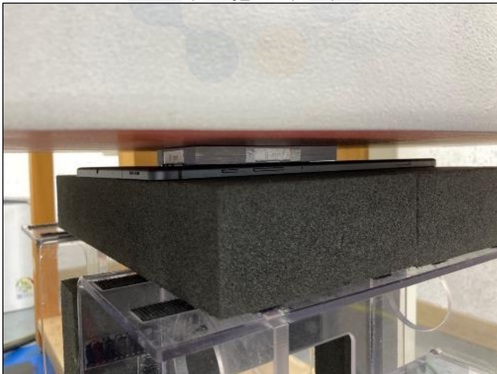
H.2) Body_Rear (9mm)
