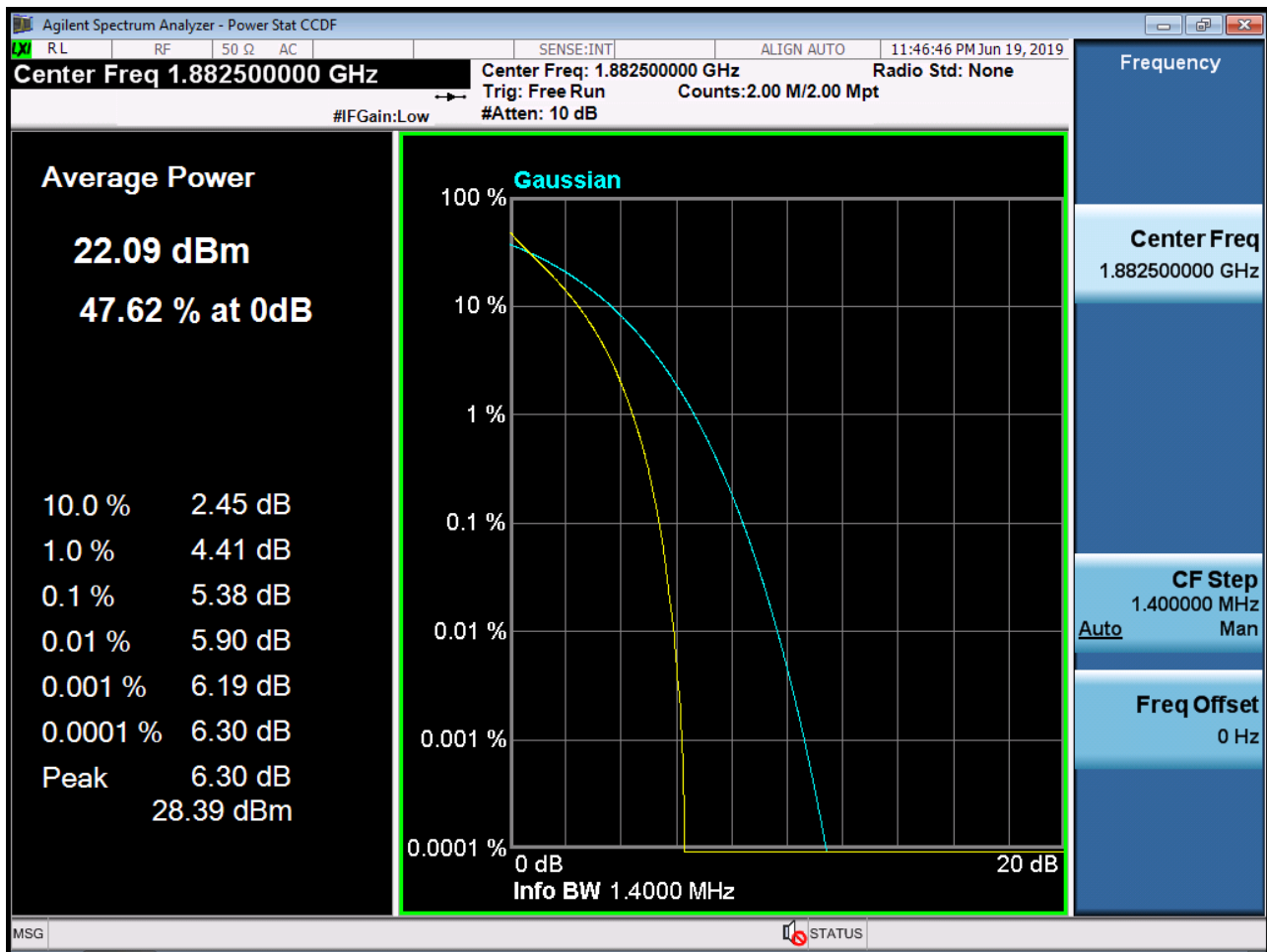
BAND 2. PAR Plot (1.4M BW Ch.26365 QPSK RB 6_0)
