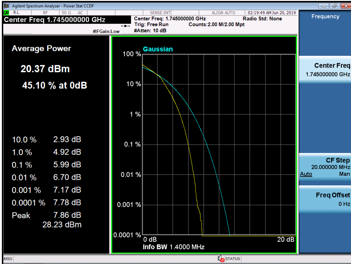
BAND 66. PAR Plot (1.4M BW_Ch.132322_16QAM_RB6_0)
