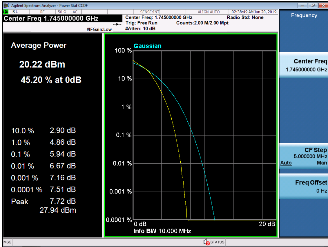
BAND 66. PAR Plot (10M BW_Ch.132322_16QAM_RB50_0)
