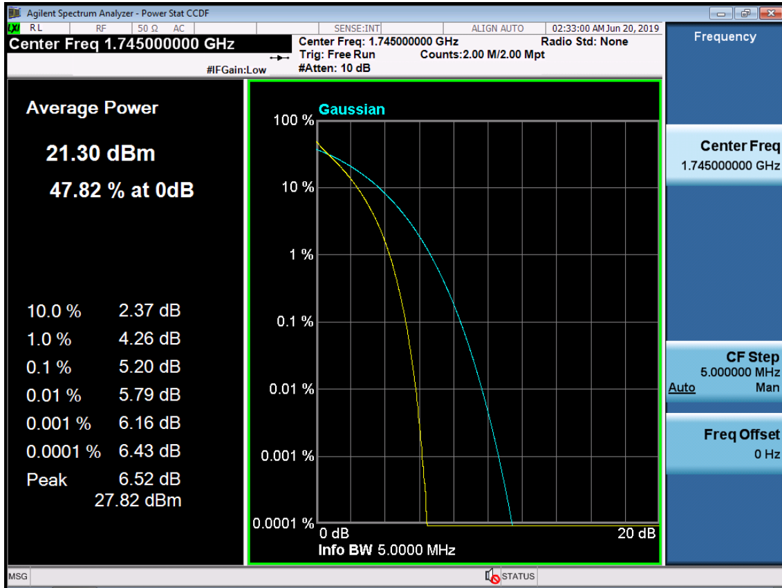
BAND 66. PAR Plot (5M BW_Ch.132322_QPSK_RB25_0)
