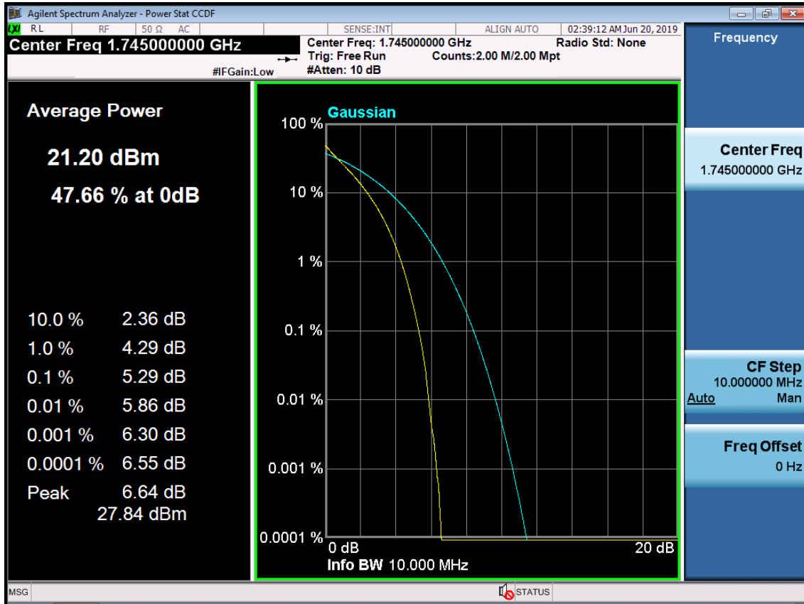
BAND 66. PAR Plot (10M BW_Ch.132322_QPSK_RB50_0)
