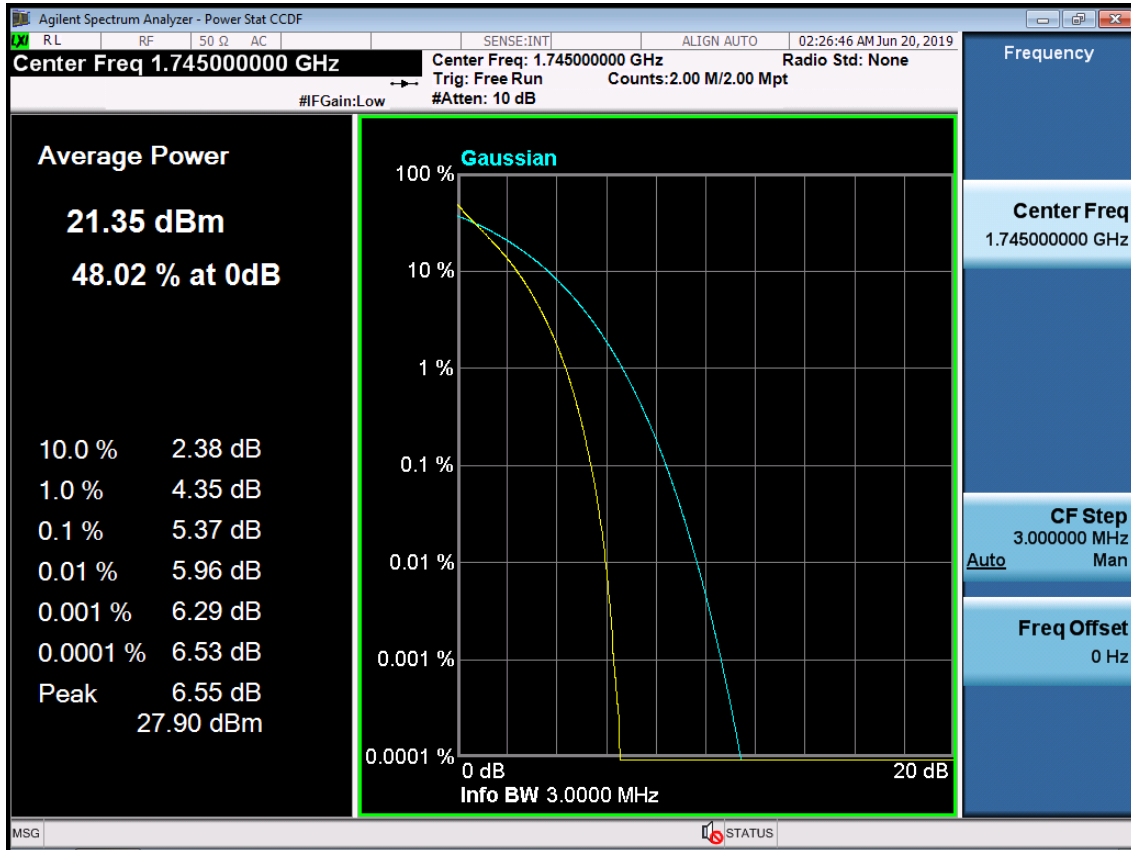
BAND 66. PAR Plot (3M BW_Ch.132322_QPSK_RB15_0)
