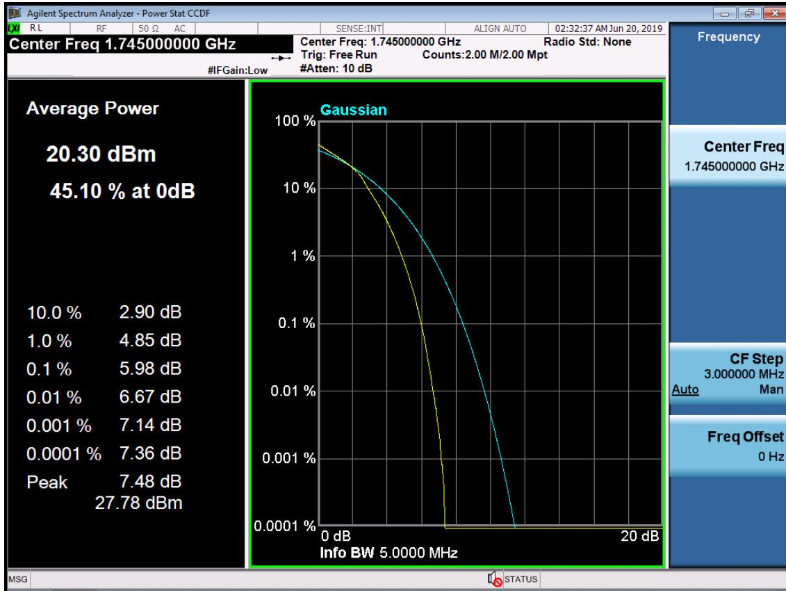
BAND 66. PAR Plot (5M BW_Ch.132322_16QAM_RB25_0)
