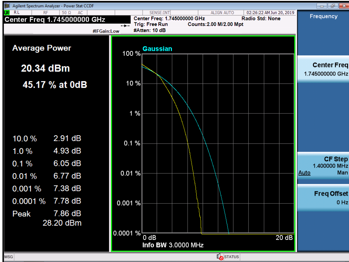
BAND 66. PAR Plot (3M BW_Ch.132322_16QAM_RB15_0)
