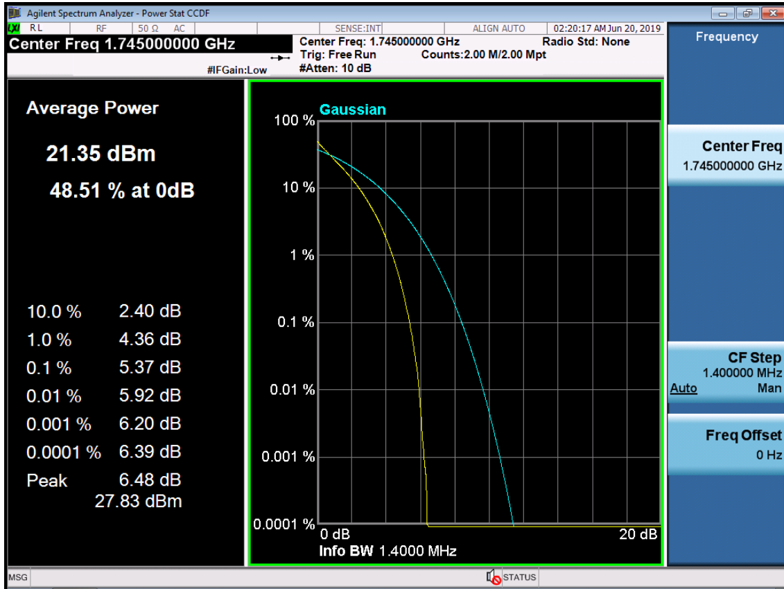
BAND 66. PAR Plot (1.4M BW_Ch.132322_QPSK_RB6_0)
