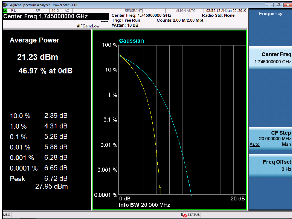
BAND 66. PAR Plot (20M BW_Ch.132322_QPSK_RB100_0)
