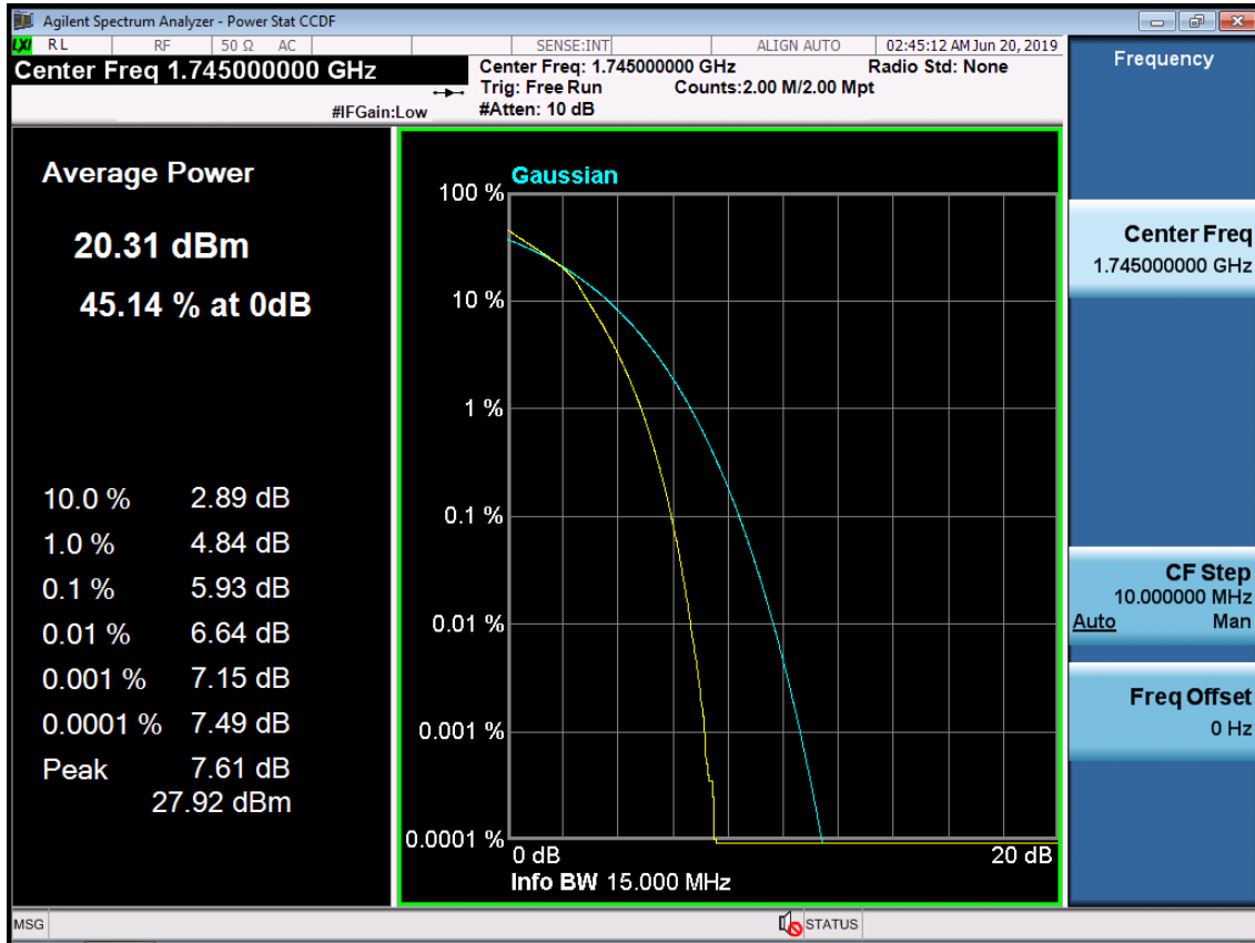
BAND 66. PAR Plot (15M BW_Ch.132322_16QAM_RB75_0)
