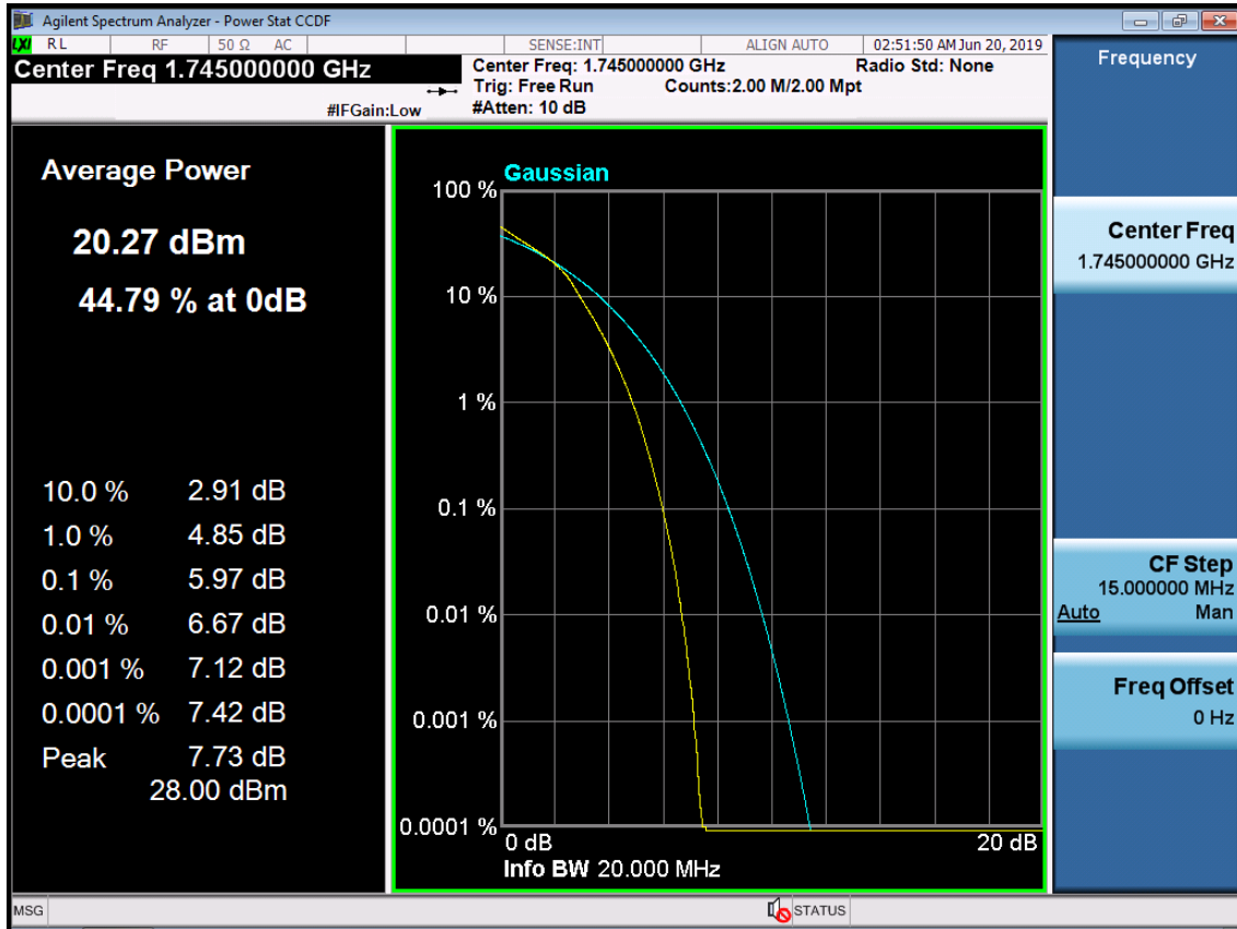
BAND 66. PAR Plot (20M BW_Ch.132322_16QAM_RB100_0)
