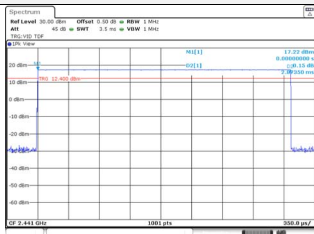
GFSK / DH5
