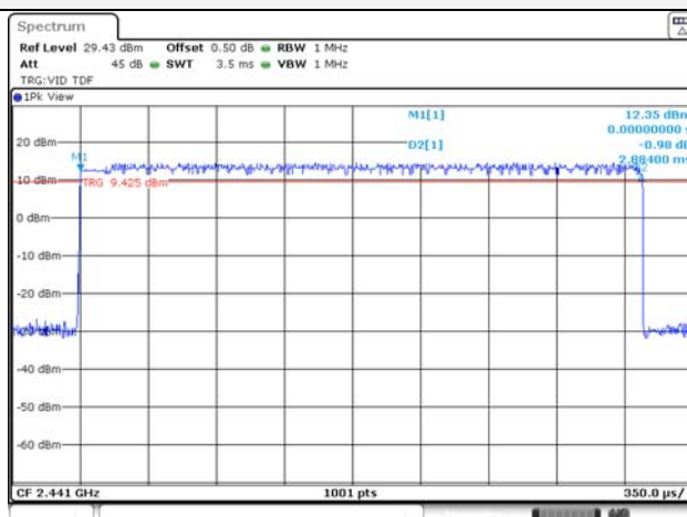
\pi/4 DQPSK / 2-DH5
