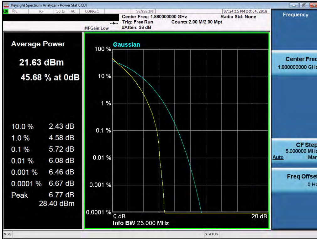
Plot 7-213. PAR Plot (Band 2 - 15.0MHz QPSK - Full RB Configuration)
