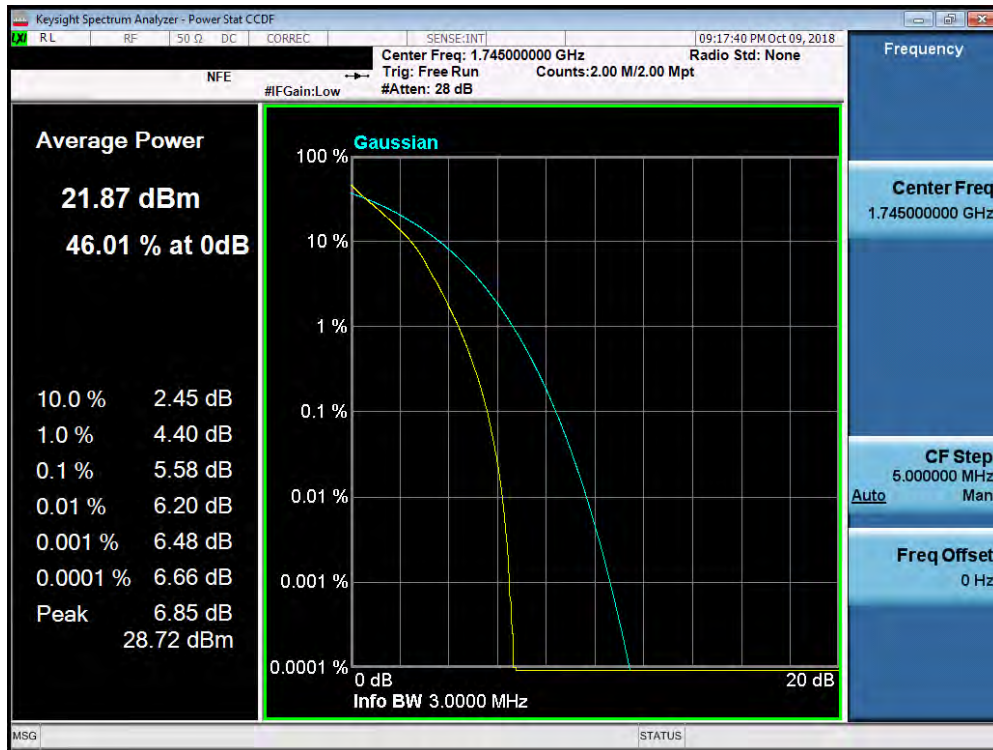
Plot 7-195. PAR Plot (Band 66/4 - 3.0MHz QPSK - Full RB Configuration)
