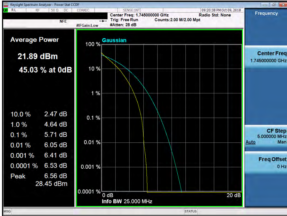
Plot 7-201. PAR Plot (Band 66/4 - 15.0MHz QPSK - Full RB Configuration)
