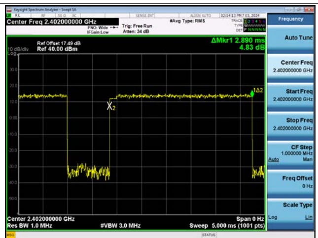
ANT.2 \pi/4 DQPSK : Dwell Time(Ch. 0)
