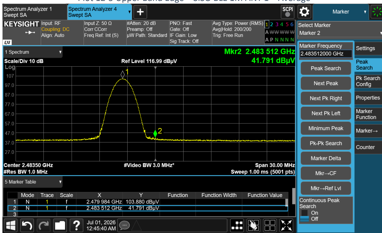
Plot 12-5 Upper Band Edge – SISO BLE 1M ANT 1 – Average
