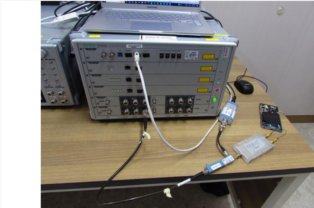
Test setup photo-5 (5G Sub 6 SA)
