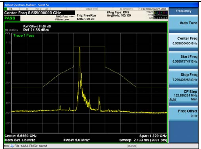
802.11be EHT160M Ch.143(6665 MHz) 242 Tones 61 RU
