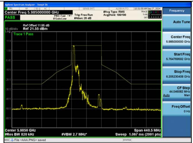
802.11be EHT80M Ch.7(5985 MHz) 242 Tones 61 RU
