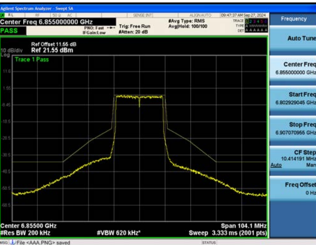
802.11be EHT20M Ch.181(6855 MHz) SU
