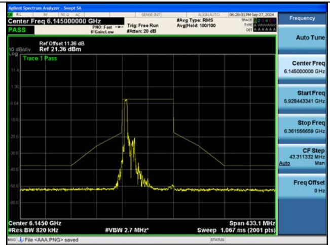
802.11be EHT80M Ch.39(6145 MHz) 242 Tones 61 RU
