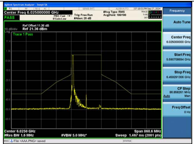
802.11be EHT160M Ch.15(6025 MHz) 242 Tones 61 RU
