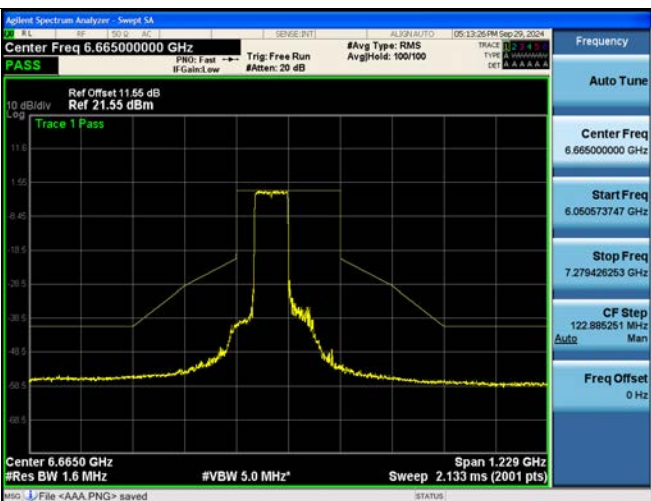
802.11be EHT160M Ch.143(6665 MHz) 996 Tones 67 RU
