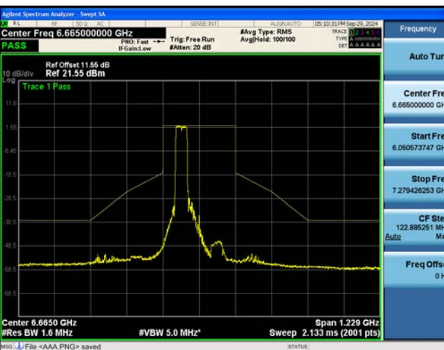
802.11be EHT160M Ch.143(6665 MHz) 484 Tones 65 RU
