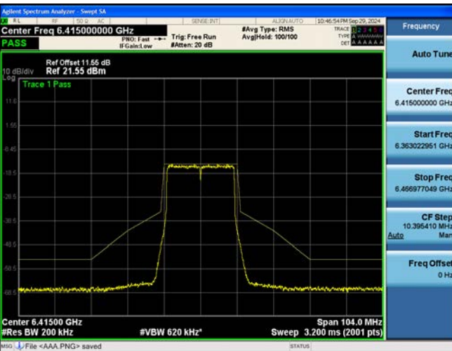
802.11be EHT20M Ch.93(6415 MHz) SU
