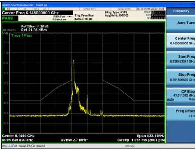
802.11be EHT80M Ch.39(6145 MHz) 106 Tones 53 RU
