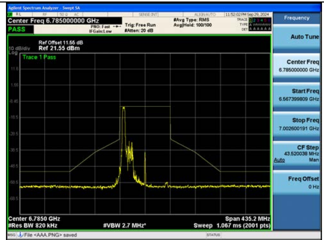
802.11be EHT80M Ch.167(6785 MHz) 242 Tones 61 RU
