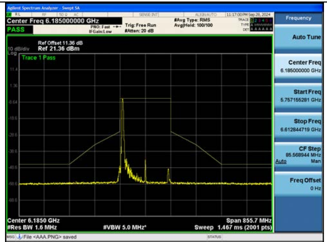
802.11be EHT160M Ch.47(6185 MHz) 242 Tones 61 RU
