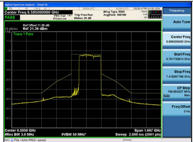
Bandwidth 320M, Ch. 127(6585 MHz) 3x996T RU104
