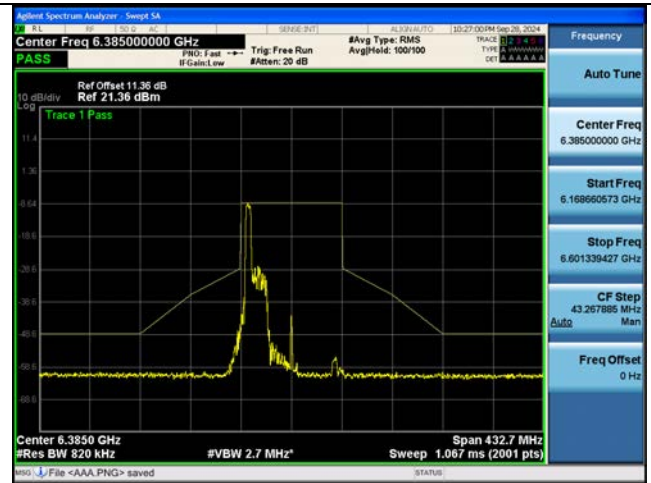
802.11be EHT80M Ch.87(6385 MHz) 242 Tones 61 RU
