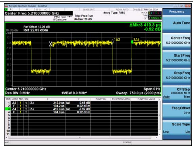
802.11ac(VHT80)
