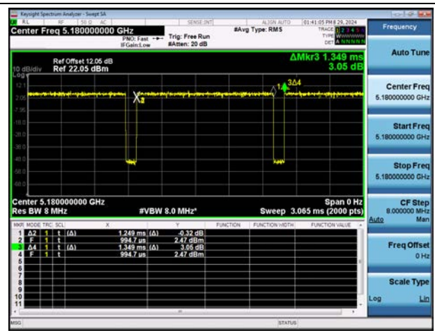
802.11ac(VHT20)
