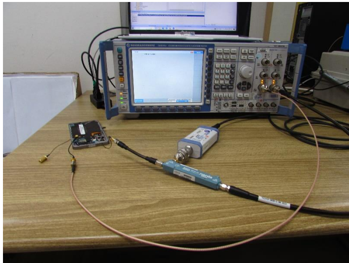
Test setup photo-4 (8-1(d) (WLAN 5 GHz))
