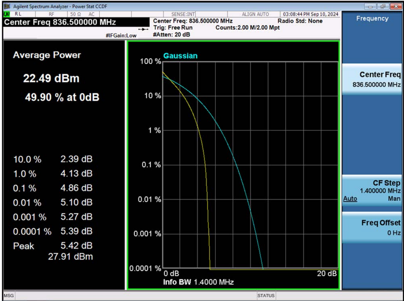
BAND 26. PAR Plot (1.4 M BW Ch.26915 QPSK_RB6_0)
