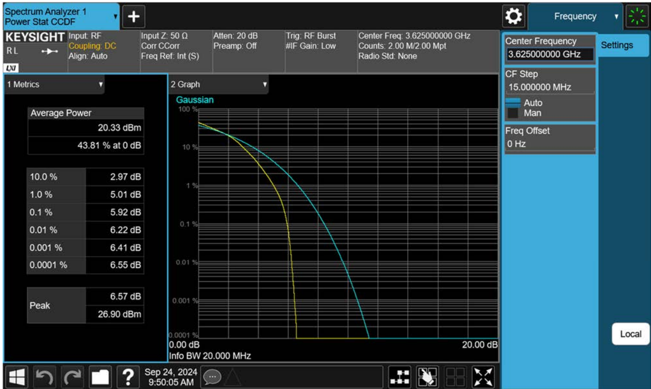
BAND 48. PAR Plot (20 M BW_Ch.55990_16QAM_RB100_0)
