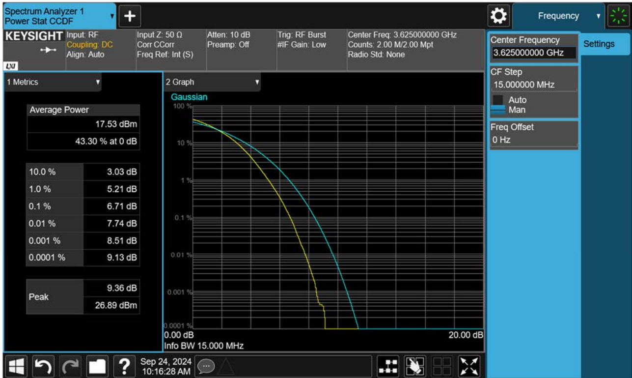
BAND 48. PAR Plot (15 M BW_Ch.55990_256QAM_RB75_0)
