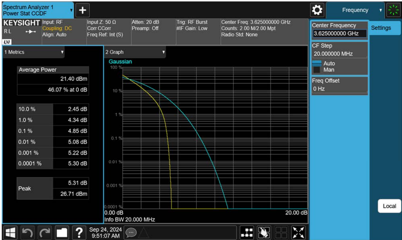
BAND 48. PAR Plot (20 M BW_Ch.55990_QPSK_RB100_0)
