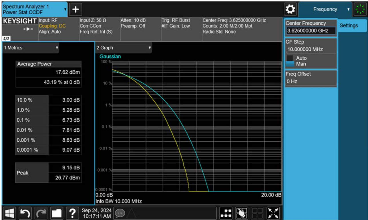
BAND 48. PAR Plot (10 M BW_Ch.55990_256QAM_RB50_0)
