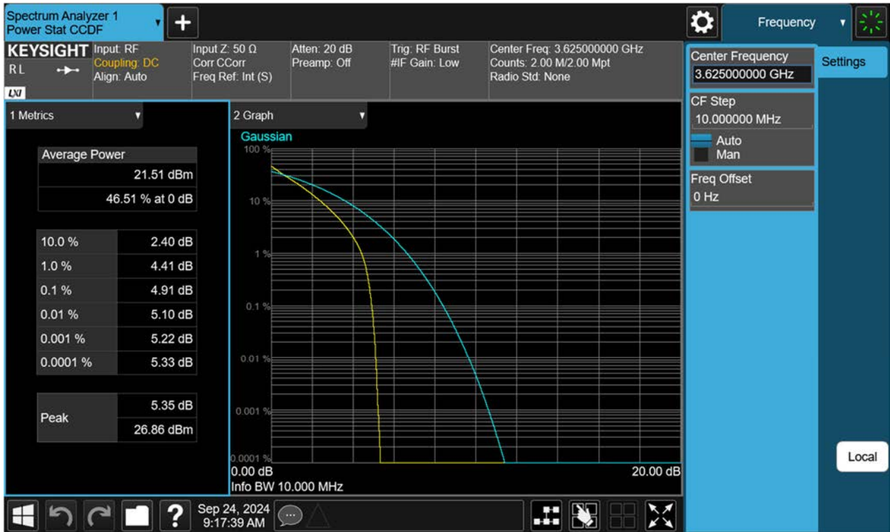
BAND 48. PAR Plot (10 M BW_Ch.55990_QPSK_RB50_0)
