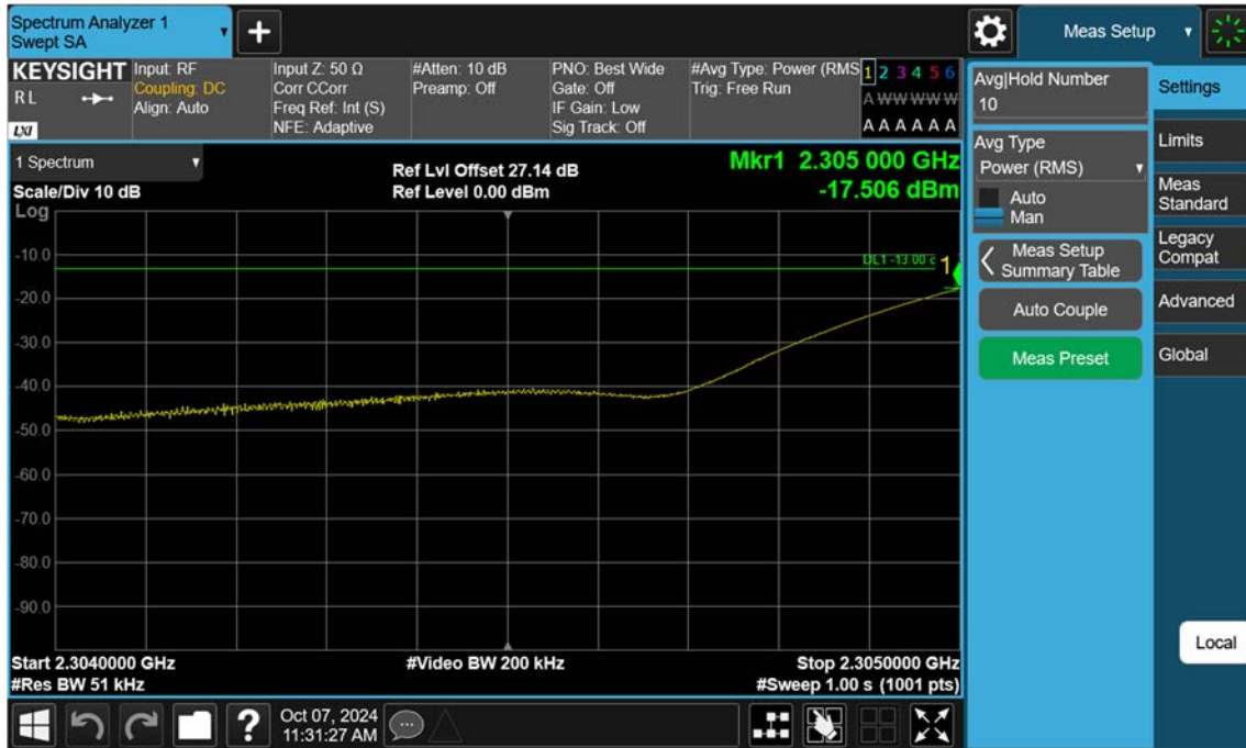
NR30_5 M_Band Edge(2304MHz-2305MHz)_Low_BPSK_1RB
