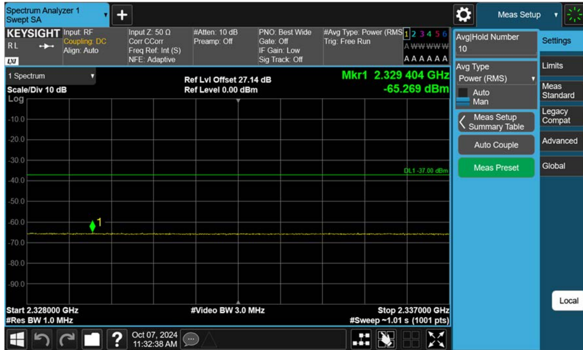
NR30_5 M_Band Edge(2328MHz-2337MHz)_Low_BPSK_1RB
