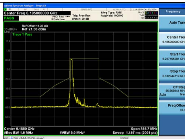
802.11be EHT160M Ch.47(6185 MHz) 996T+484T RU94
