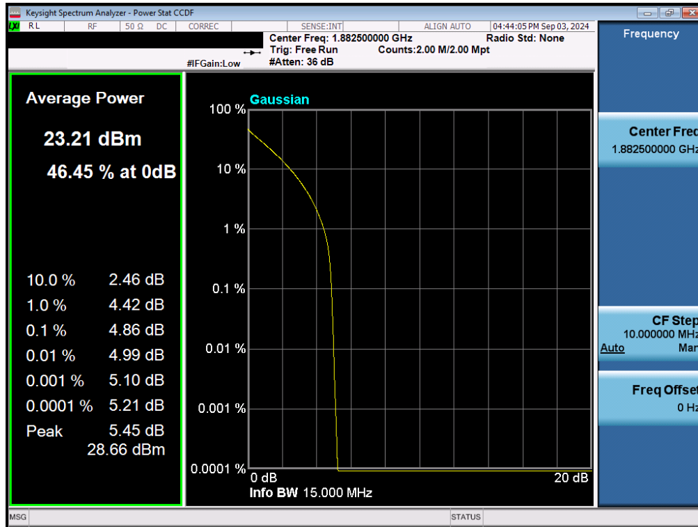
Plot 7-165. PAR Plot (LTE Band 25/2 - 15MHz QPSK - Full RB - Ant1)
