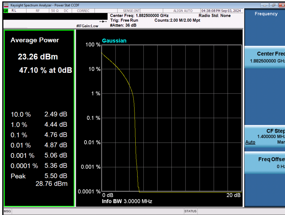
Plot 7-171. PAR Plot (LTE Band 25/2 - 3MHz QPSK - Full RB - Ant1)
