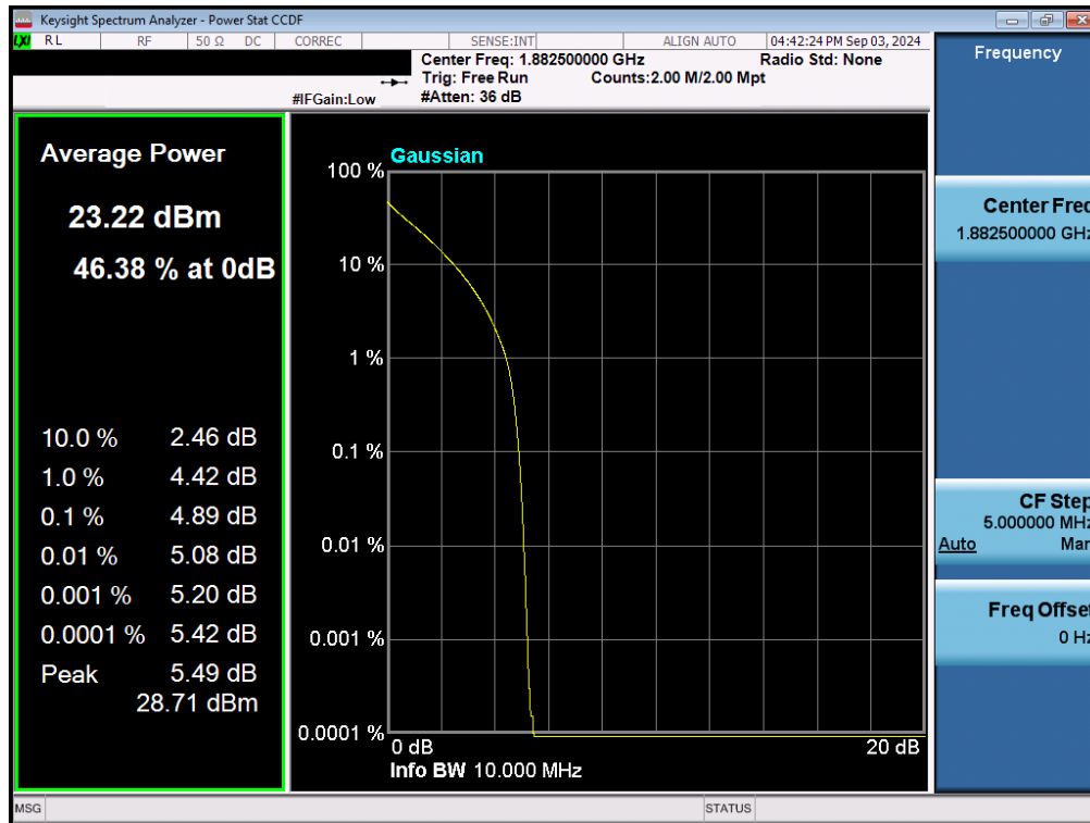
Plot 7-167. PAR Plot (LTE Band 25/2 - 10MHz QPSK - Full RB - Ant1)
