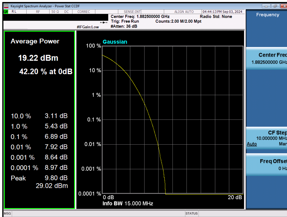
Plot 7-166. PAR Plot (LTE Band 25/2 - 15MHz 256-QAM - Full RB - Ant1)
