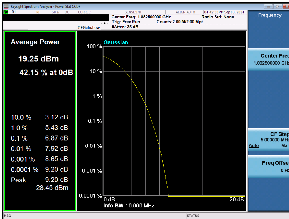
Plot 7-168. PAR Plot (LTE Band 25/2 - 10MHz 256-QAM - Full RB - Ant1)
