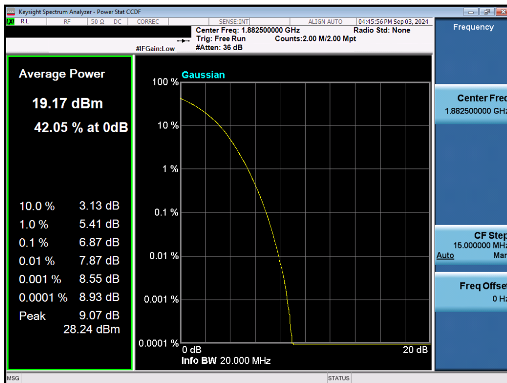
Plot 7-164. PAR Plot (LTE Band 25/2 - 20MHz 256-QAM - Full RB - Ant1)
