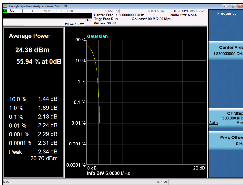
Plot 7-162. PAR Plot (WCDMA, Ch. 9400 - Ant1)
