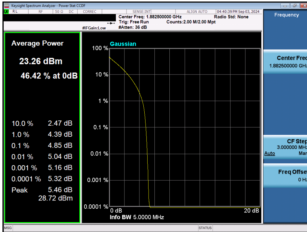
Plot 7-169. PAR Plot (LTE Band 25/2 - 5MHz QPSK - Full RB - Ant1)
