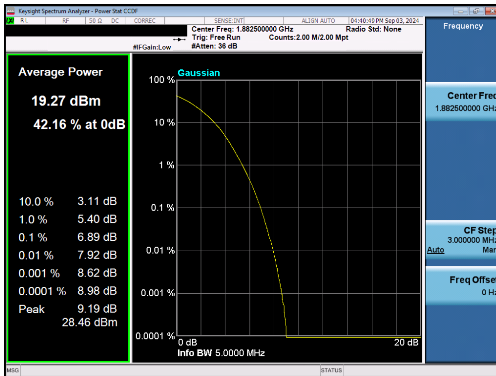
Plot 7-170. PAR Plot (LTE Band 25/2 - 5MHz 256-QAM - Full RB - Ant1)
