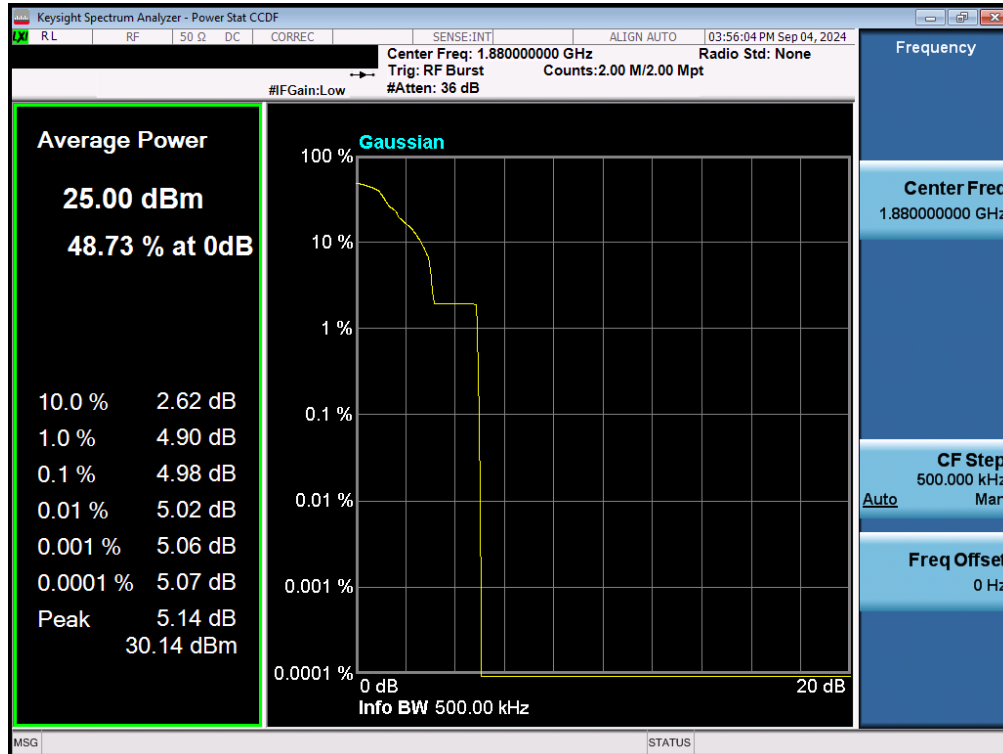
Plot 7-161. PAR Plot (EDGE, Ch. 661 - Ant1)
