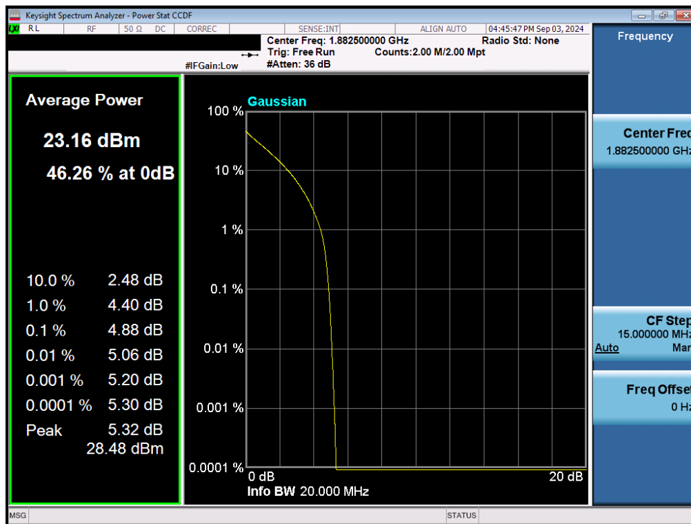
Plot 7-163. PAR Plot (LTE Band 25/2 - 20MHz QPSK - Full RB - Ant1)
