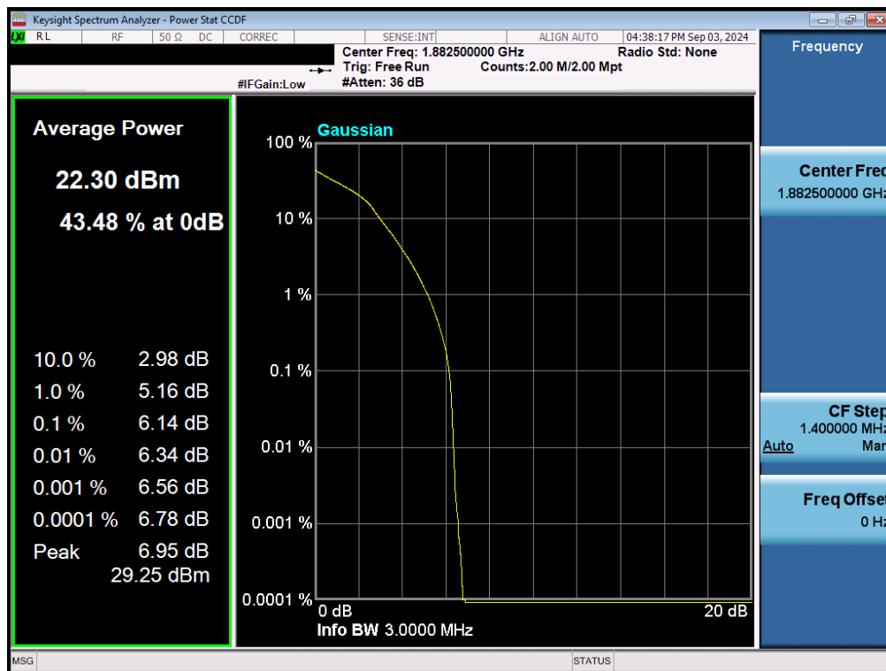
Plot 7-172. PAR Plot (LTE Band 25/2 - 3MHz 16-QAM - Full RB - Ant1)
