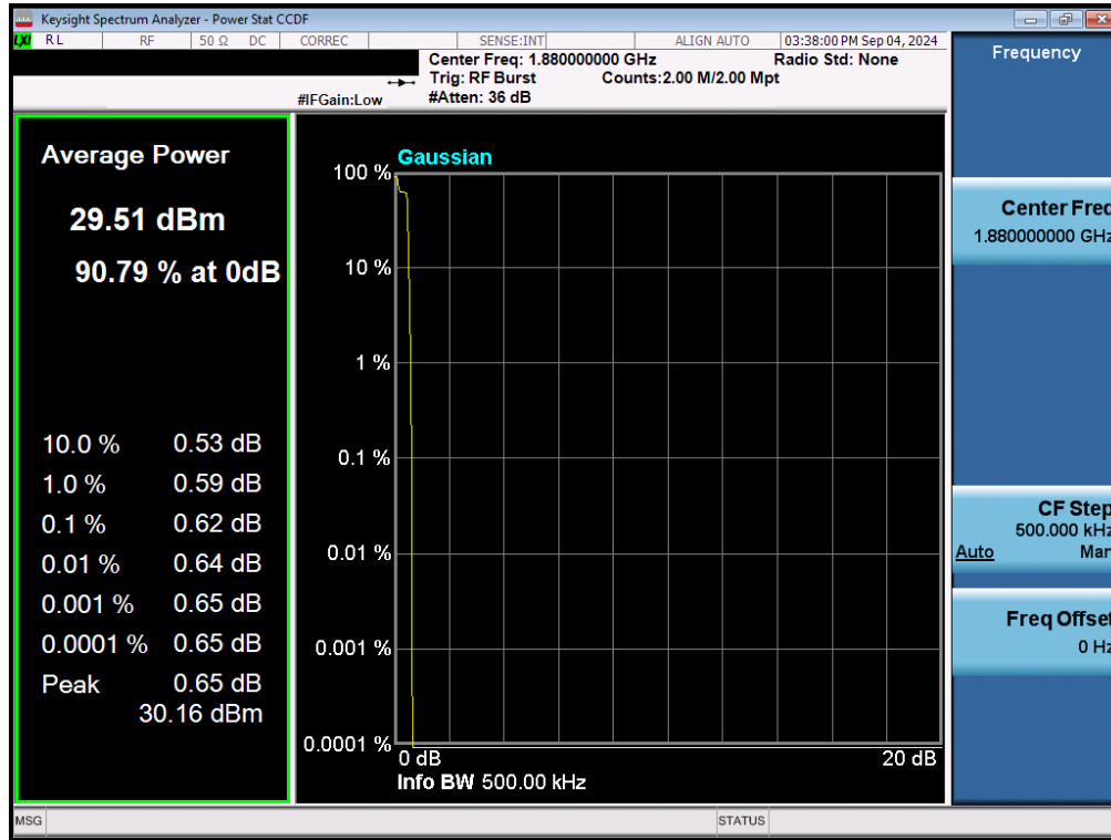
Plot 7-160. PAR Plot (GPRS, Ch. 661 - Ant1)
