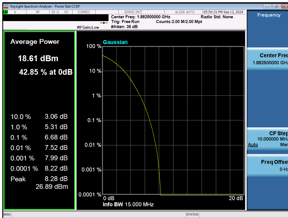
Plot 7-164. PAR Plot (LTE Band 25/2 - 15MHz 256-QAM - Full RB - Ant1)
