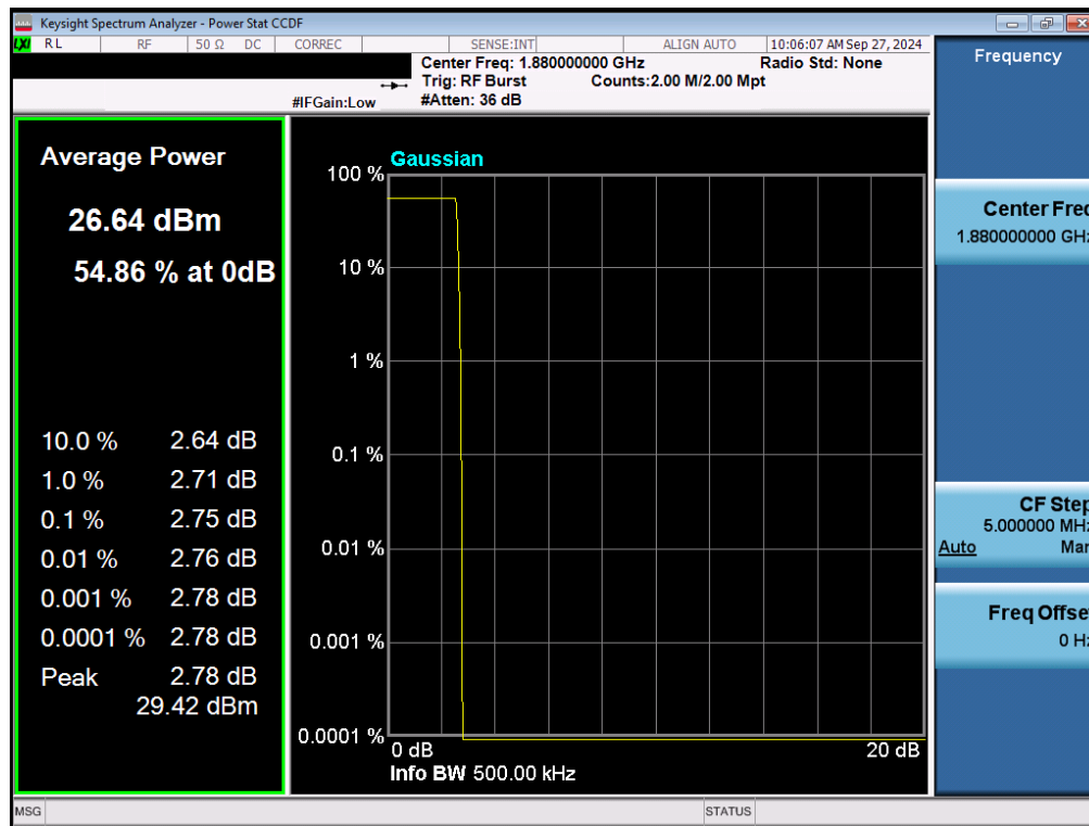
Plot 7-158. PAR Plot (GPRS, Ch. 661 - Ant1)
