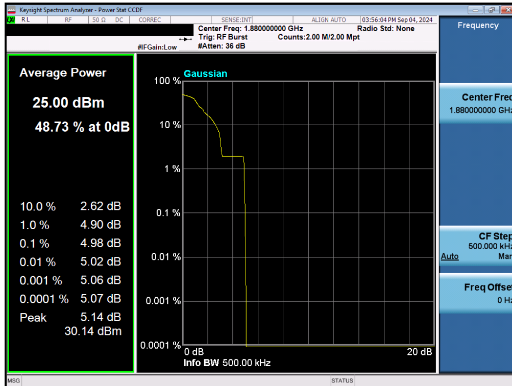
Plot 7-159. PAR Plot (EDGE, Ch. 661 - Ant1)
