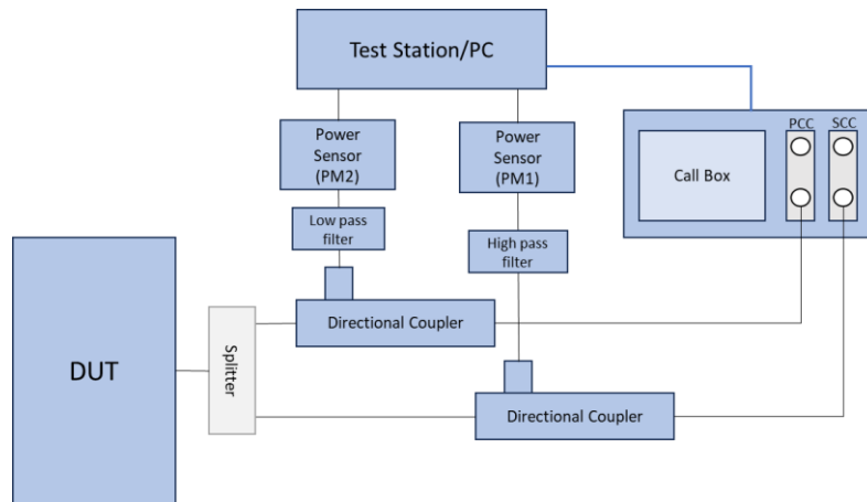
(d) Appendix A – Test Setup Photo 6
