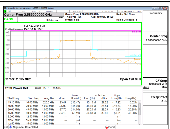
5G NR N38 30MHz BPSK Low Channel RB75-0
