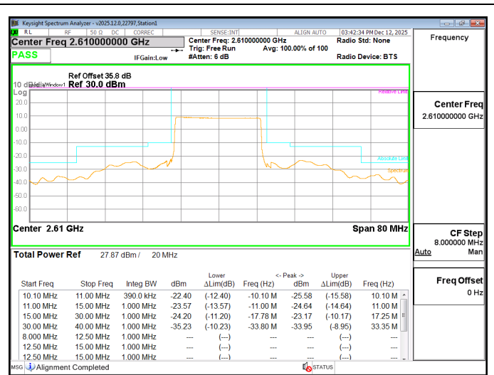
5G NR N38 20MHz BPSK High Channel RB50-0
