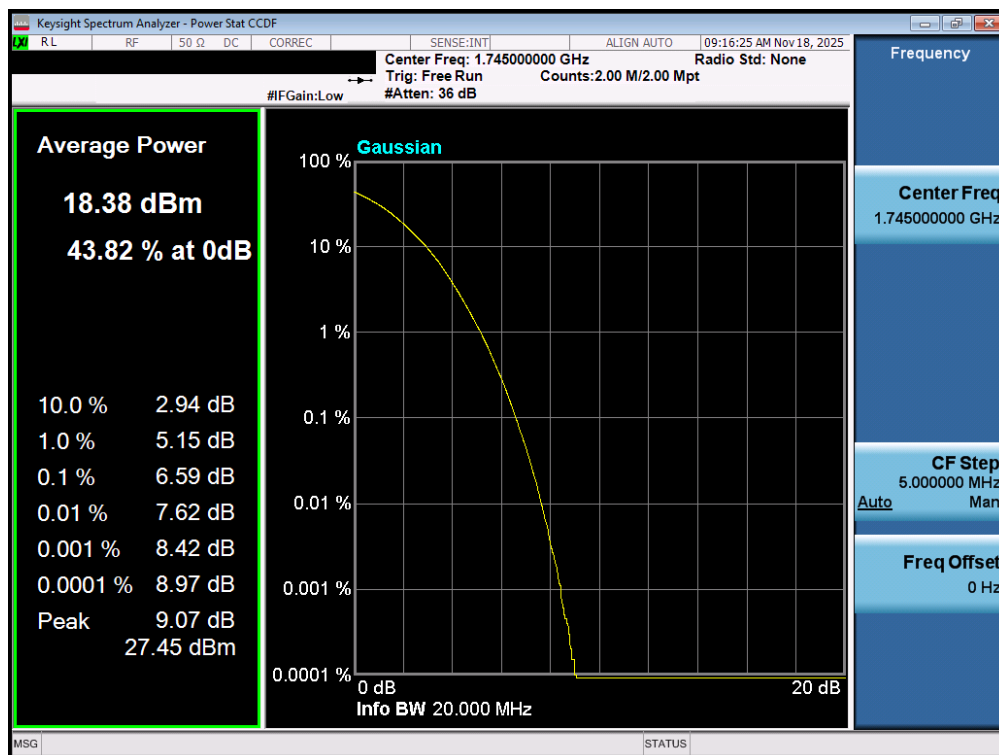
Plot 7-198. PAR Plot (LTE Band 66/4 - 20MHz 256-QAM - Full RB - ANT1)
