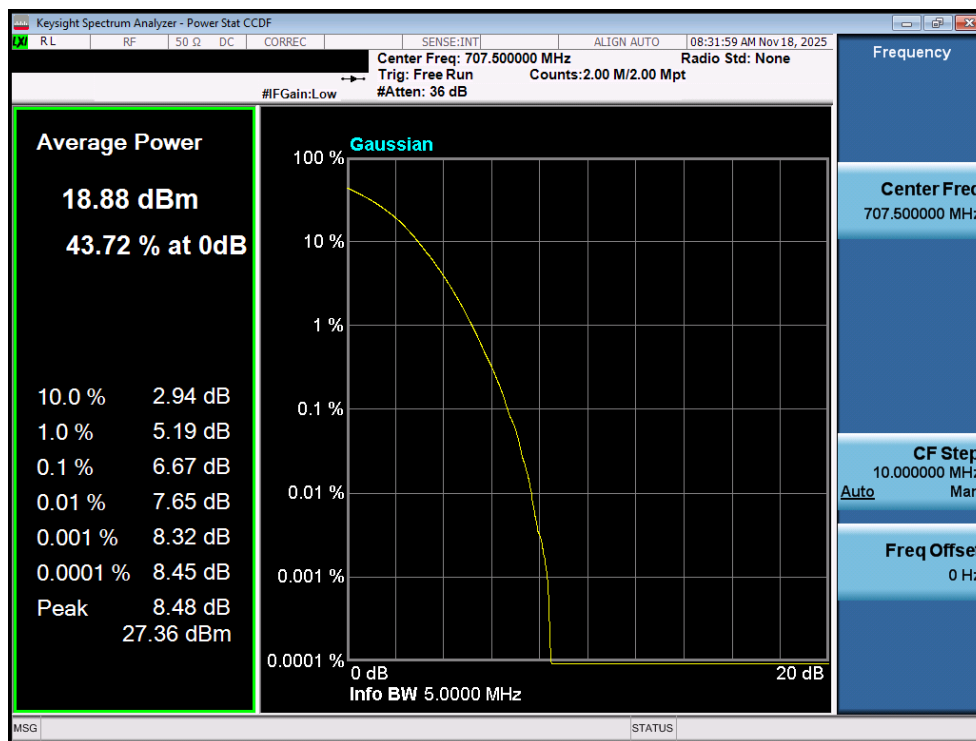
Plot 7-193. PAR Plot (LTE Band 12/17 - 5MHz 256-QAM - Full RB - ANT1)
