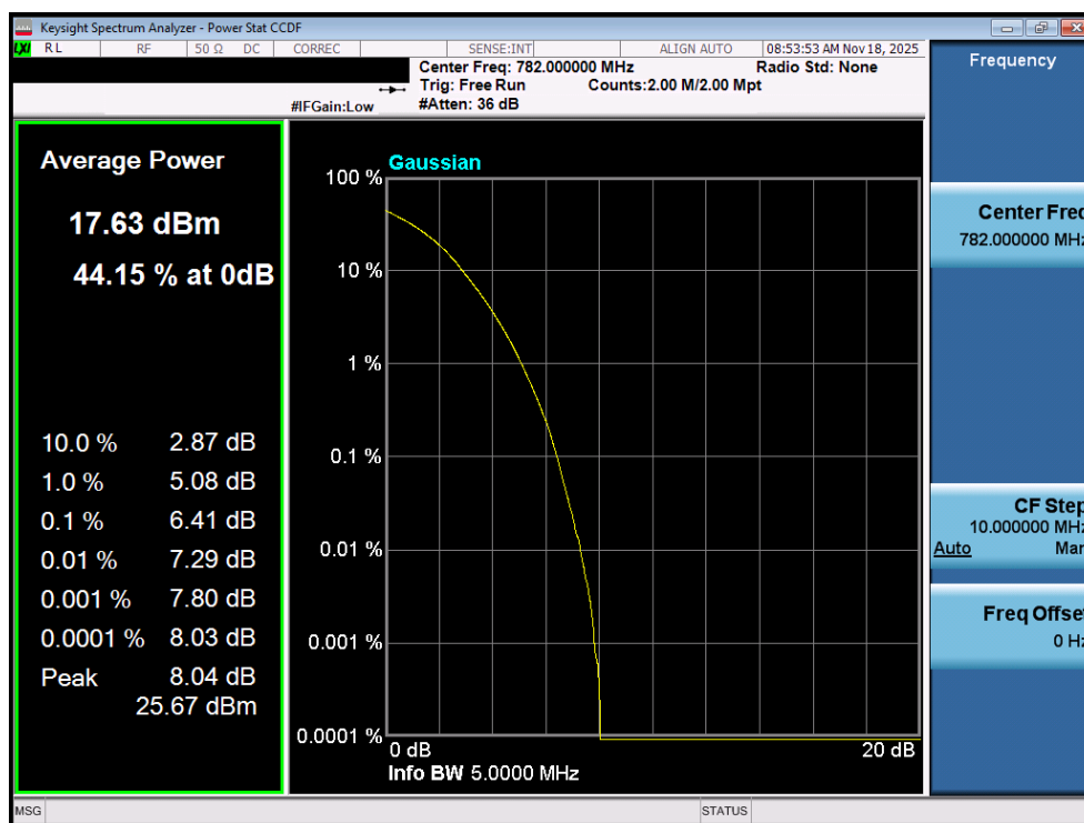
Plot 7-197. PAR Plot (LTE Band 13 - 5MHz 256-QAM - Full RB - ANT1)
