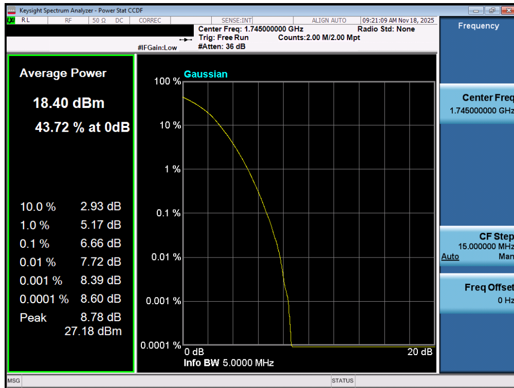
Plot 7-201. PAR Plot (LTE Band 66/4 - 5MHz 256-QAM - Full RB - ANT1)
