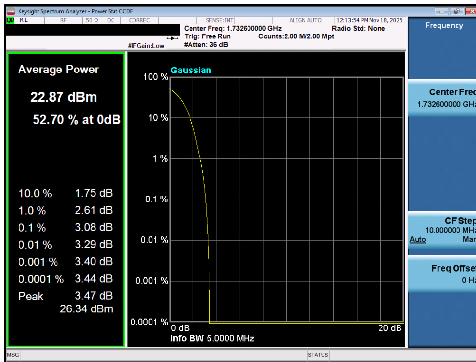
Plot 7-191. PAR Plot (WCDMA, Ch. 1413 – ANT1)
