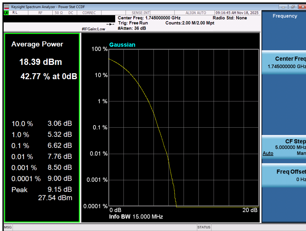
Plot 7-199. PAR Plot (LTE Band 66/4 - 15MHz 256-QAM - Full RB - ANT1)
