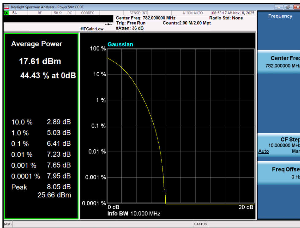
Plot 7-196. PAR Plot (LTE Band 13 - 10MHz 256-QAM - Full RB - ANT1)
