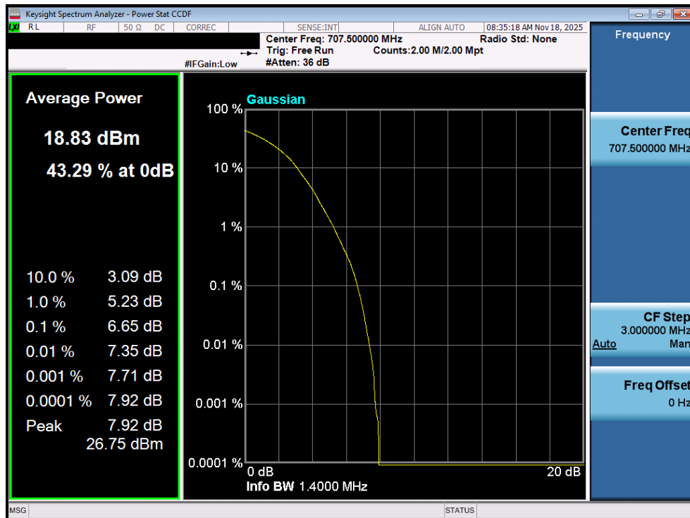
Plot 7-195. PAR Plot (LTE Band 12 - 1.4MHz 256-QAM - Full RB - ANT1)
