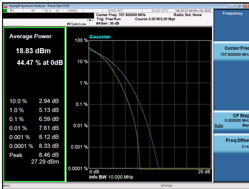
Plot 7-192. PAR Plot (LTE Band 12/17 - 10MHz 256-QAM - Full RB - ANT1)
