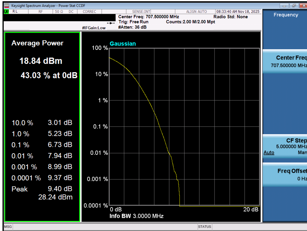
Plot 7-194. PAR Plot (LTE Band 12 - 3MHz 256-QAM - Full RB - ANT1)
