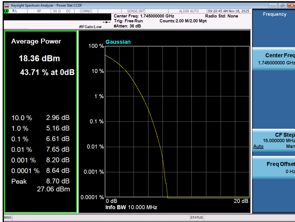
Plot 7-200. PAR Plot (LTE Band 66/4 - 10MHz 256-QAM - Full RB - ANT1)
