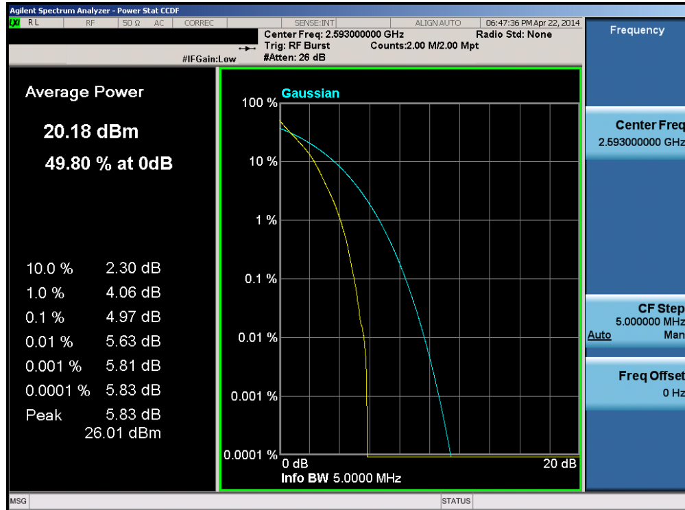
Plot 6-40. PAR Plot (Band 41 – 5.0MHz QPSK – RB Size 25)
