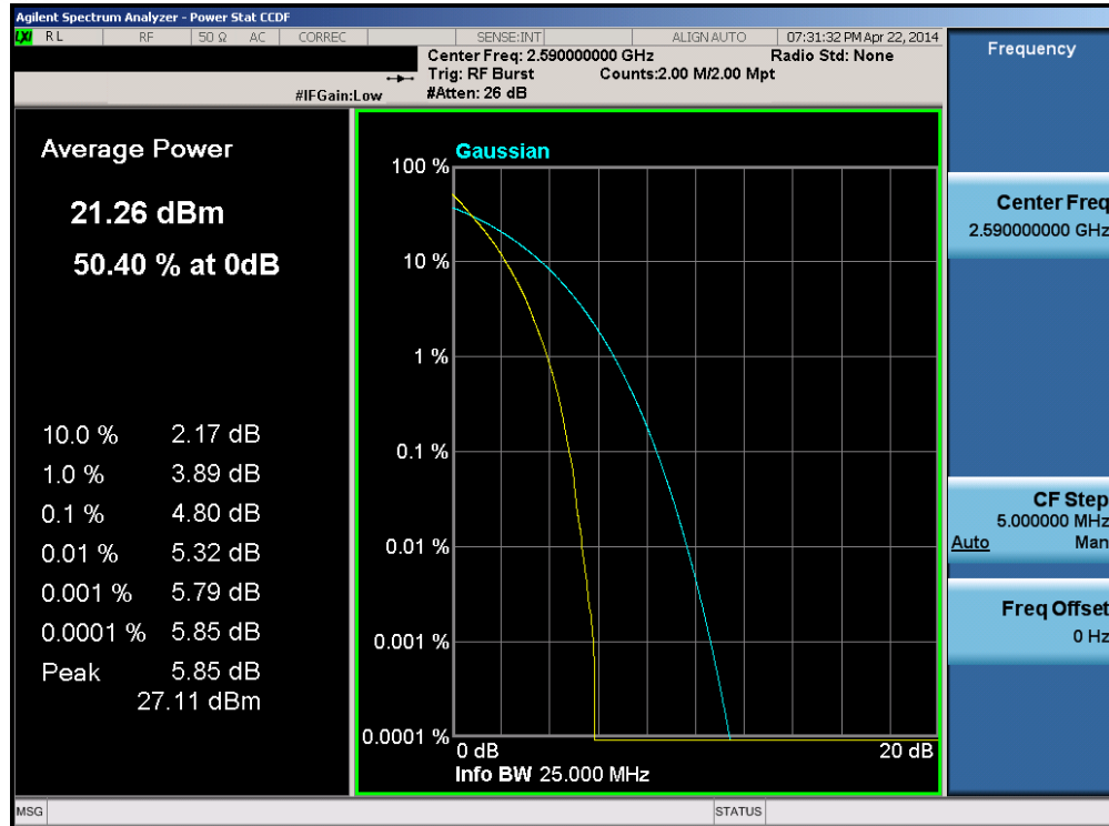
Plot 6-46. PAR Plot (Band 41 – 20.0MHz QPSK – RB Size 100)
