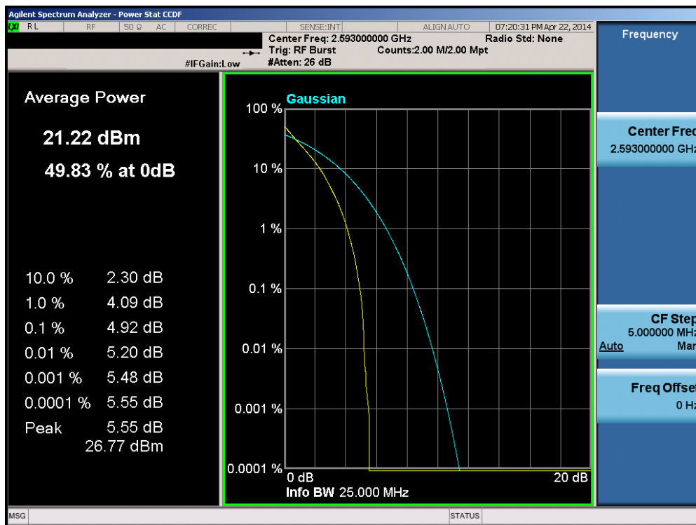
Plot 6-44. PAR Plot (Band 41 – 15.0MHz QPSK – RB Size 75)
