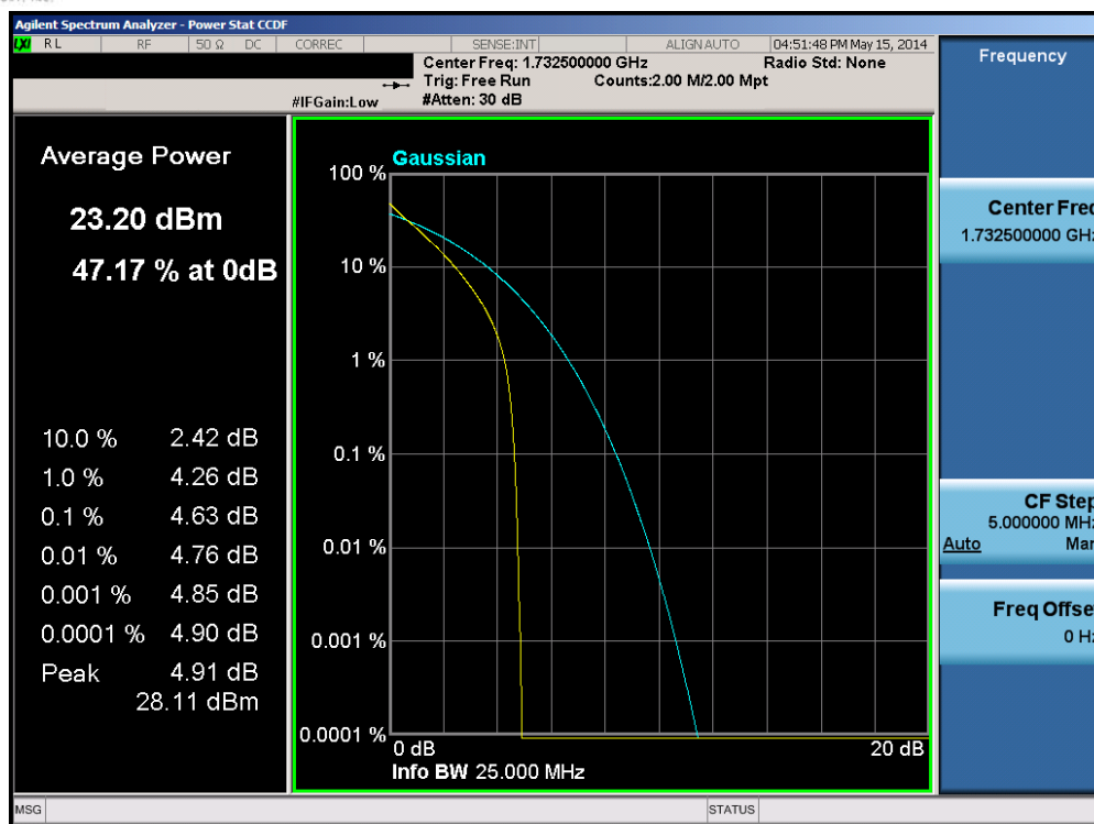
Plot 6-137. PAR Plot (Band 4 – 15.0MHz QPSK – RB Size 75)
