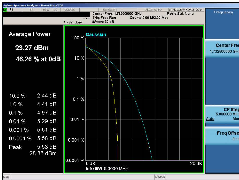
Plot 6-133. PAR Plot (Band 4 – 5.0MHz QPSK – RB Size 25)
