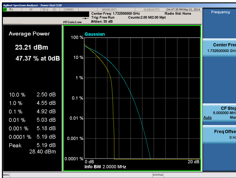
Plot 6-129. PAR Plot (Band 4 – 1.4MHz QPSK – RB Size 6)
