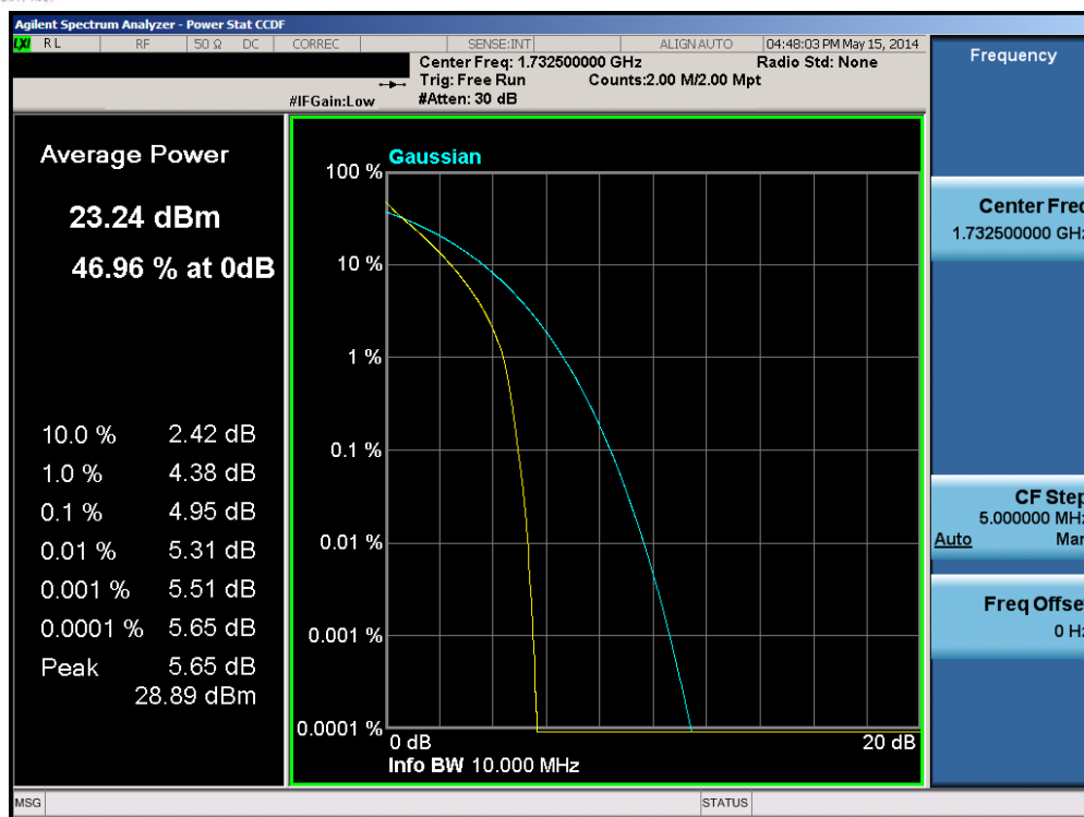
Plot 6-135. PAR Plot (Band 4 – 10.0MHz QPSK – RB Size 50)
