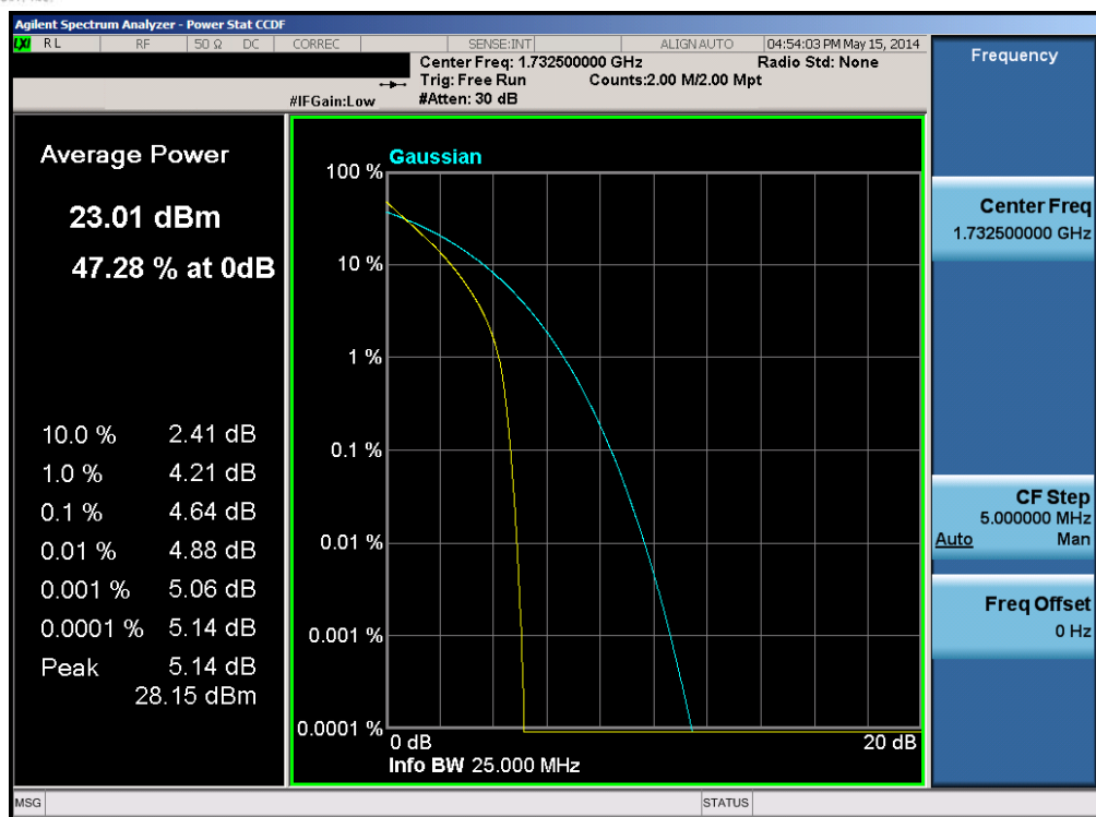
Plot 6-139. PAR Plot (Band 4 – 20.0MHz QPSK – RB Size 100)
