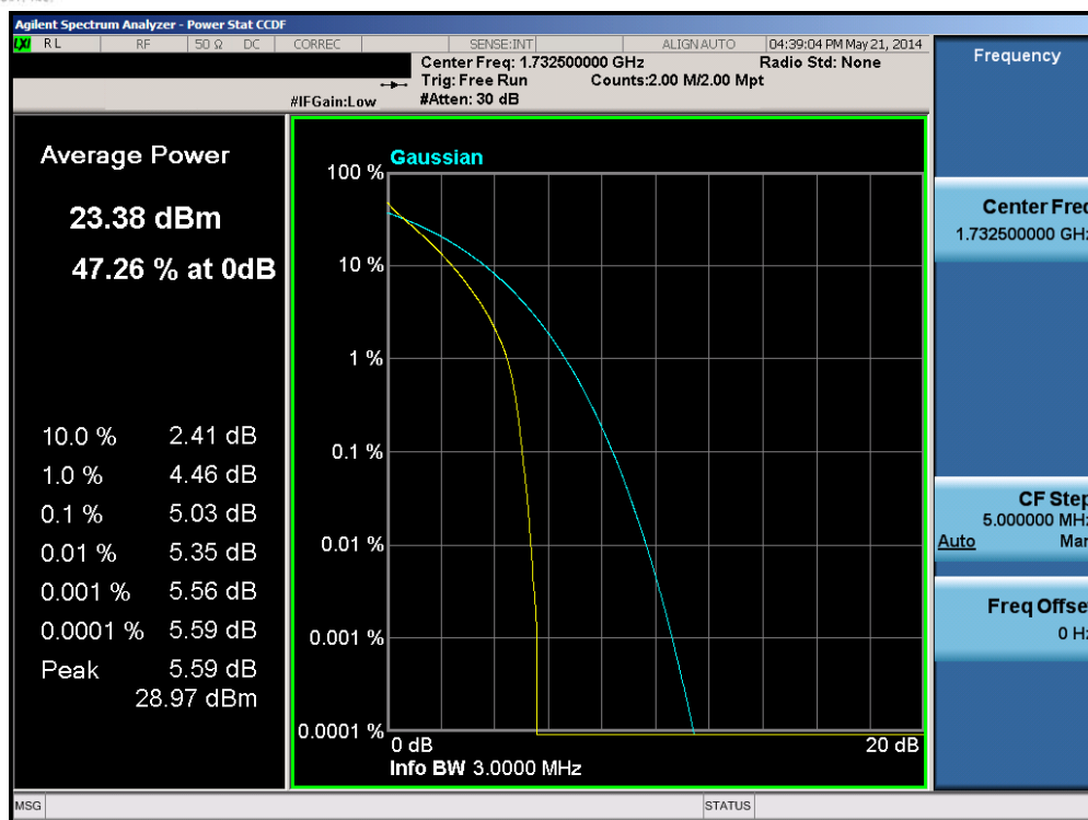
Plot 6-131. PAR Plot (Band 4 – 3.0MHz QPSK – RB Size 15)
