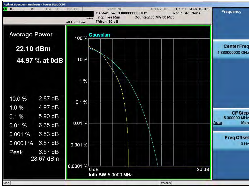
Plot 6-115. PAR Plot (Band 2 – 5.0MHz 16-QAM – RB Size 25)
