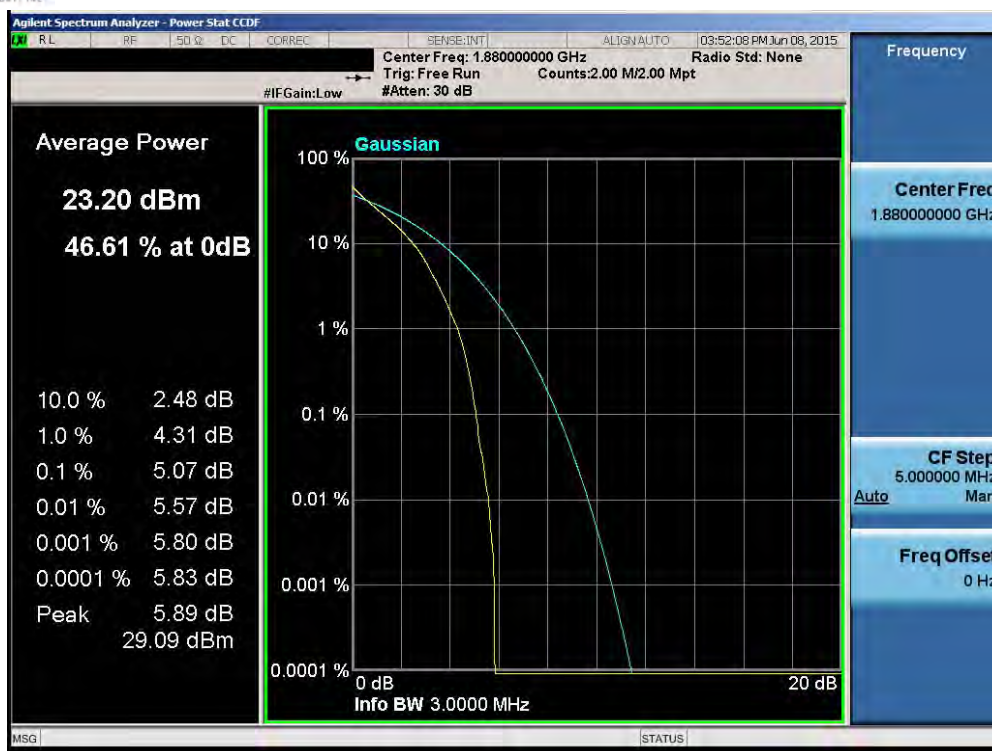
Plot 6-112. PAR Plot (Band 2 – 3.0MHz QPSK – RB Size 15)
