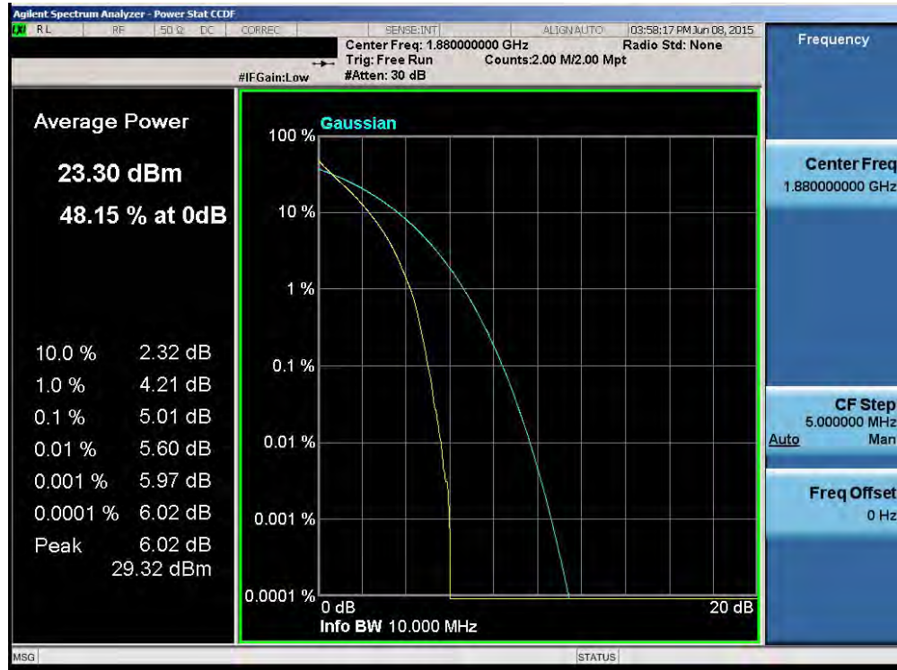
Plot 6-116. PAR Plot (Band 2 – 10.0MHz QPSK – RB Size 50)
