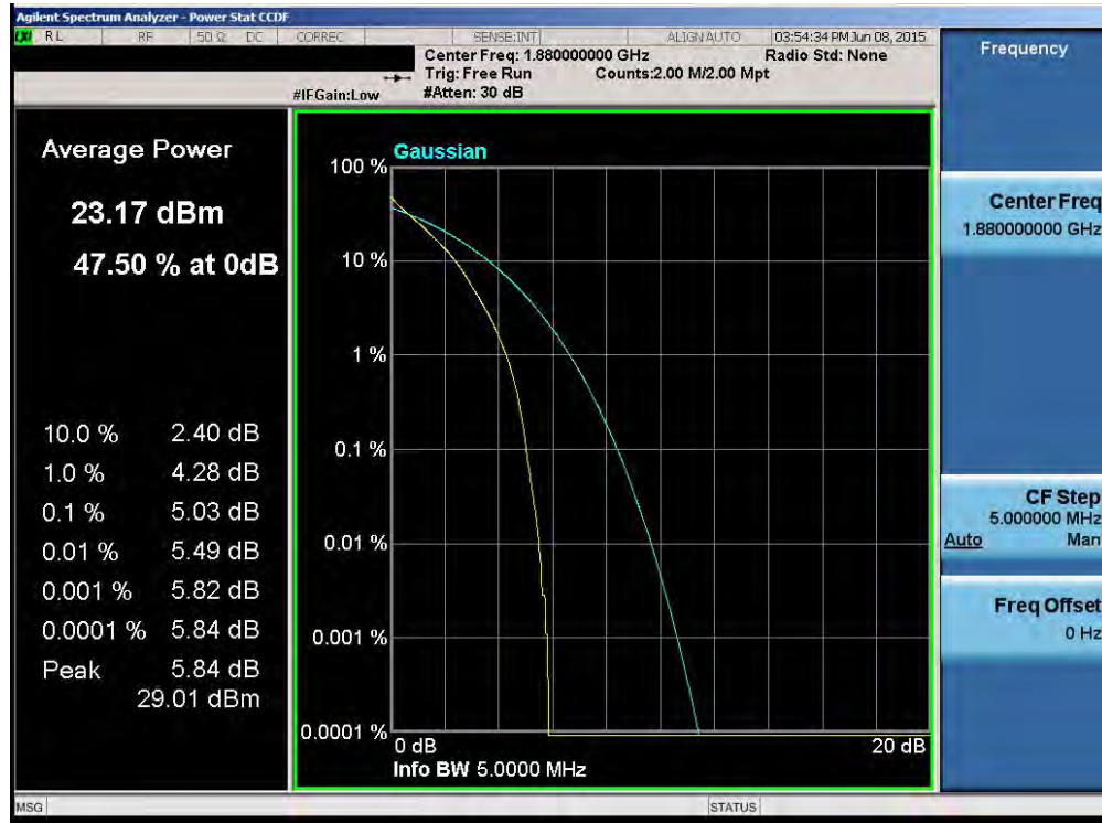
Plot 6-114. PAR Plot (Band 2 – 5.0MHz QPSK – RB Size 25)
