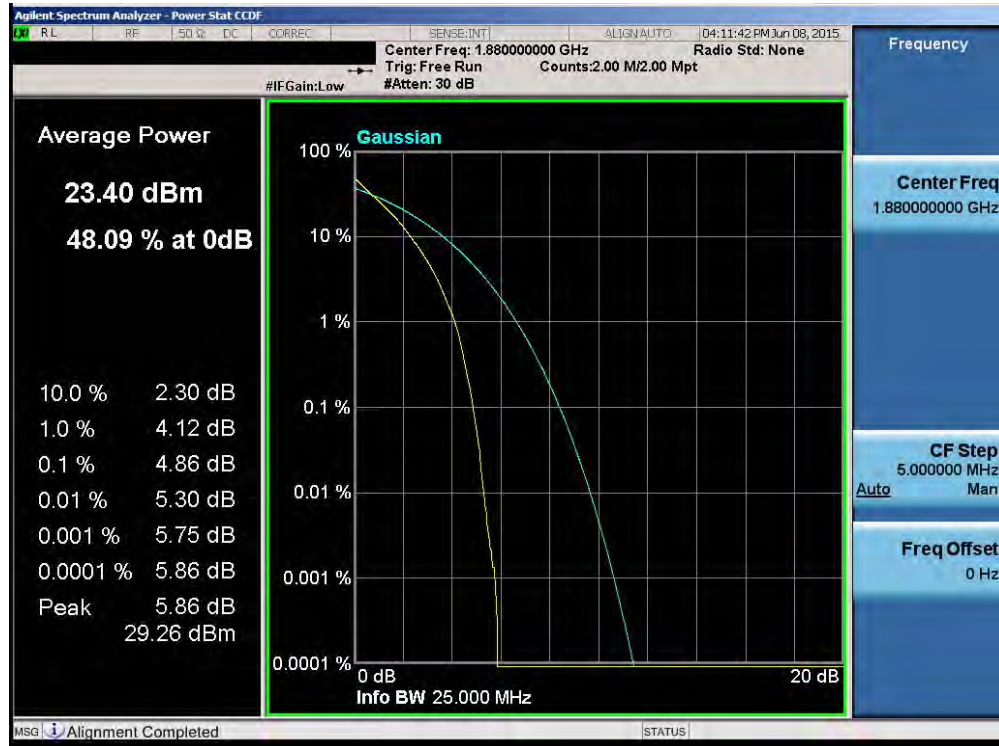
Plot 6-120. PAR Plot (Band 2 – 20.0MHz QPSK – RB Size 100)
