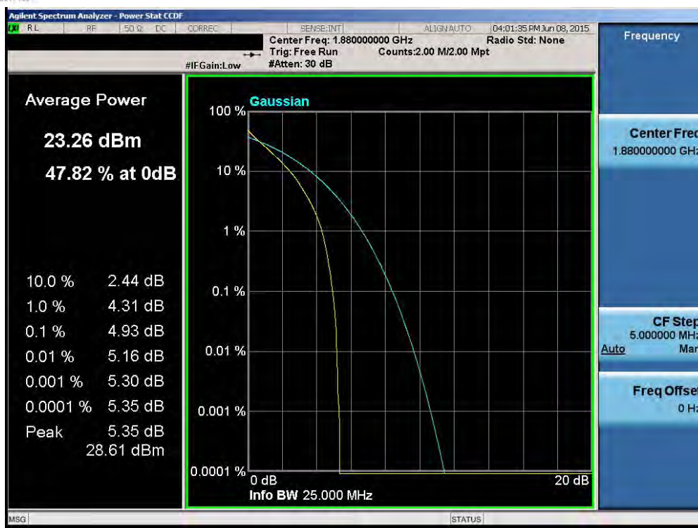
Plot 6-118. PAR Plot (Band 2 – 15.0MHz QPSK – RB Size 75)
