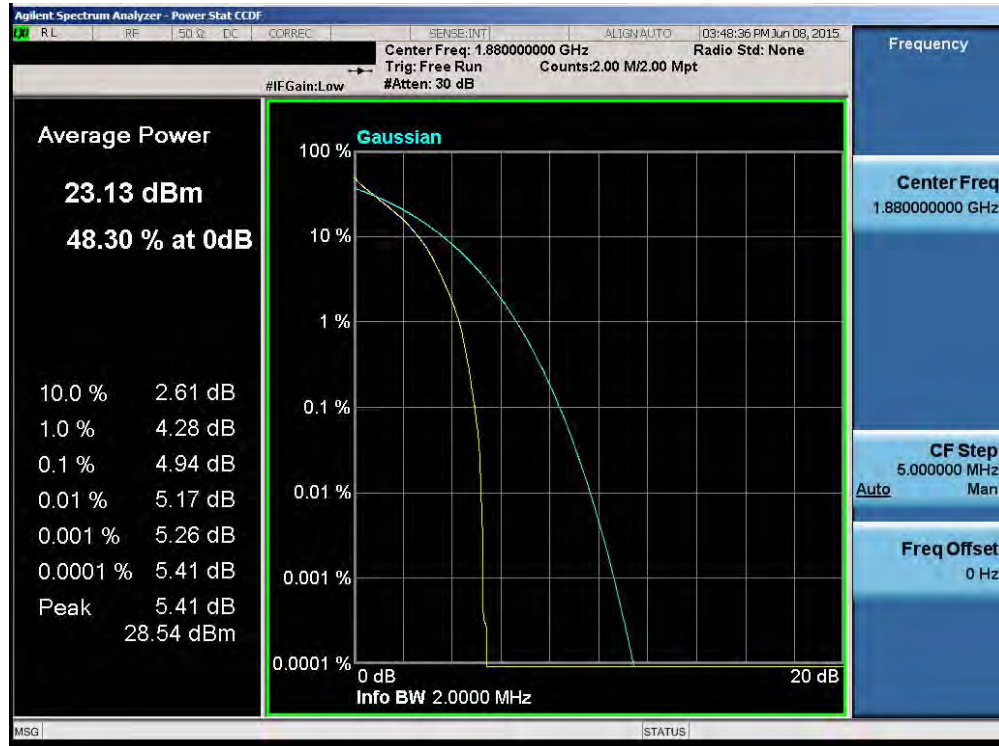
Plot 6-110. PAR Plot (Band 2 – 1.4MHz QPSK – RB Size 6)
