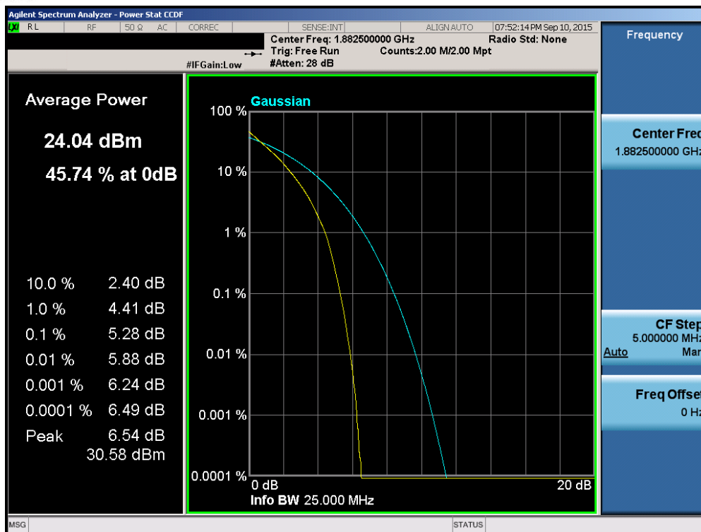
Plot 6-194. PAR Plot (Band 2/25 – 20.0MHz QPSK – RB Size 100)
