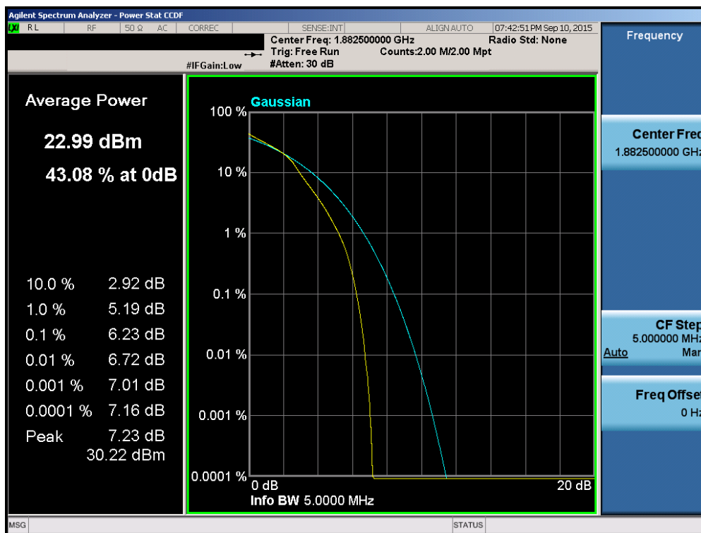
Plot 6-189. PAR Plot (Band 2/25 – 5.0MHz 16-QAM – RB Size 25)
