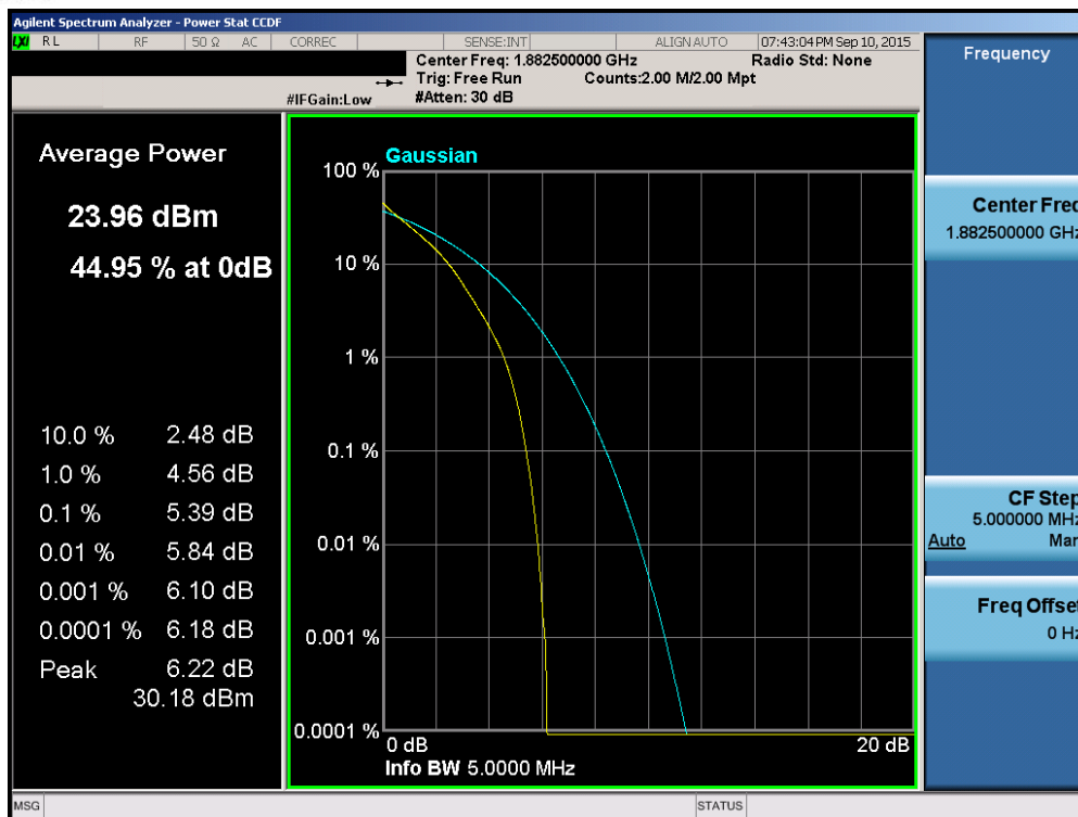
Plot 6-188. PAR Plot (Band 2/25 – 5.0MHz QPSK – RB Size 25)
