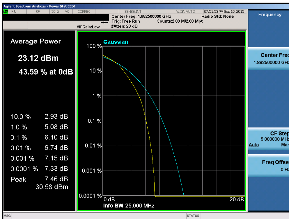
Plot 6-195. PAR Plot (Band 2/25 – 20.0MHz 16-QAM – RB Size 100)
