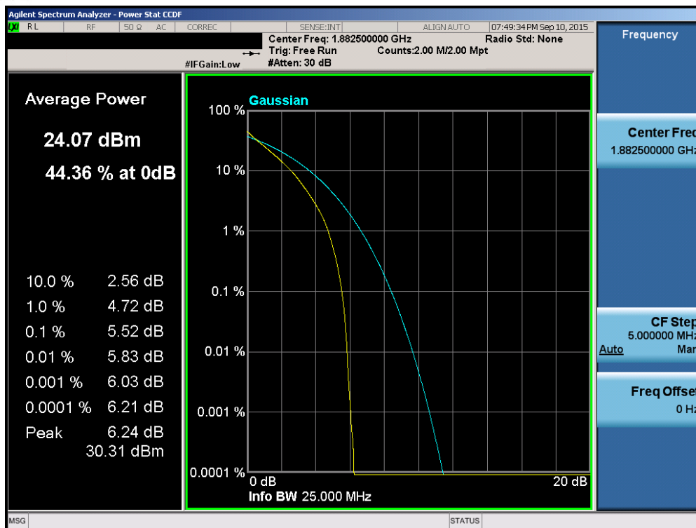
Plot 6-161. PAR Plot (Band 2/25 – 15.0MHz QPSK – RB Size 75)
