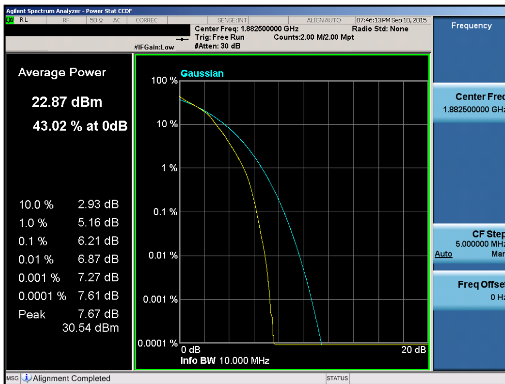
Plot 6-160. PAR Plot (Band 2/25 – 10.0MHz 16-QAM – RB Size 50)
