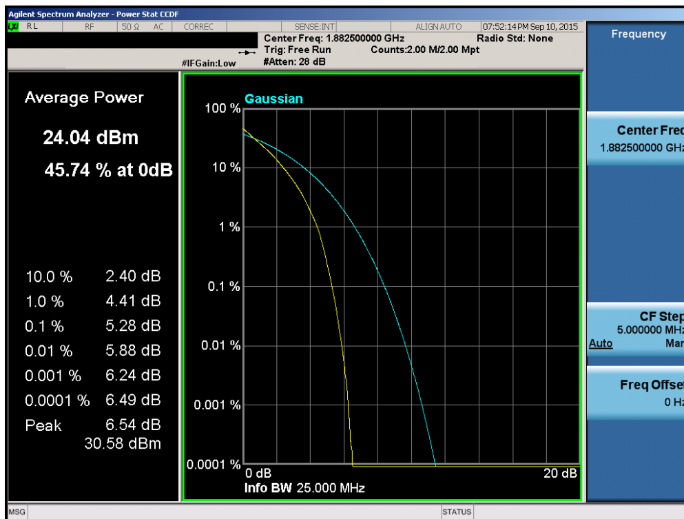
Plot 6-163. PAR Plot (Band 2/25 – 20.0MHz QPSK – RB Size 100)
