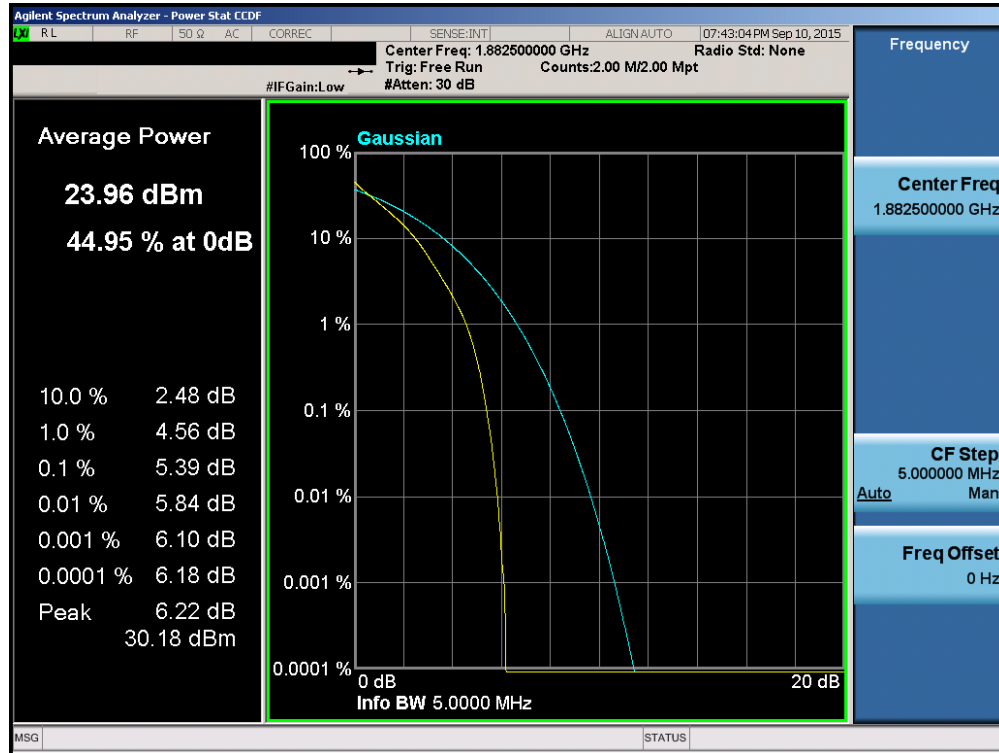
Plot 6-157. PAR Plot (Band 2/25 – 5.0MHz QPSK – RB Size 25)
