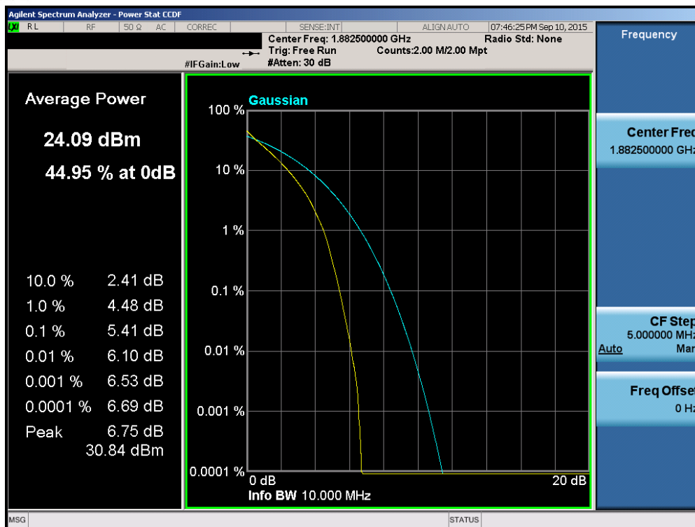
Plot 6-159. PAR Plot (Band 2/25 – 10.0MHz QPSK – RB Size 50)
