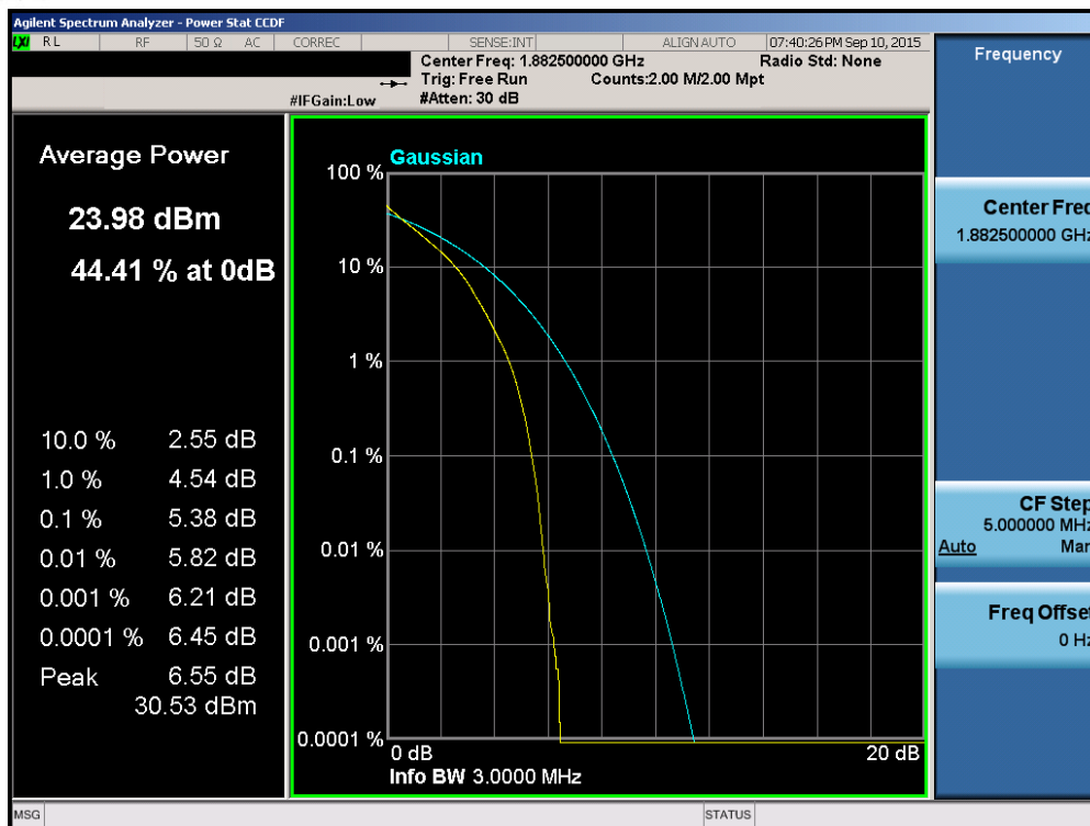
Plot 6-155. PAR Plot (Band 2/25 – 3.0MHz QPSK – RB Size 15)
