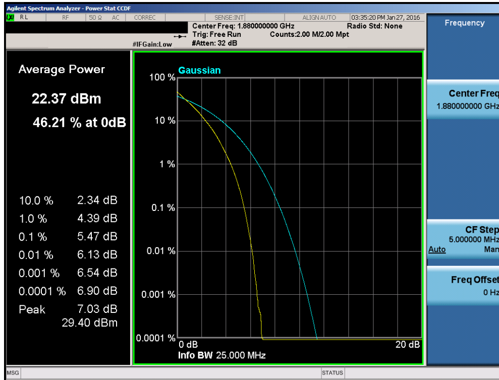
Plot 7-126. PAR Plot (Band 2 – 20.0MHz QPSK – RB Size 100)
