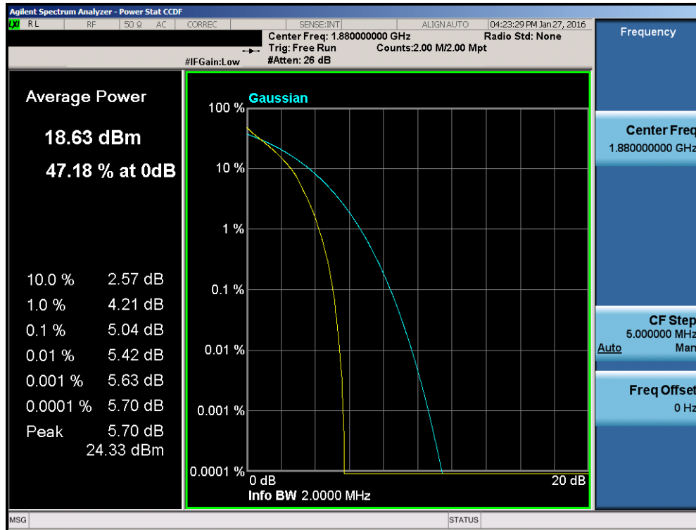
Plot 7-116. PAR Plot (Band 2 – 1.4MHz QPSK – RB Size 6)
