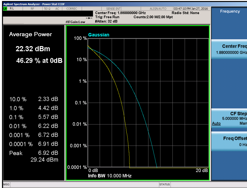
Plot 7-122. PAR Plot (Band 2 – 10.0MHz QPSK – RB Size 50)
