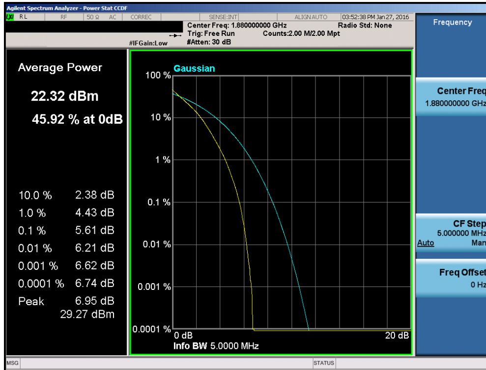
Plot 7-120. PAR Plot (Band 2 – 5.0MHz QPSK – RB Size 25)
