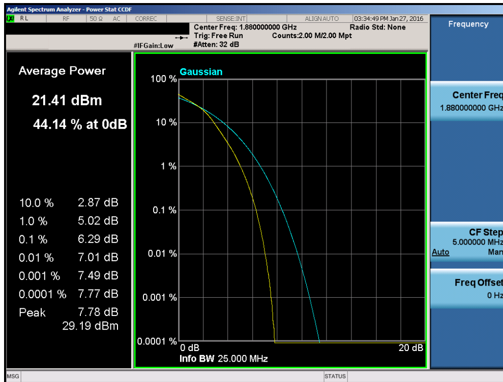
Plot 7-127. PAR Plot (Band 2 – 20.0MHz 16-QAM – RB Size 100)
