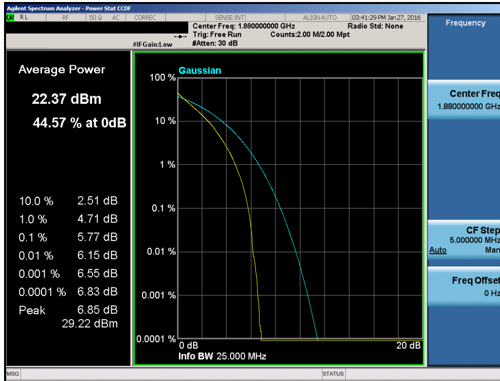
Plot 7-124. PAR Plot (Band 2 – 15.0MHz QPSK – RB Size 75)
