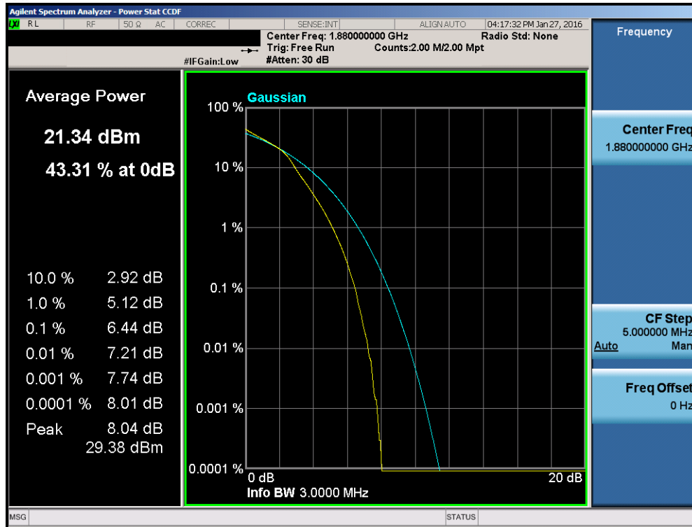
Plot 7-118. PAR Plot (Band 2 – 3.0MHz QPSK – RB Size 15)
