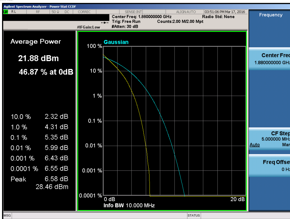
Plot 7-180. PAR Plot (Band 2 – 10.0MHz QPSK – RB Size 50)
