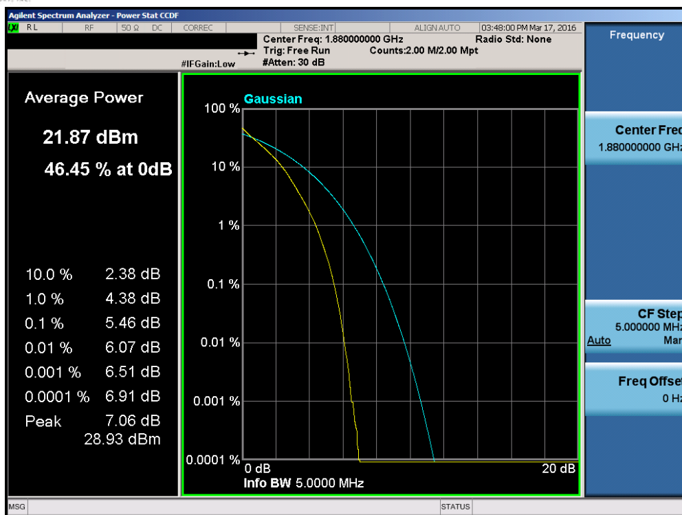
Plot 7-178. PAR Plot (Band 2 – 5.0MHz QPSK – RB Size 25)
