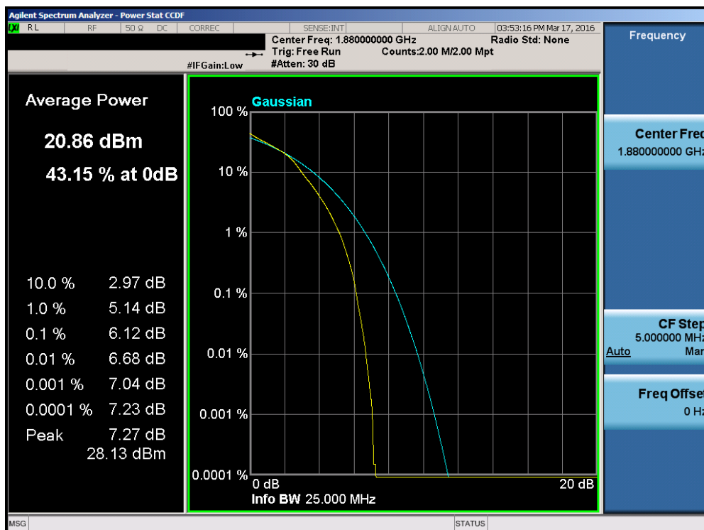
Plot 7-183. PAR Plot (Band 2 – 15.0MHz 16-QAM – RB Size 75)
