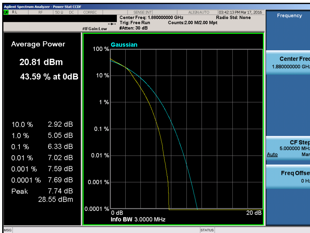
Plot 7-177. PAR Plot (Band 2 - 3.0MHz 16-QAM - RB Size 15)
