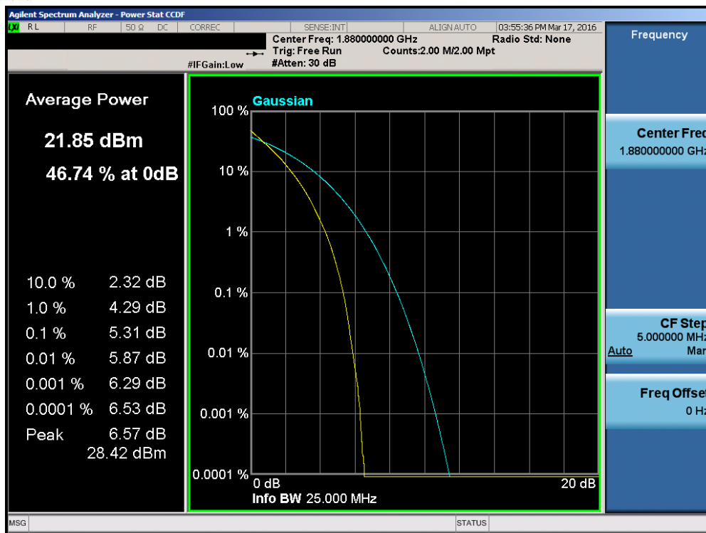
Plot 7-184. PAR Plot (Band 2 – 20.0MHz QPSK – RB Size 100)
