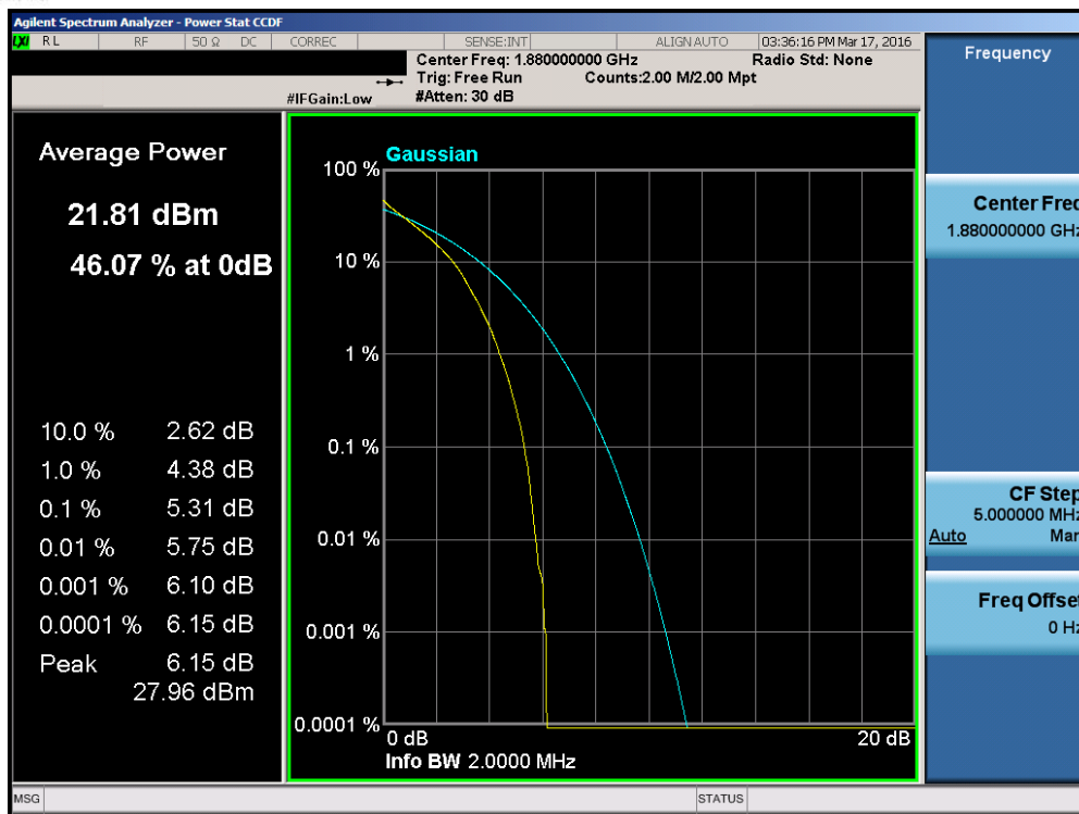
Plot 7-174. PAR Plot (Band 2 – 1.4MHz QPSK – RB Size 6)
