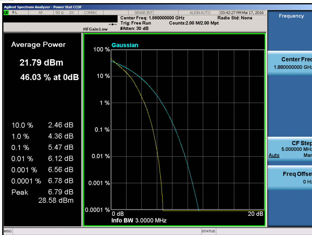
Plot 7-176. PAR Plot (Band 2 - 3.0MHz QPSK - RB Size 15)
