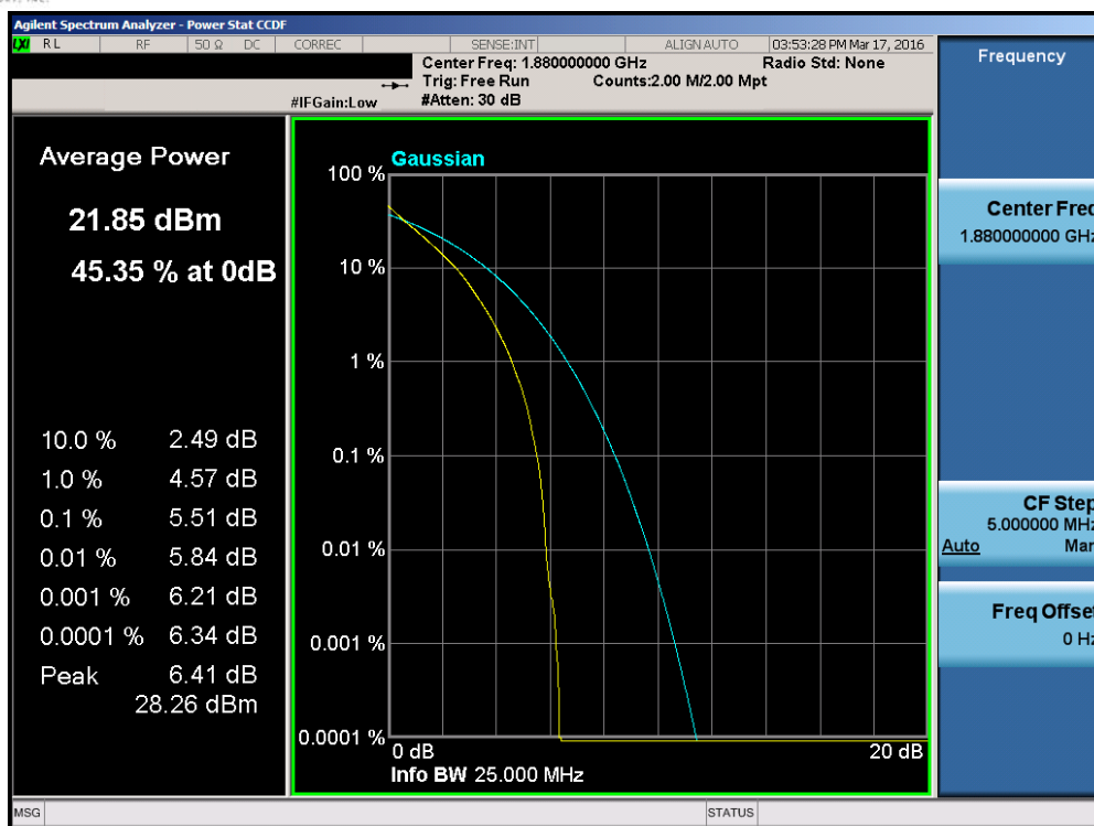
Plot 7-182. PAR Plot (Band 2 – 15.0MHz QPSK – RB Size 75)
