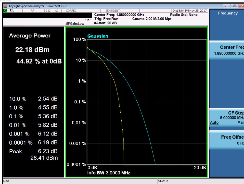
Plot 7-185. PAR Plot (Band 2 – 3.0MHz QPSK – RB Size 15)
