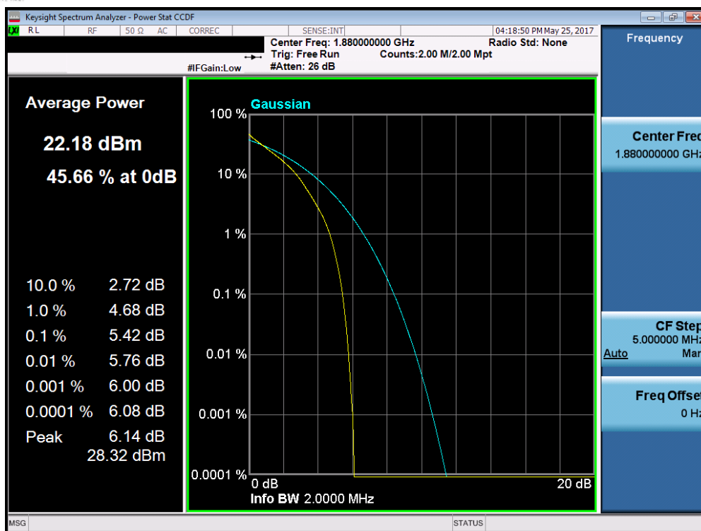
Plot 7-191. PAR Plot (Band 2 – 1.4MHz QPSK – RB Size 6)
