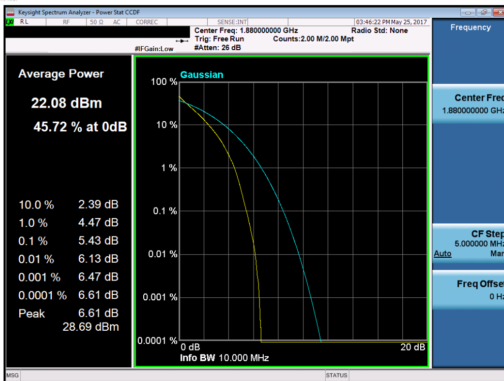
Plot 7-197. PAR Plot (Band 2 – 10.0MHz QPSK – RB Size 50)
