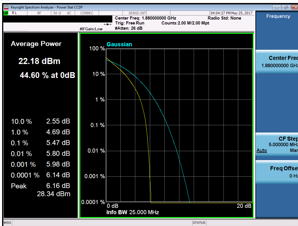
Plot 7-199. PAR Plot (Band 2 – 15.0MHz QPSK – RB Size 75)
