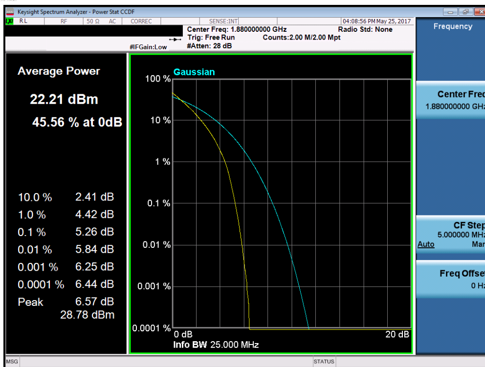
Plot 7-201. PAR Plot (Band 2 – 20.0MHz QPSK – RB Size 100)
