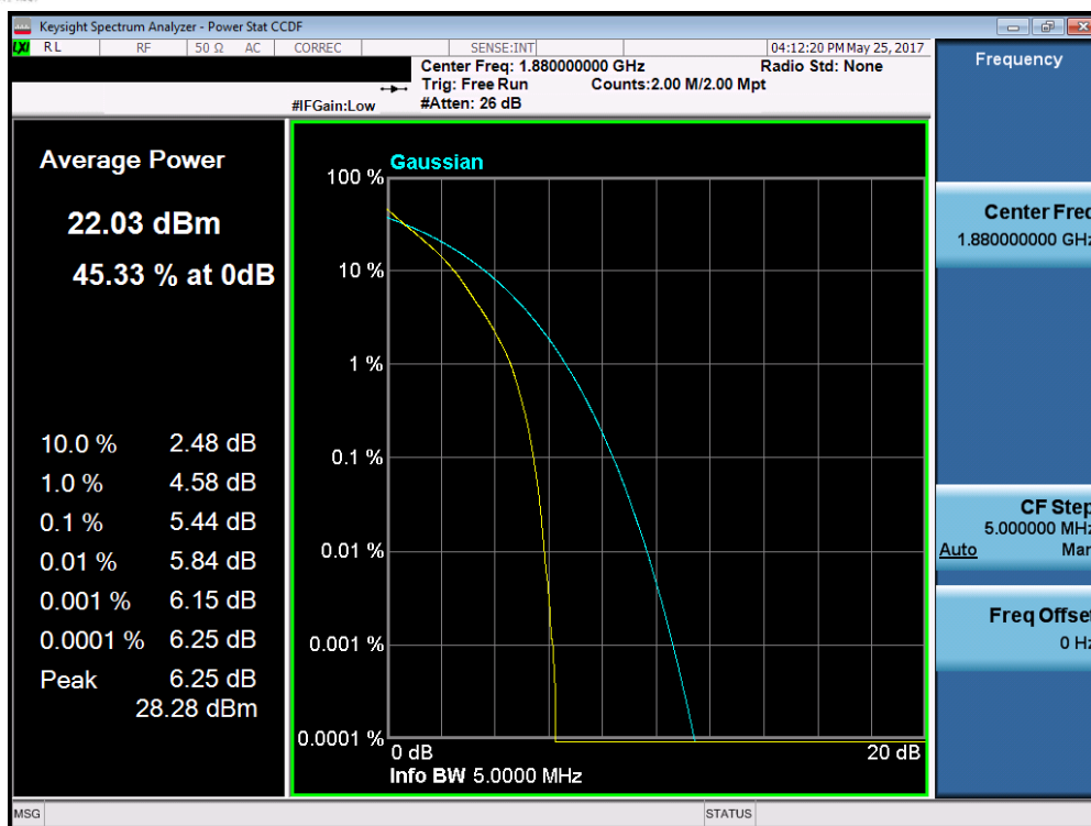
Plot 7-195. PAR Plot (Band 2 – 5.0MHz QPSK – RB Size 25)
