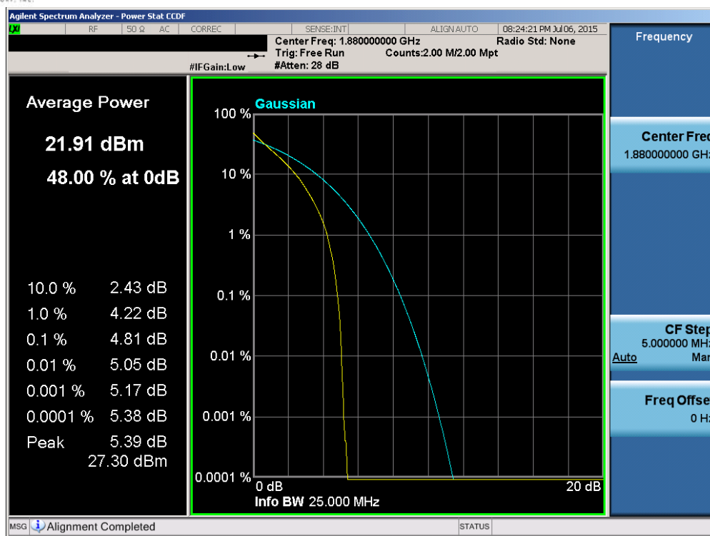
Plot 6-120. PAR Plot (Band 2 – 15.0MHz QPSK – RB Size 75)
