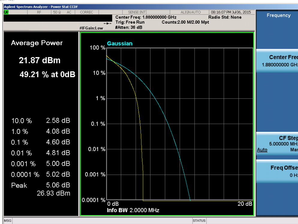
Plot 6-112. PAR Plot (Band 2 – 1.4MHz QPSK – RB Size 6)
