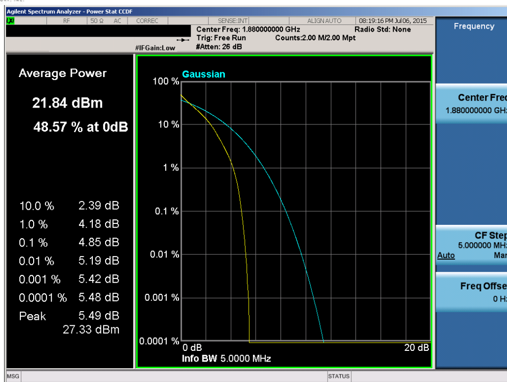
Plot 6-116. PAR Plot (Band 2 – 5.0MHz QPSK – RB Size 25)
