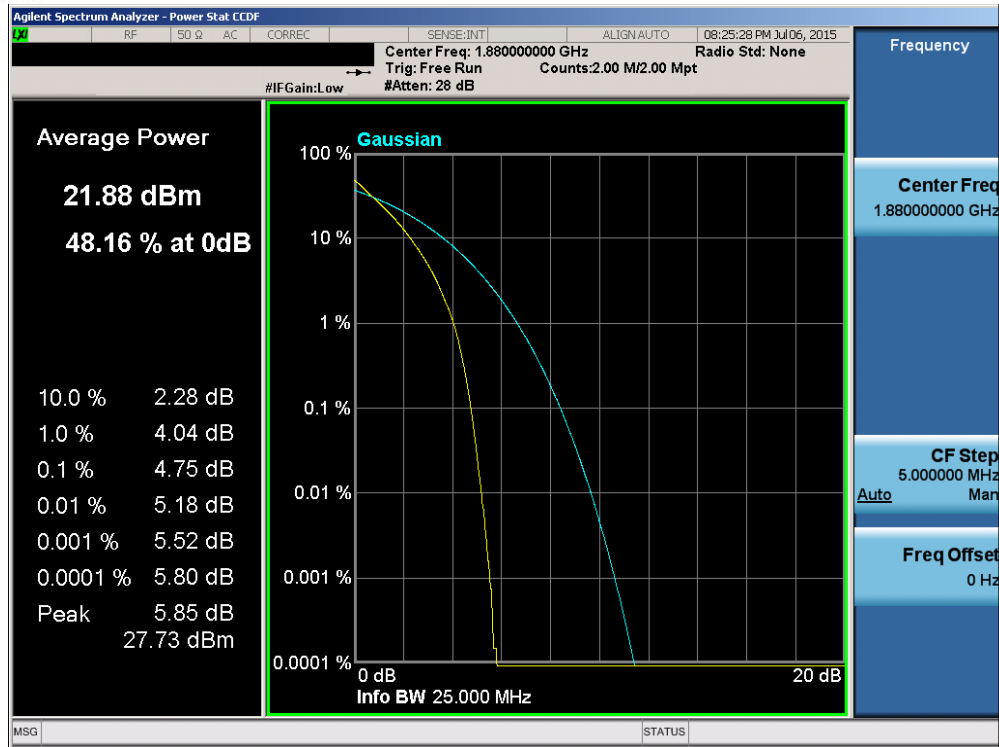
Plot 6-122. PAR Plot (Band 2 – 20.0MHz QPSK – RB Size 100)
