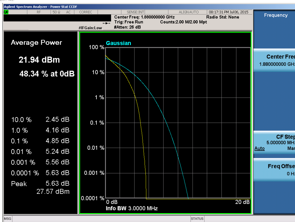
Plot 6-114. PAR Plot (Band 2 – 3.0MHz QPSK – RB Size 15)
