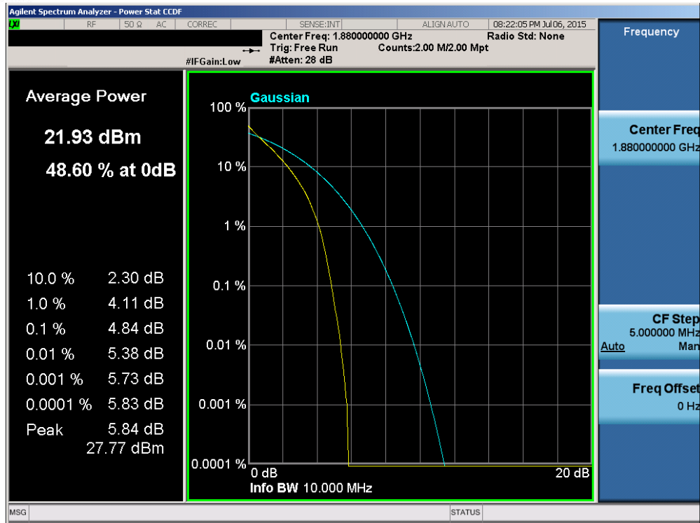
Plot 6-118. PAR Plot (Band 2 – 10.0MHz QPSK – RB Size 50)
