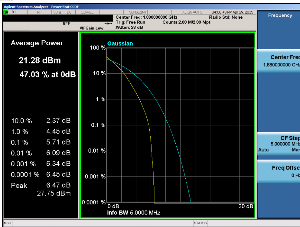
Plot 6-174. PAR Plot (Band 2 – 5.0MHz QPSK – RB Size 25)
