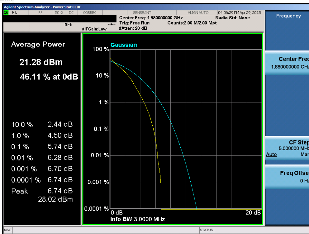
Plot 6-172. PAR Plot (Band 2 – 3.0MHz QPSK – RB Size 15)
