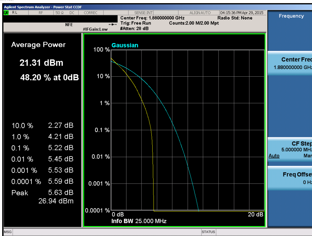
Plot 6-180. PAR Plot (Band 2 – 20.0MHz QPSK – RB Size 100)
