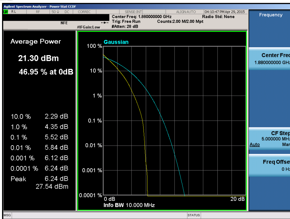
Plot 6-176. PAR Plot (Band 2 – 10.0MHz QPSK – RB Size 50)
