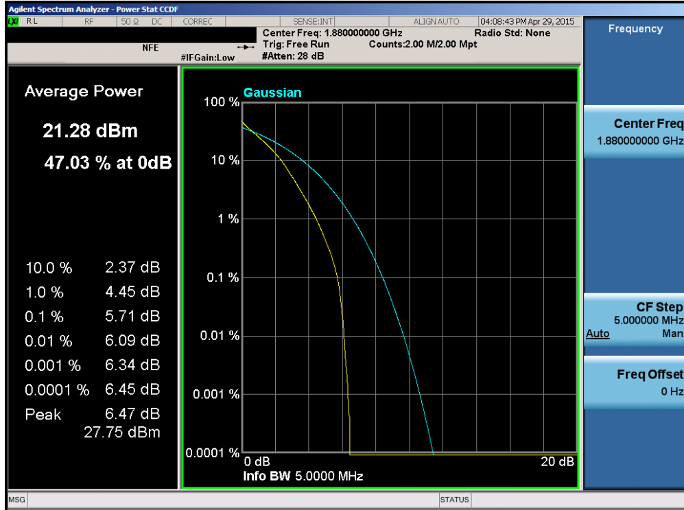
Plot 6-147. PAR Plot (Band 2 – 5.0MHz QPSK – RB Size 25)
