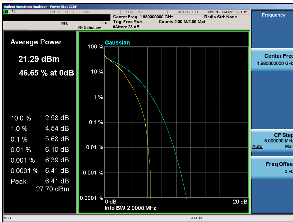
Plot 6-143. PAR Plot (Band 2 – 1.4MHz QPSK – RB Size 6)
