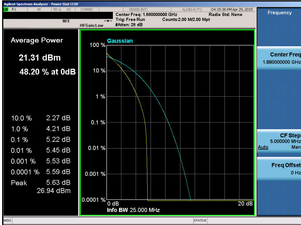
Plot 6-153. PAR Plot (Band 2 – 20.0MHz QPSK – RB Size 100)
