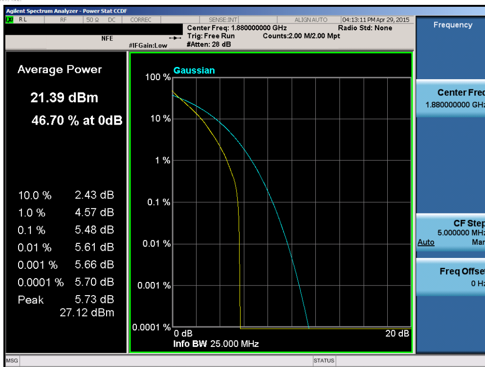
Plot 6-151. PAR Plot (Band 2 – 15.0MHz QPSK – RB Size 75)
