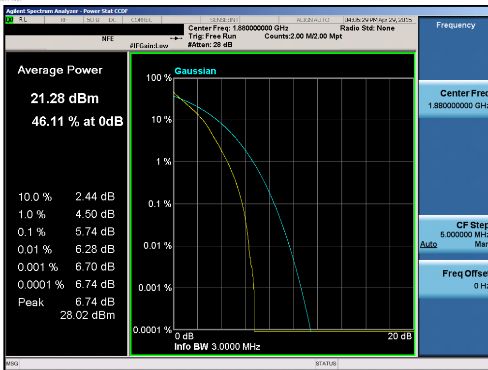
Plot 6-145. PAR Plot (Band 2 – 3.0MHz QPSK – RB Size 15)
