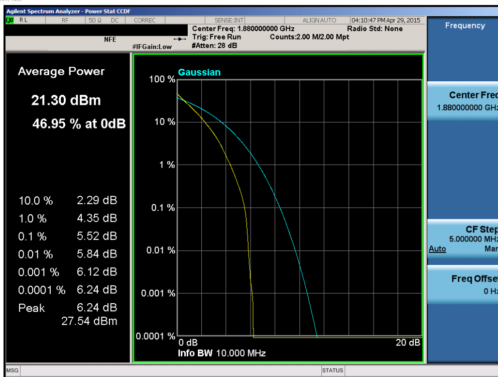
Plot 6-149. PAR Plot (Band 2 – 10.0MHz QPSK – RB Size 50)
